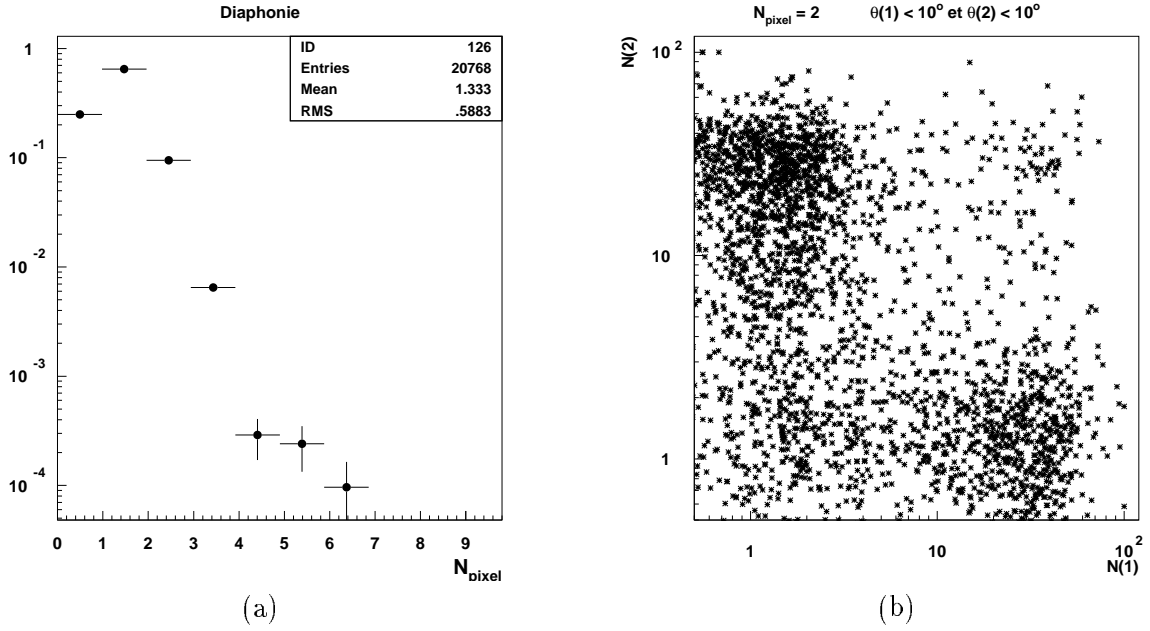
FIG. 5.4: (a) Distribution expérimentale du nombre de pixels touchés au voisinage immédiat de la trajectoire dans le cas de trajectoires ne passant pas par le radiateur. (b) Nombre de photoélectrons détectés sur l'imageur dans le cas d'une multiplicité de 2 et d'un angle \theta_c reconstruit inférieur à 10^\circ pour les 2 pixels.
