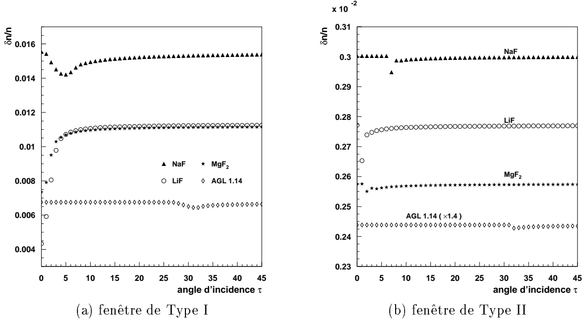
FIG. 3.10: Contribution de la dispersion optique à l'incertitude sur la mesure de la vitesse \beta en fonction de l'angle d'incidence \tau de la particule, pour des radiateurs en \text{NaF} , \text{LiF} et \text{MgF}_2 d'un cm d'épaisseur. (a) Photocathode en Bialkali B + fenêtre en silice fondue (Type I). (b) Photocathode en bialkali B + fenêtre en verre sodocalcique (Type II).
