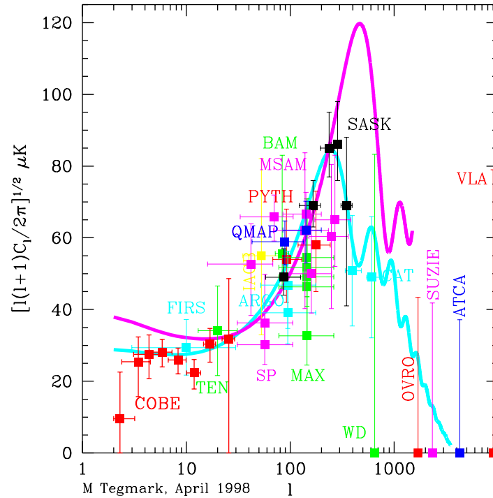
FIG. 1.2: Résumé des mesures des anisotropies du rayonnement à "3 K" (CMB) [5]. Les anisotropies sont développées en harmoniques sphériques : \delta T(\theta, \phi) = \sum a_{lm} Y_{lm} S(\theta, \phi) , avec C_l = \langle |a_{lm}|^2 \rangle . Cette figure montre la variation de la température entre deux lignes de visée séparées d'un angle \theta , avec l = \frac{200^\circ}{\theta} . Les courbes sont des prédictions des modèles de CDM (matière noire froide, non baryonique) avec \Omega_0 = 1 (courbe claire) et \Omega_0 = 0.3 (courbe foncée). L'ajustement est meilleur pour la première courbe et est compatible avec l'existence de pics acoustiques, qui signalent le découplage de la matière et du rayonnement dans l'univers jeune.
