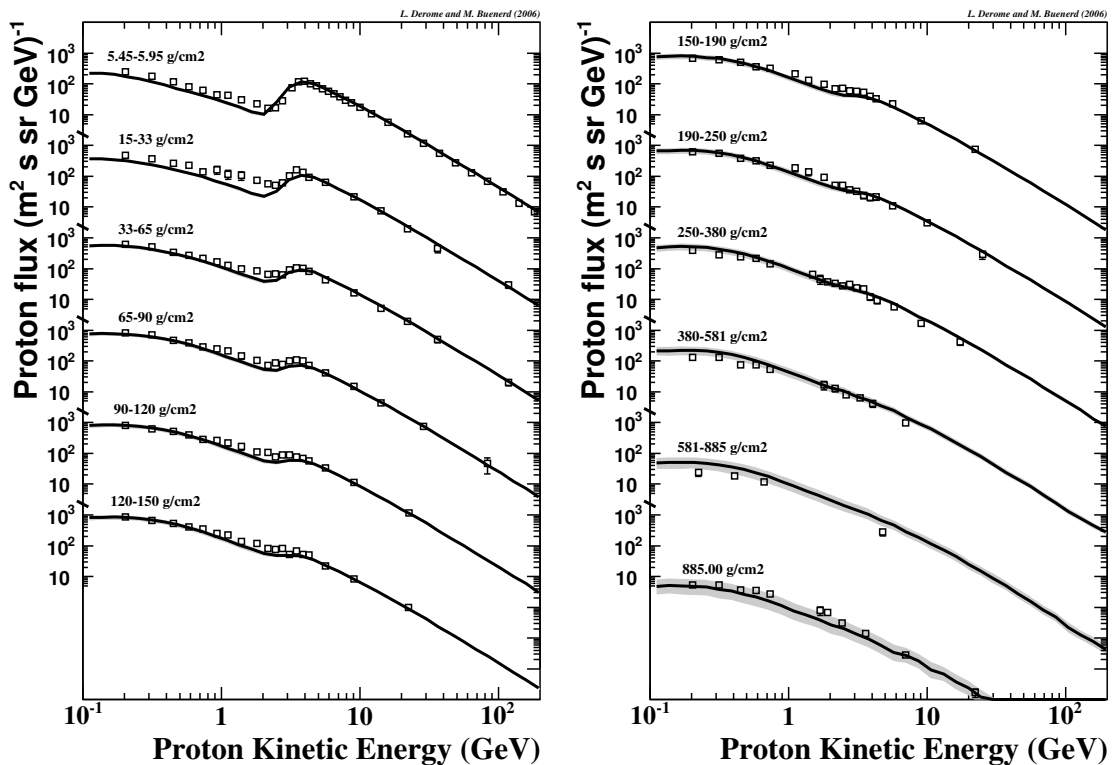
FIG. 1.25 – Symboles : Flux de protons mesurés par l’expérience CAPRICE pour différentes altitudes lors du vol effectué en 1998 depuis Fort Sumner, New Mexico [95] comparés au résultat de la simulation. La zone gris clair correspond à l’intervalle de confiance à 95 % estimé à partir de la simulation (seule l’erreur venant des sections efficaces de production est considérée).
