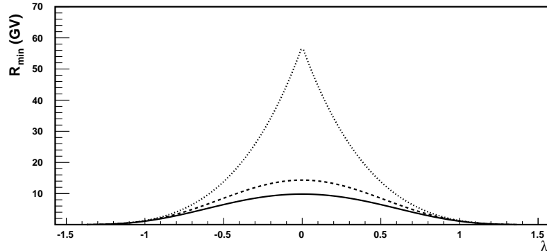
FIG. 1.4 – Evolution de la coupure géomagnétique en rigidité R en fonction de la latitude \lambda pour une particule chargée positivement ( \xi = 1 ) et pour plusieurs angles est-ouest. \eta = \frac{\pi}{2} : trait plein, \eta = 0 : trait tireté, \eta = -\frac{\pi}{2} : trait pointillé.
