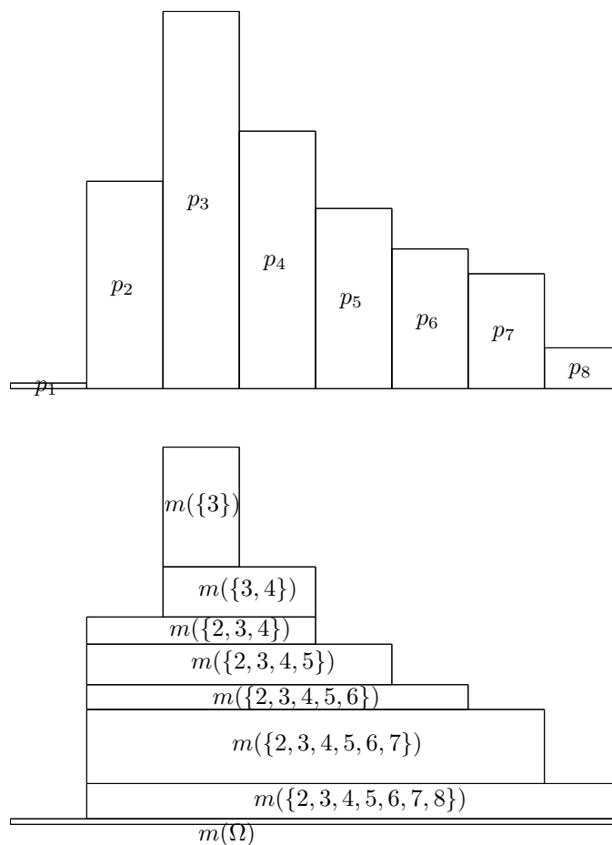
FIG. 7.1 – Correspondance entre, en haut, une distribution de probabilité p représentée par la surface des rectangles et, en bas, une fonction de croyance dont la distribution m est représentée par la surface des tranches successives. Par construction les ensembles focaux sont emboîtés, c'est à dire que la fonction de croyance est consonnante, c'est une mesure de possibilité. Source des données : opinion de l'expert 1 dans le chapitre 9.
