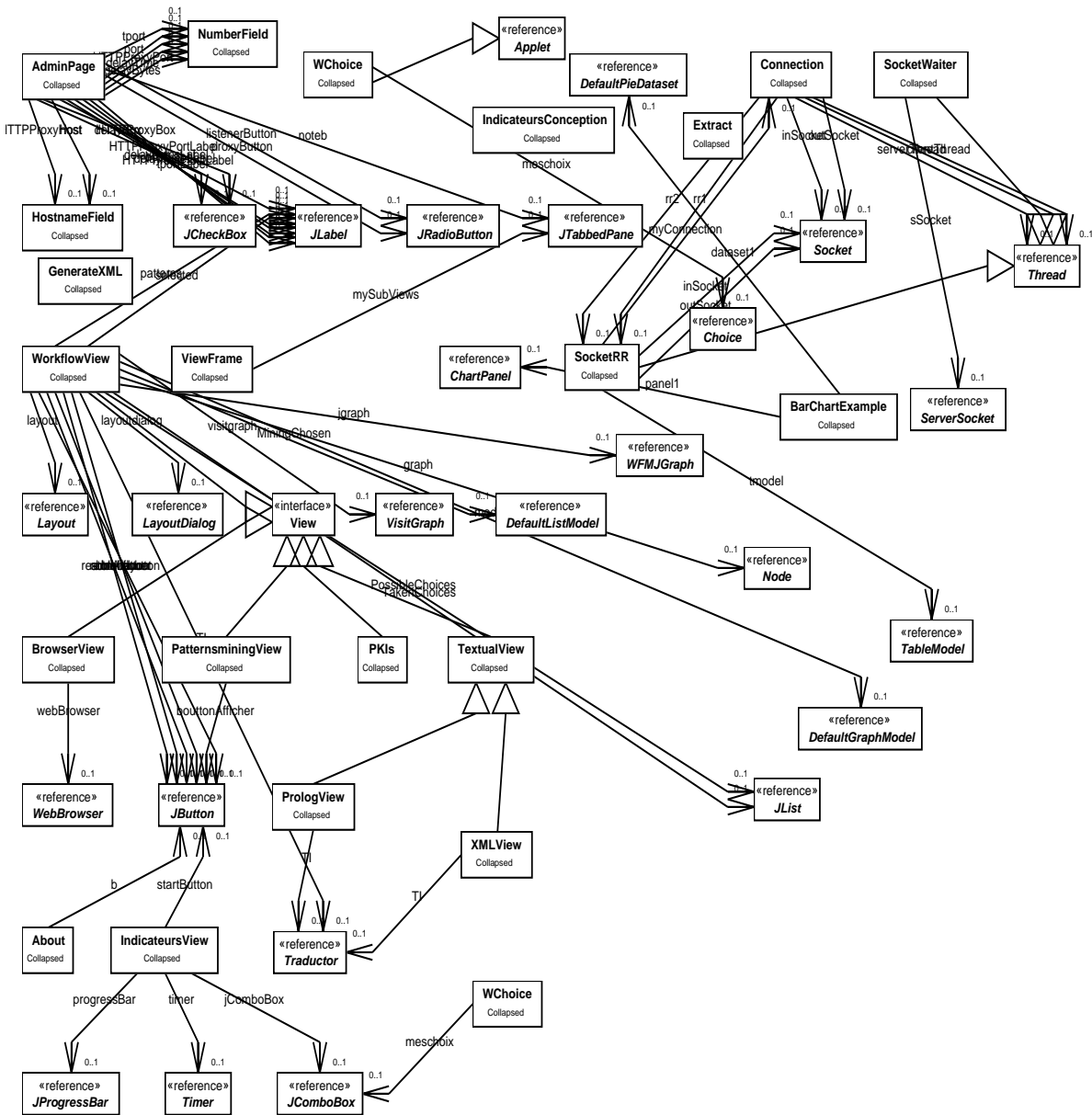
Figure C.8 Diagramme de classes de l'architecture générale de Workflowminer
