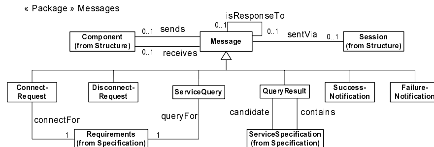
FIG. 3.3 – Module pour la partie messages du modèle statique, Baresi et al. (2003).
