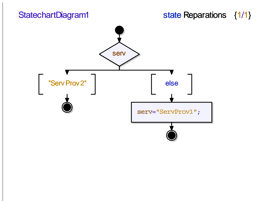
FIG. B.6 – Diagramme de machine à état de l'intercepteur Concrete Service Invoquer (2/2).
