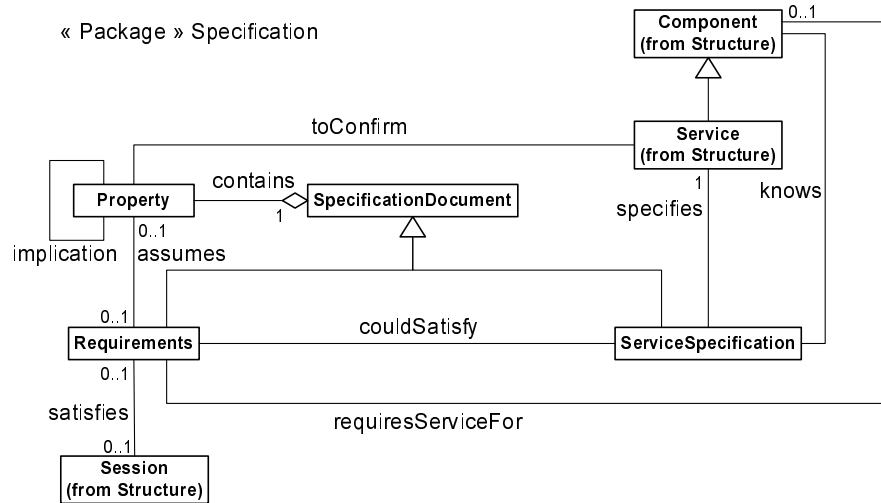
FIG. 3.2 – Module pour la partie spécification de documents du modèle statique, Baresi et al. (2003).
