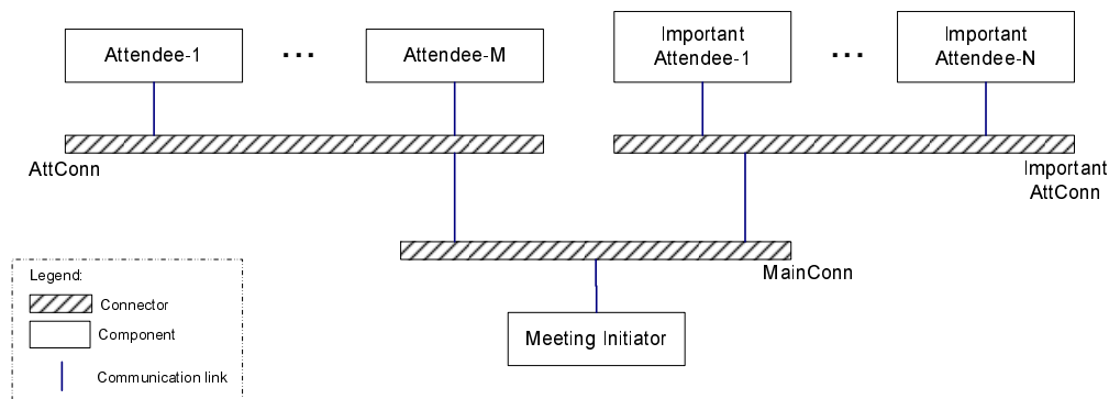
FIG. 2.4 – Style d'architecture C2 pour un système de gestion de réunions, Taylor et al. (1996) .
