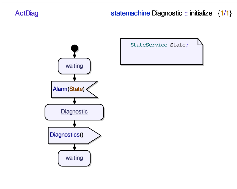
FIG. B.11 – Diagramme de machine à état du composant Diagnostic .
