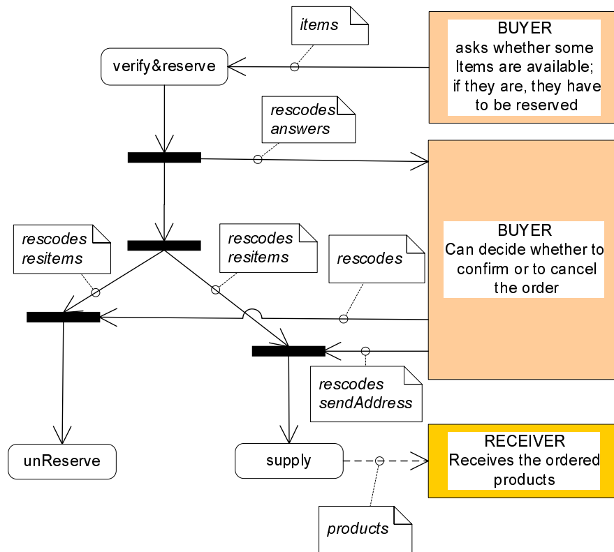
FIG. 5.28 – Workflow du fournisseur dans l'application « Foodshopping ».
