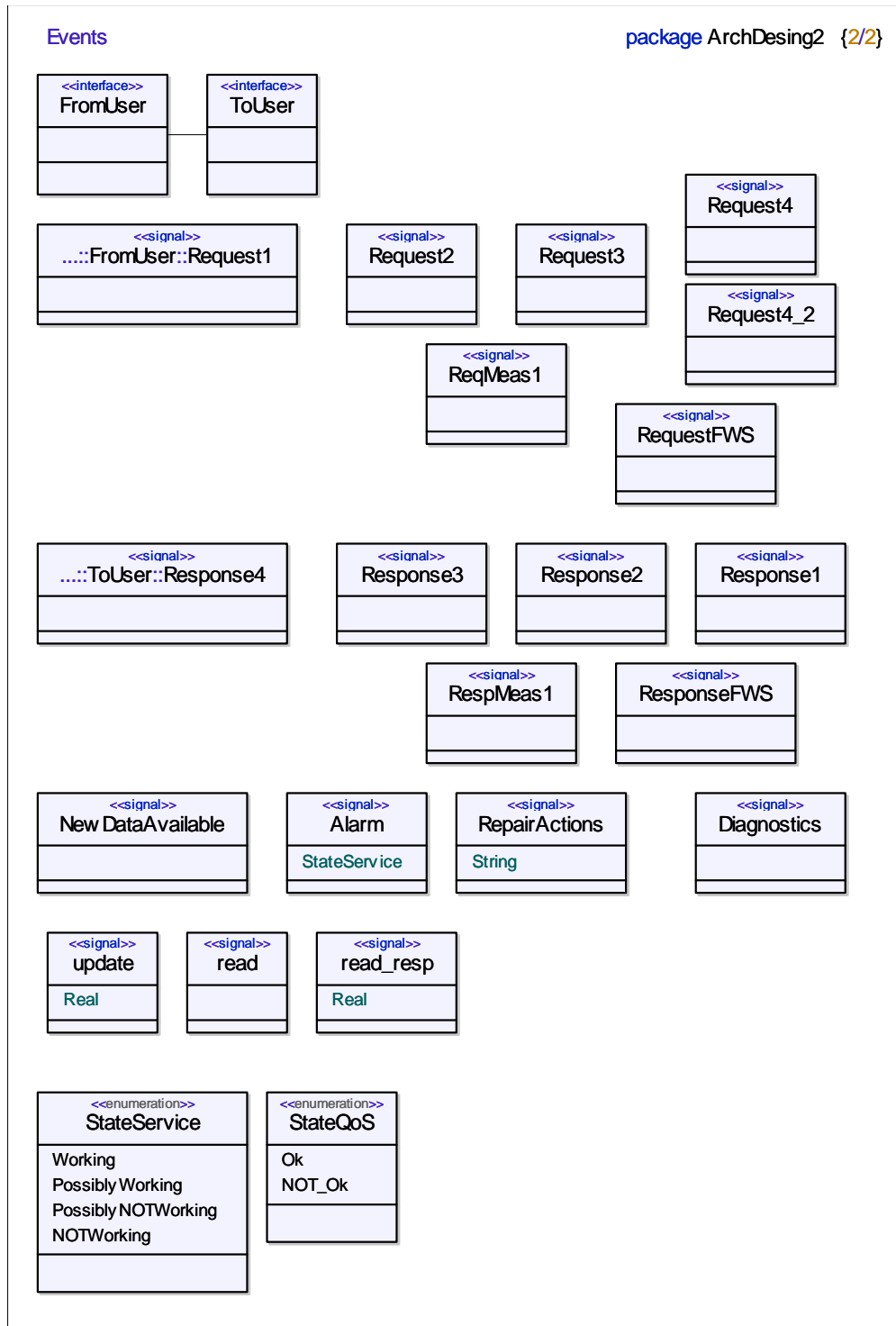
FIG. B.1 – Messages échangés pour les composants de l'architecture de gestion de la QoS.
