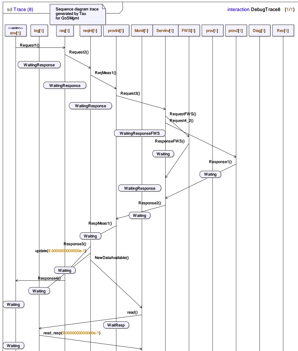
FIG. 6.28 – Simulation de l'architecture de gestion de la QoS (3/3).
