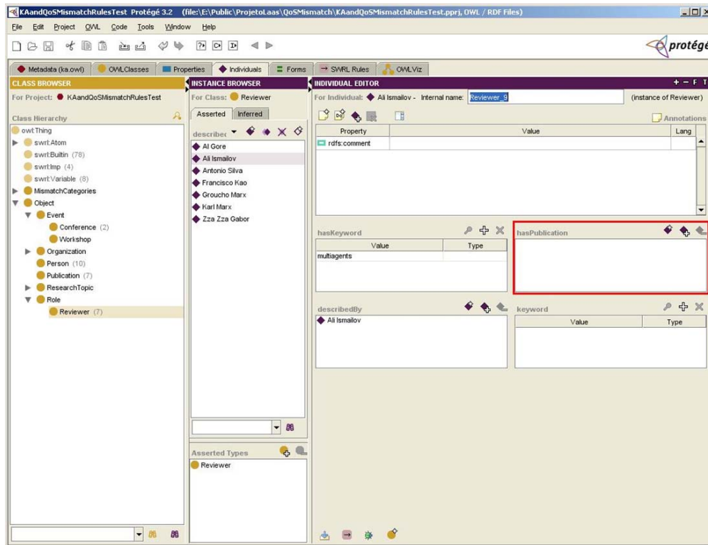
FIG. 6.10 – Instances de la classe Reviewer .
