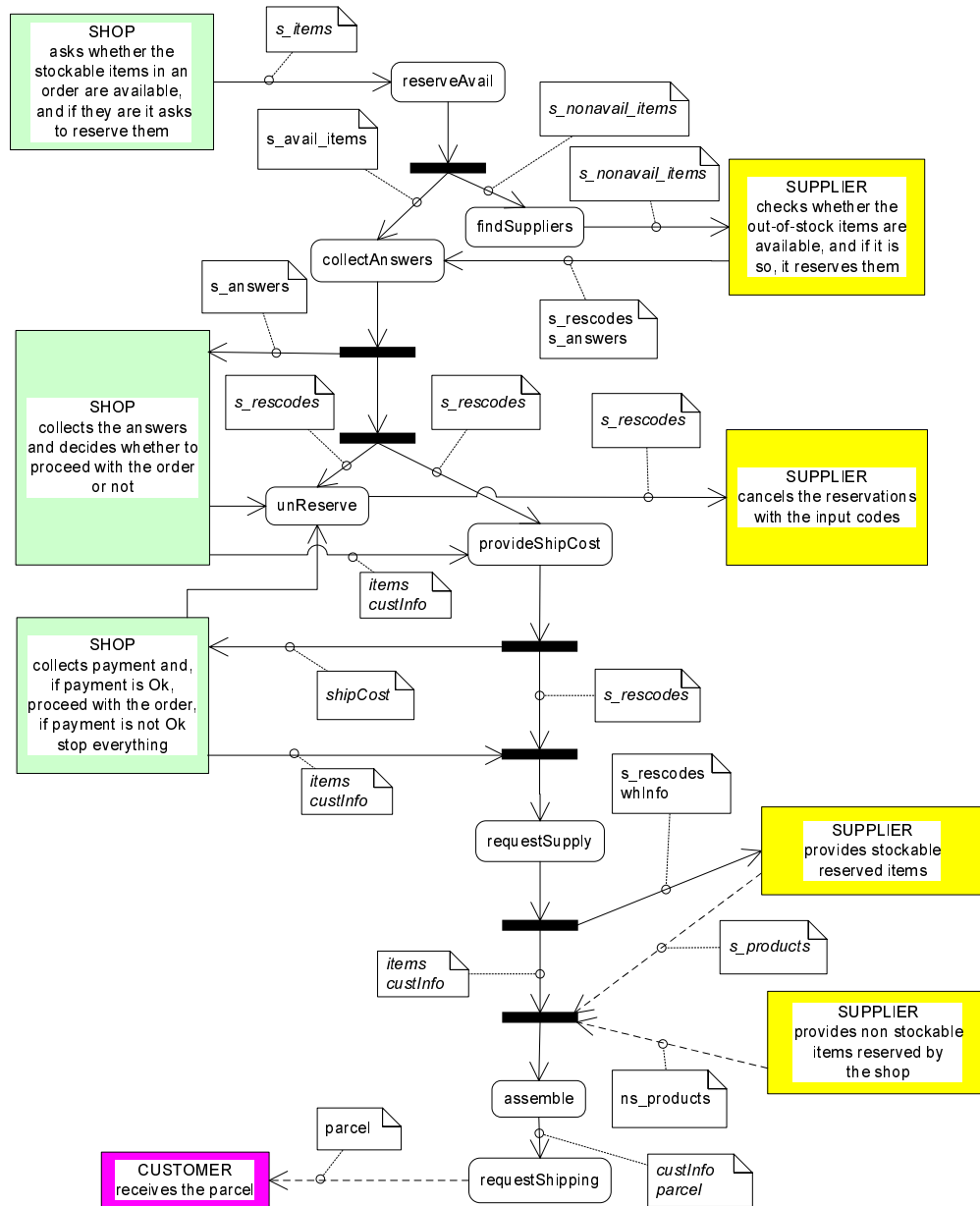
FIG. 5.27 – Workflow de l'entrepôt dans l'application « Foodshopping ».
