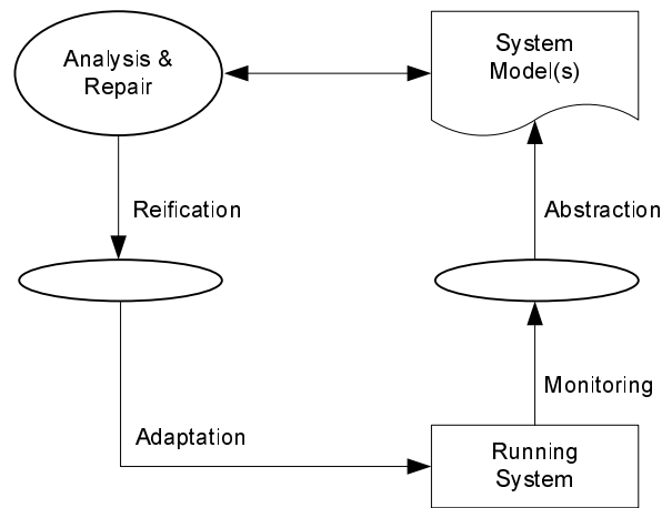
FIG. 3.5 – Modèle abstrait pour l'adaptation des architectures, Garlan et Schmerl (2002) .
