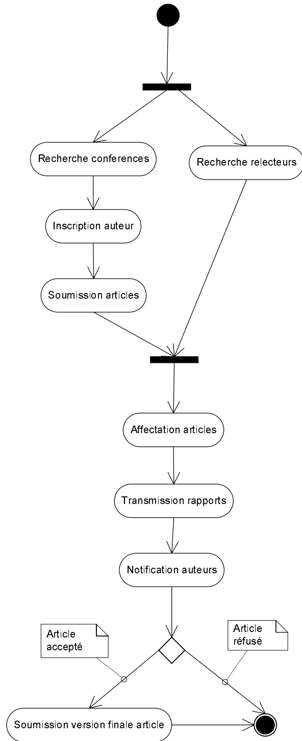
FIG. 5.9 – Relations de dépendances entre phases.
