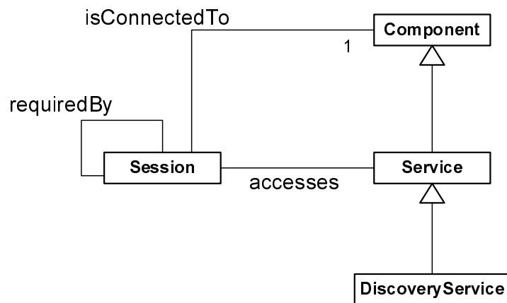
FIG. 3.1 – Module pour la partie structurelle du modèle statique, Baresi et al. (2003).
