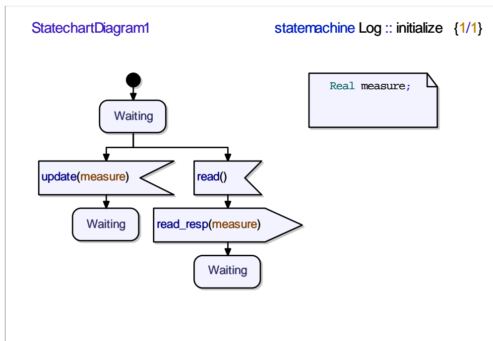
FIG. B.8 – Diagramme de machine à état du composant Log .
