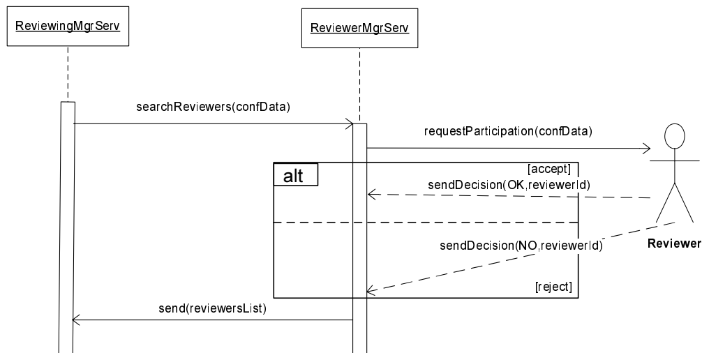
FIG. 5.2 – Recherche de relecteurs.
