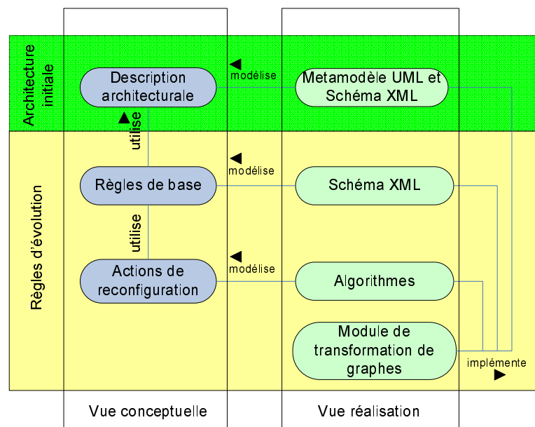
FIG. 4.1 – Stratégie générale pour le cadre logiciel.
