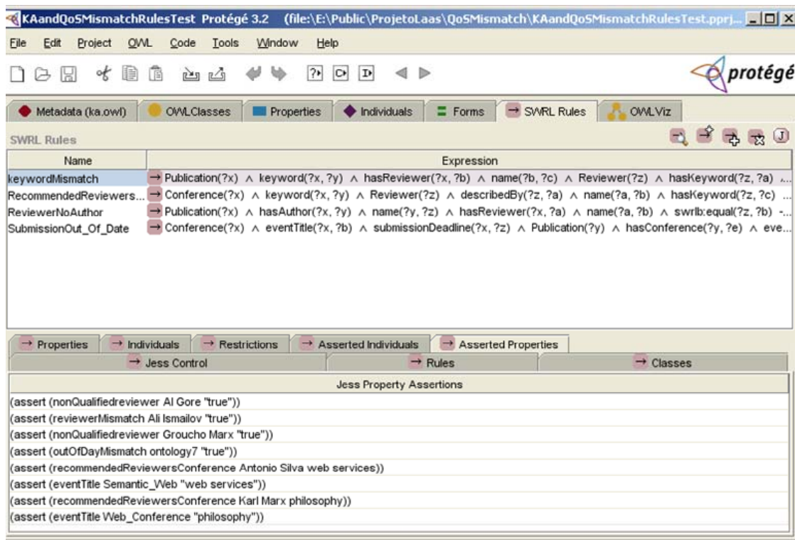
FIG. 6.15 – Exécution des règles avec Jess.
