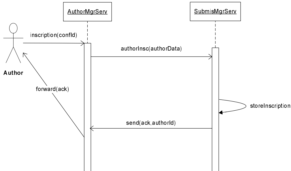
FIG. 5.3 – Inscription à une conférence.
