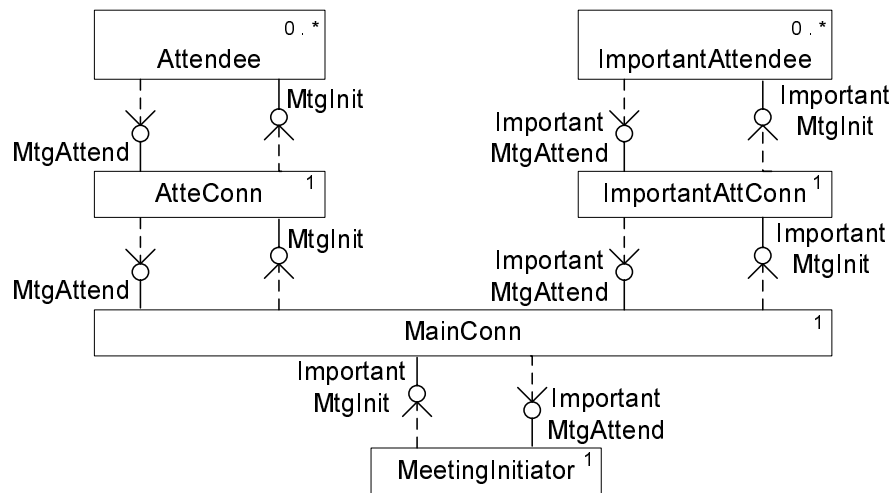
FIG. 2.8 – Utilisation des diagrammes de classes UML pour représenter une application de gestion de réunions selon le style C2.
