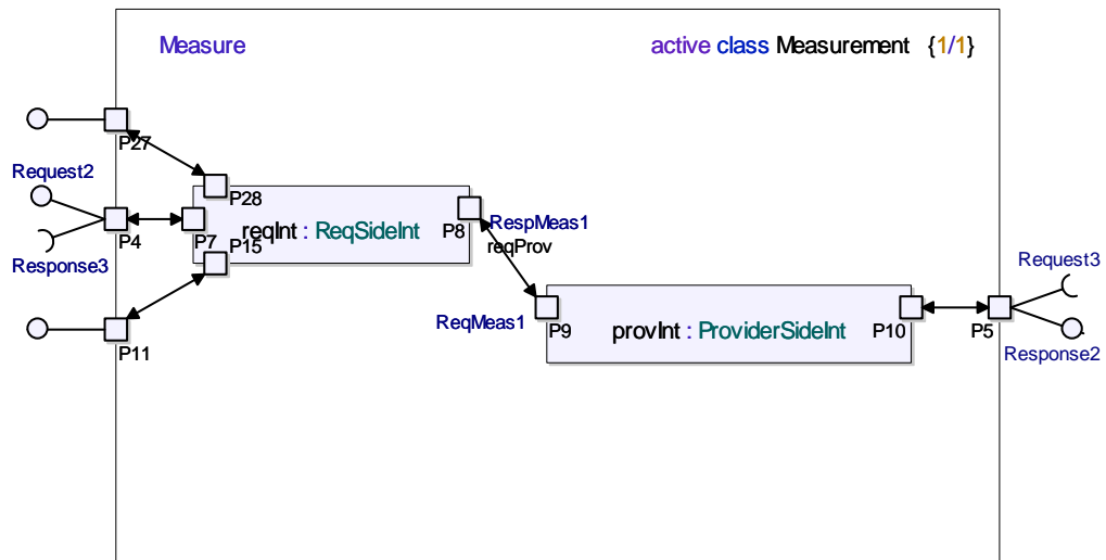
FIG. 6.23 – Diagramme de structures composites pour le module Measurement .
