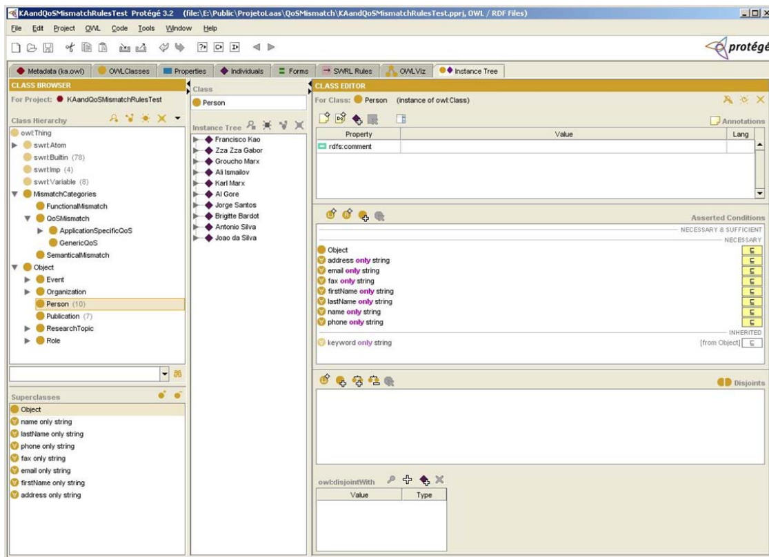
FIG. 6.5 – Propriétés de la classe Person .
