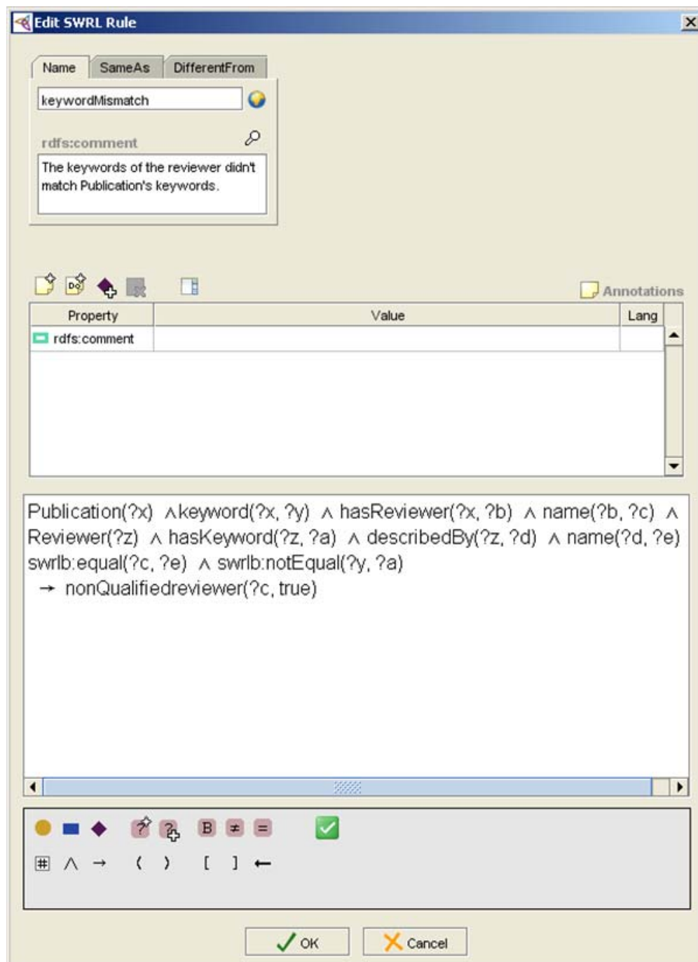
FIG. 6.11 – Dysfonctionnement dans l'affectation des papiers : relecteur dont le domaine de recherche et étranger au sujet du papier.
