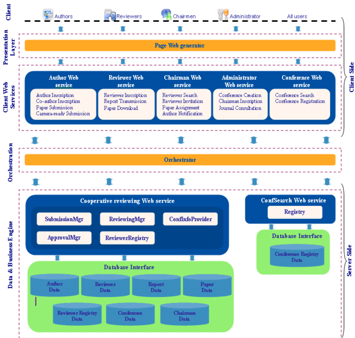
FIG. 5.18 – Architecture de mise en œuvre du système de gestion de conférences.
