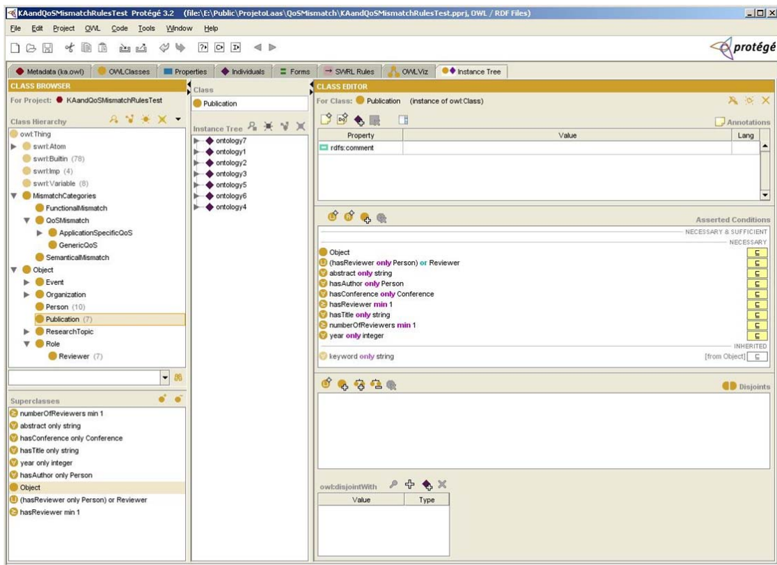
FIG. 6.4 – Propriétés de la classe Publication .
