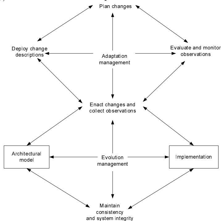
FIG. 3.7 – Une approche générique pour le logiciel auto-adaptatif, Oreizy et al. (1999).
