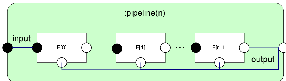
FIG. 2.2 – Architecture pipeline à base d'un composant composite dans Darwin.
