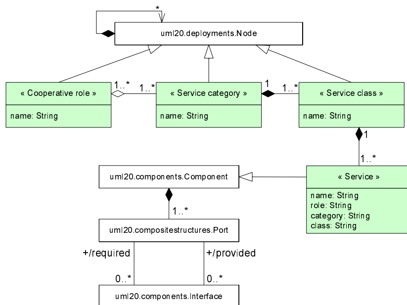
FIG. 4.2 – Un métamodèle étendant la vue de déploiement UML.
