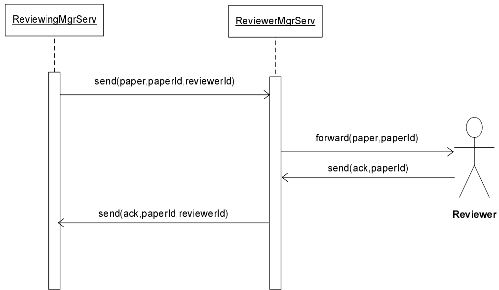
FIG. 5.5 – Affectation des articles.
