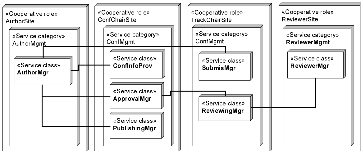
FIG. 5.10 – Architecture de déploiement du système de gestion de conférences.
