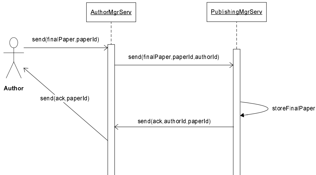
FIG. 5.8 – Soumission des articles pour édition.
