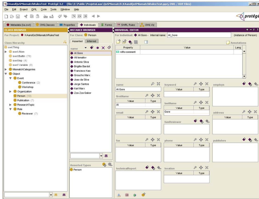
FIG. 6.9 – Instances de la classe Person .
