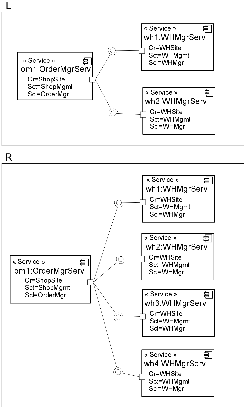
FIG. 5.31 – Application de la règle de duplication.
