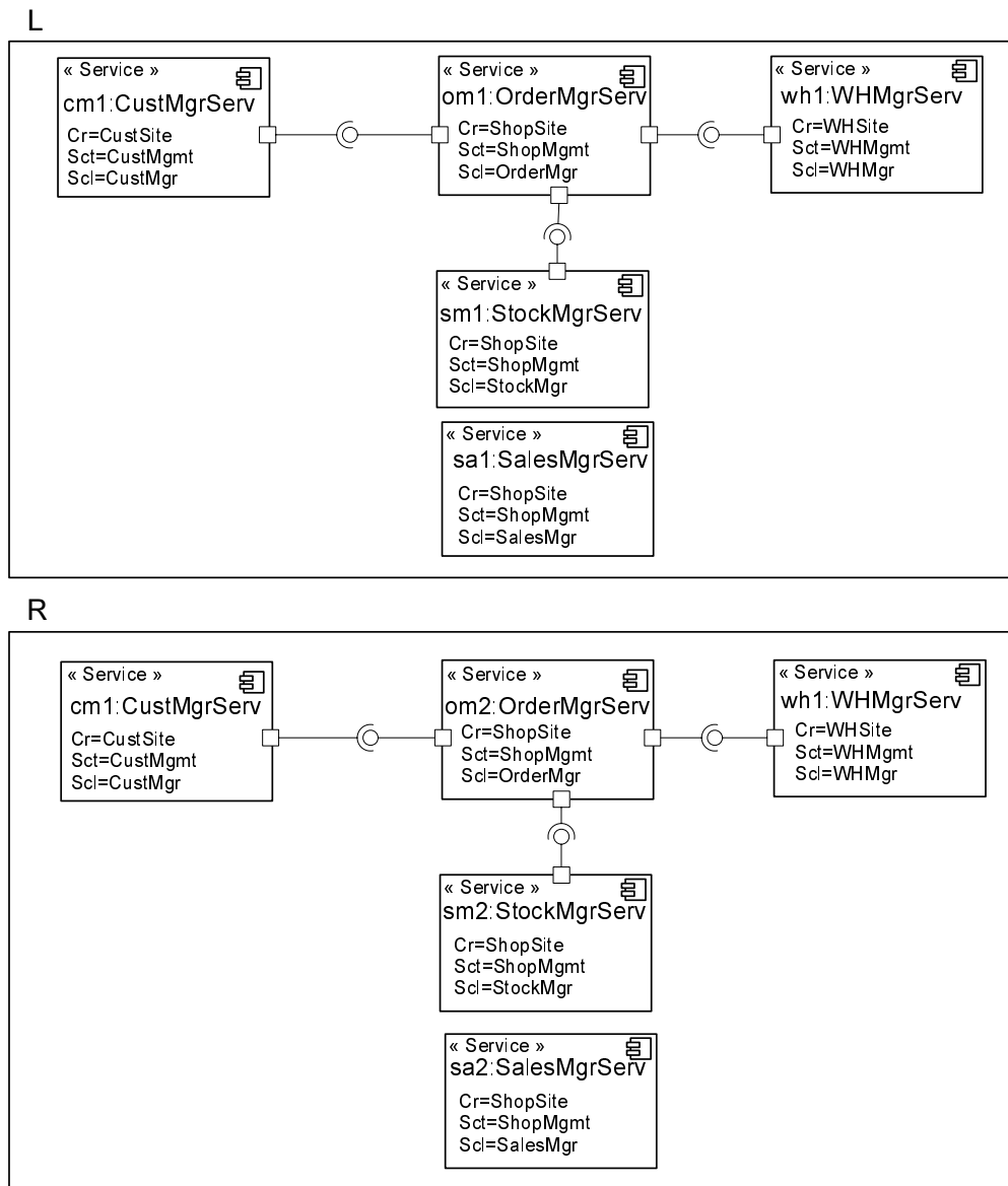
FIG. 5.34 – Application de la règle de substitution.
