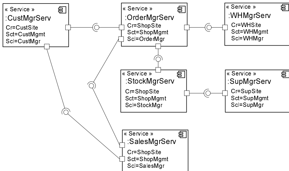
FIG. 5.30 – Interconnexion des services Web interagissant dans l'application « Foodshopping ».
