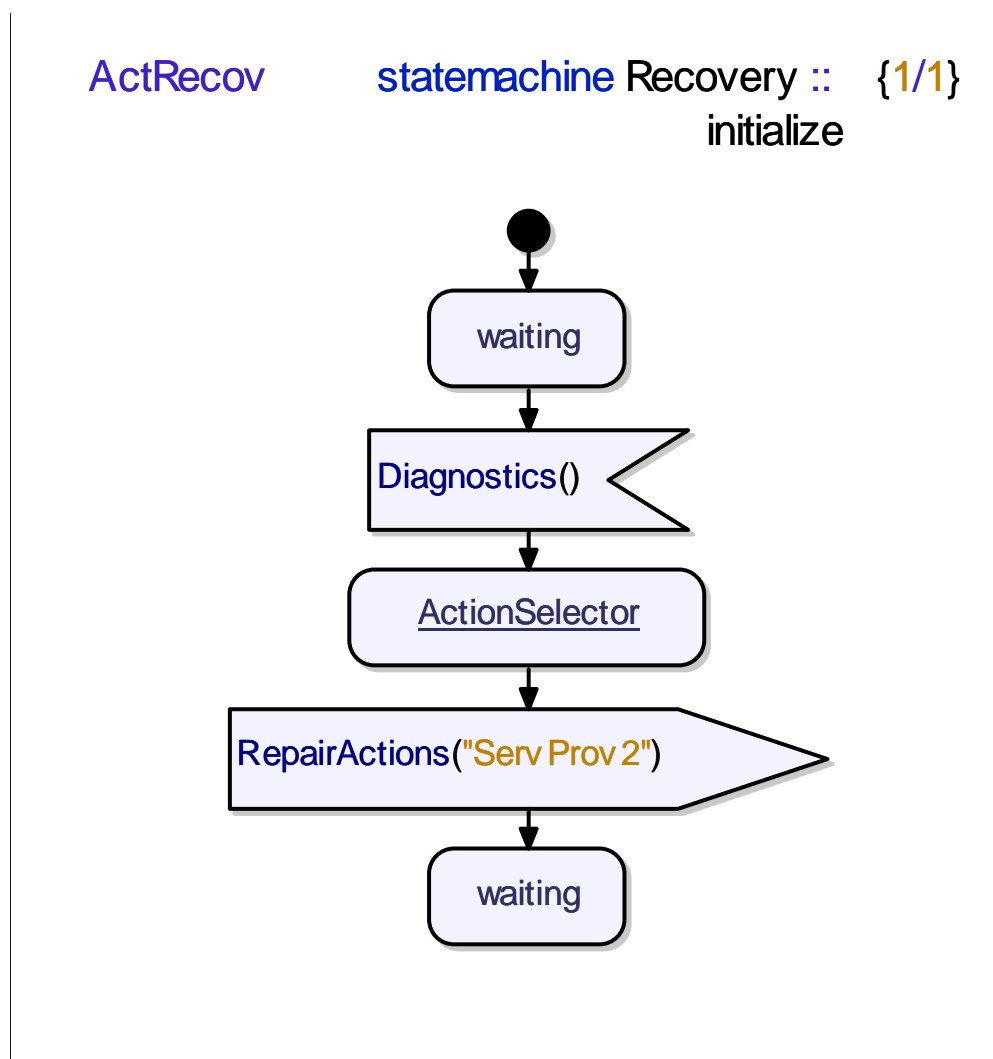
FIG. B.12 – Diagramme de machine à état du composant Recovery .
