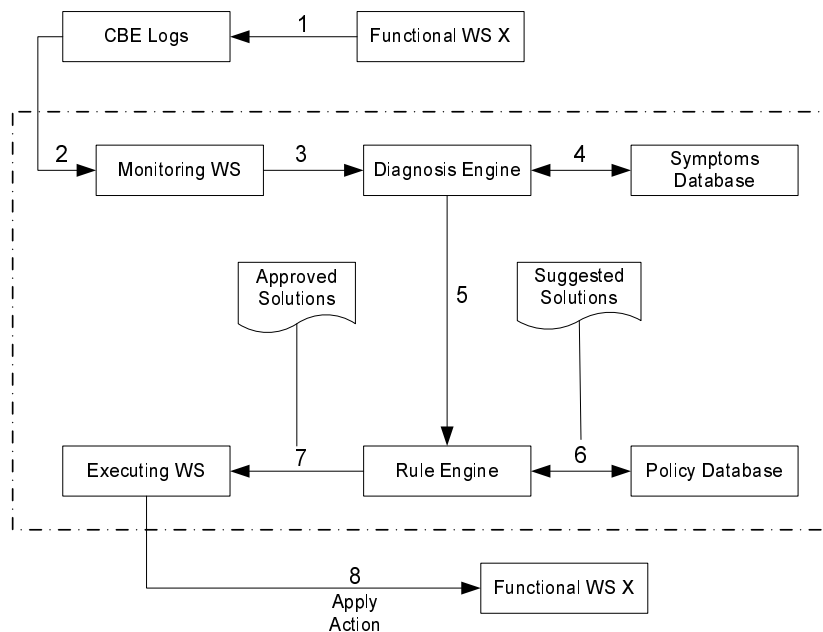
FIG. 3.12 – Implémentation de la stratégie MAPE pour le « self-healing » de services Web, Gurguis et Zeid (2005).
