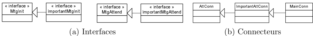
FIG. 2.7 – Modélisation UML des interfaces et des connecteurs d’une application de gestion de réunions.
