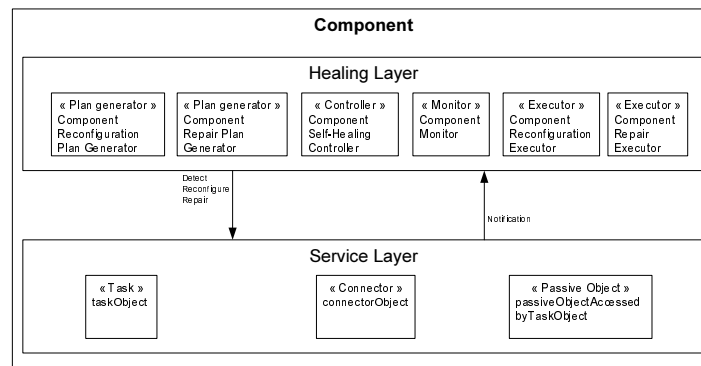
FIG. 3.8 – Architecture des composants « self-healing », Shin (2005).
