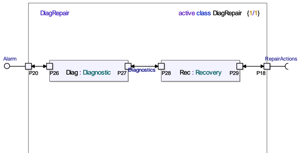
FIG. 6.24 – Diagramme de structure composite pour le module Diagnosis&Repair .
