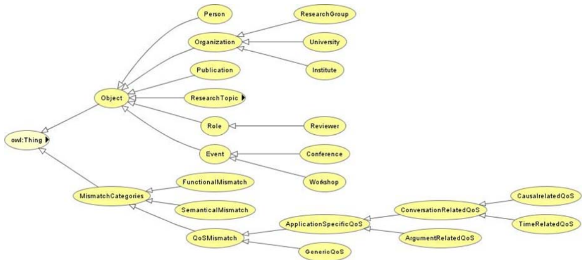
FIG. 6.2 – Ontologie caractérisant les cas de dysfonctionnements dans un système de gestion de conférences.
