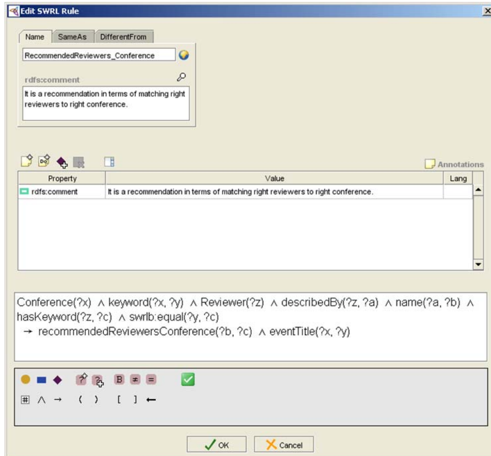
FIG. 6.14 – Recommandation de lecteurs en fonction des thèmes de la conférence.
