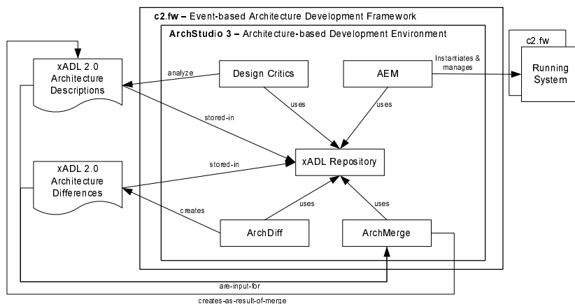
FIG. 3.9 – Outils et documents pour le développement de systèmes « self-healing », Dashofy et al. (2002).
