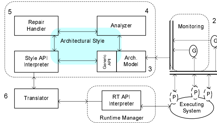
FIG. 3.6 – Infrastructure pour l'adaptation des systèmes, Garlan et Schmerl (2002) .
