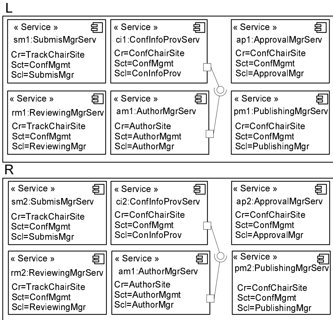
FIG. 5.14 – Application de la règle de substitution de services Web par le biais de la Catégorie de service .
