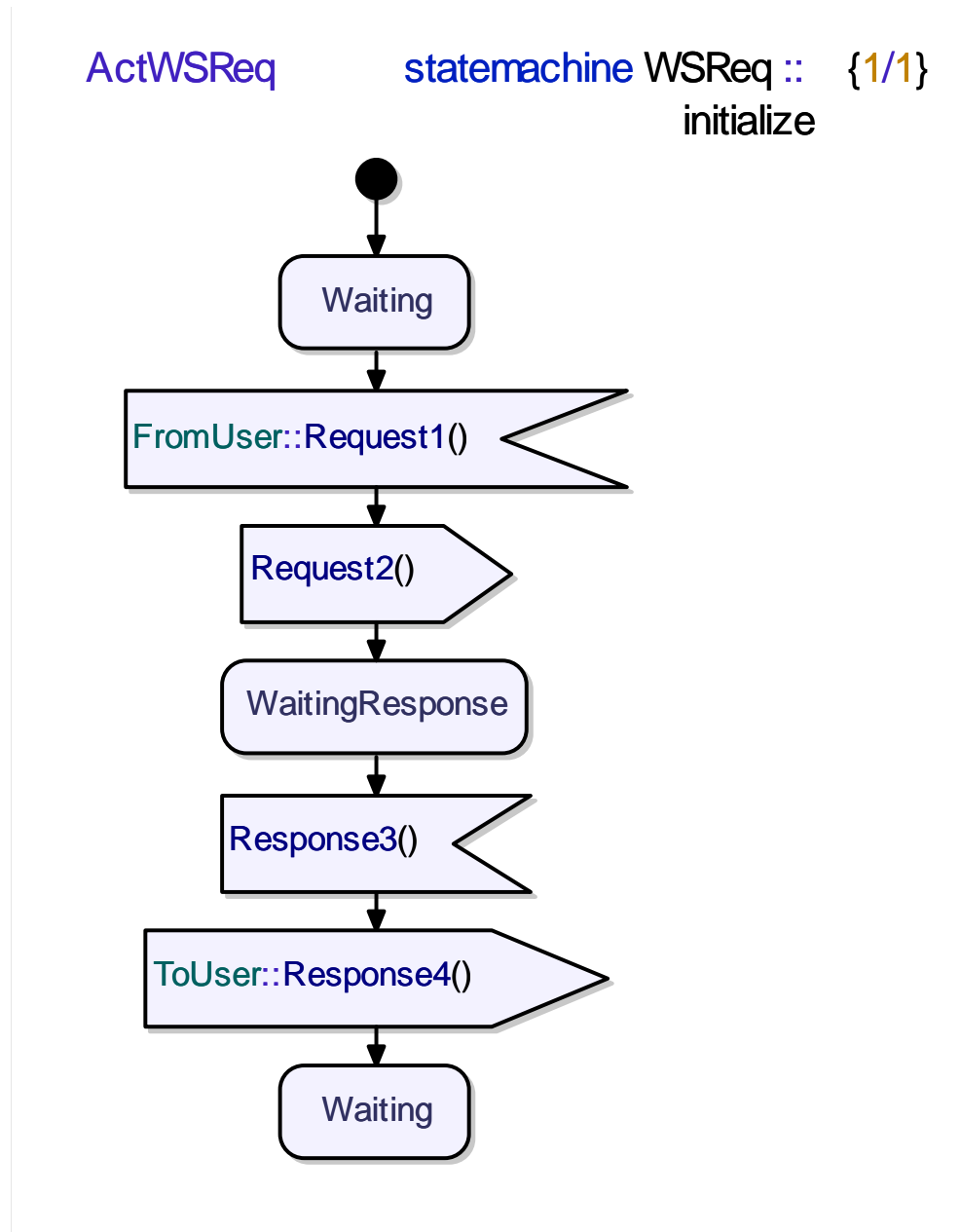
FIG. B.2 – Diagramme de machine à état du service Web demandeur.
