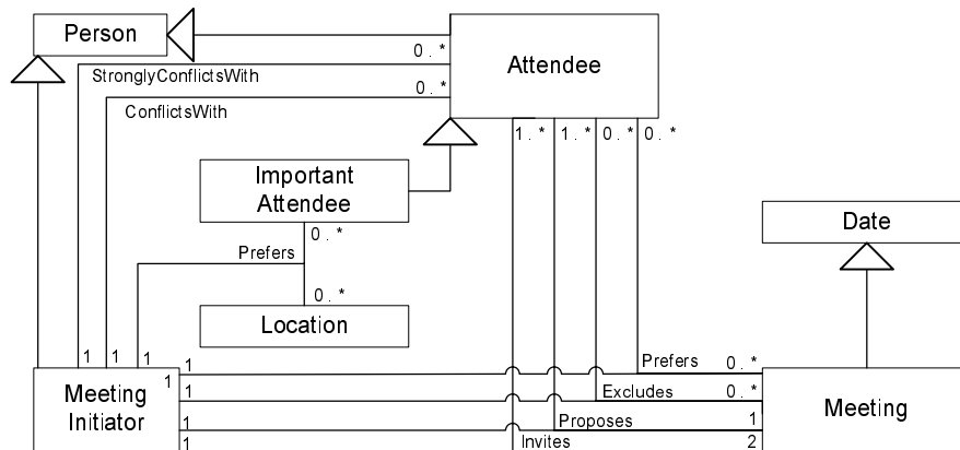
FIG. 2.6 – Modélisation d’une application de gestion de réunions par un diagramme de classe UML.
