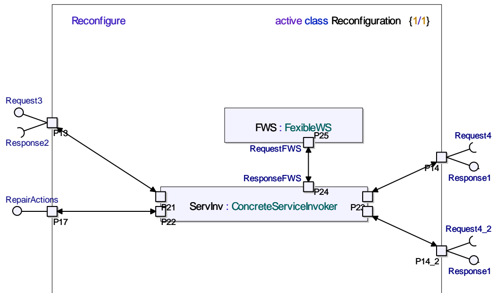
FIG. 6.25 – Diagramme de structure composite pour le module Reconfiguration .
