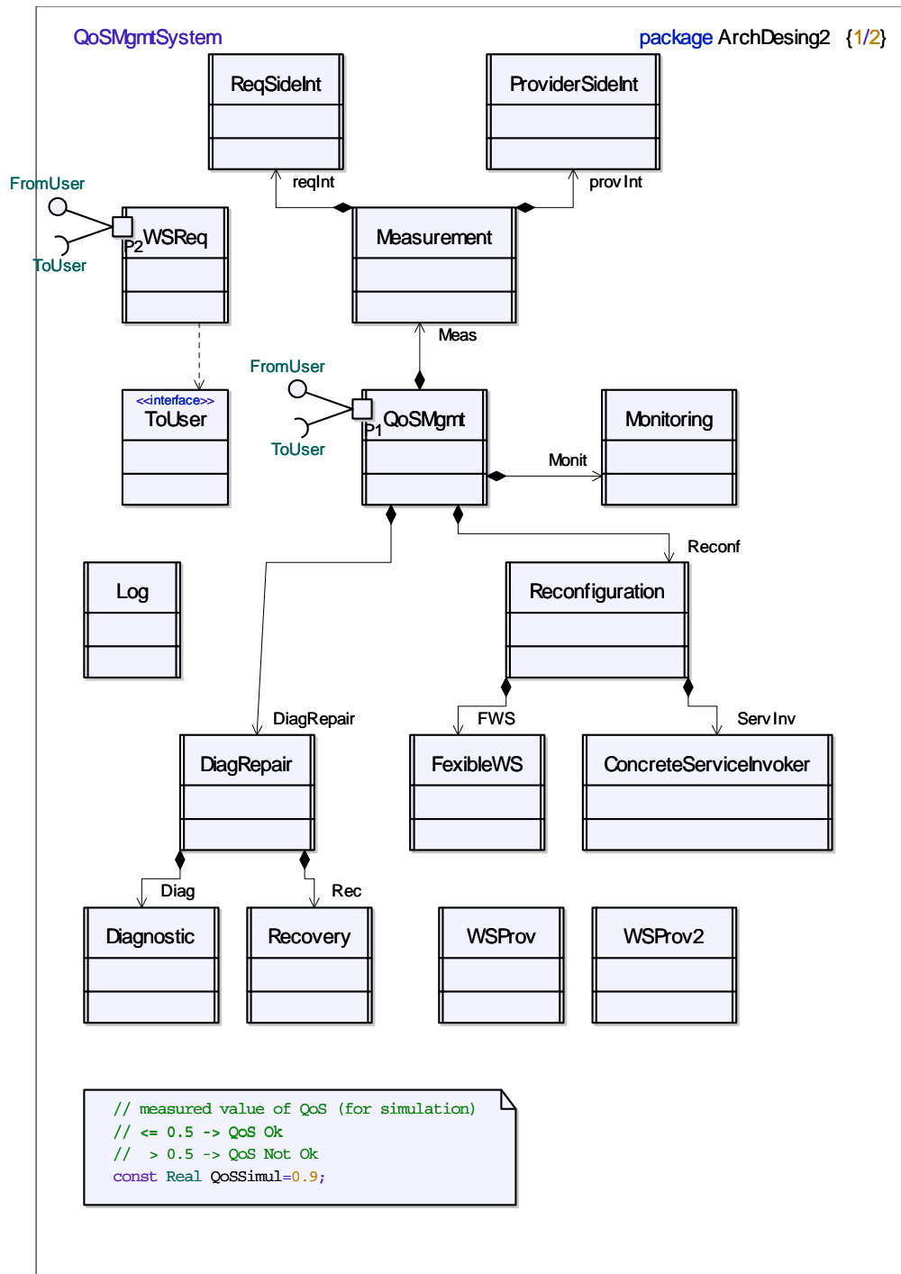
FIG. 6.21 – Diagramme de classes.
