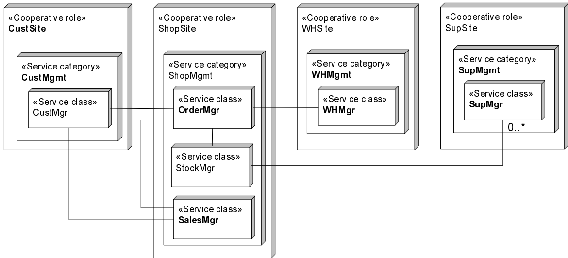
FIG. 5.29 – Architecture de déploiement de l'application « Foodshopping ».
