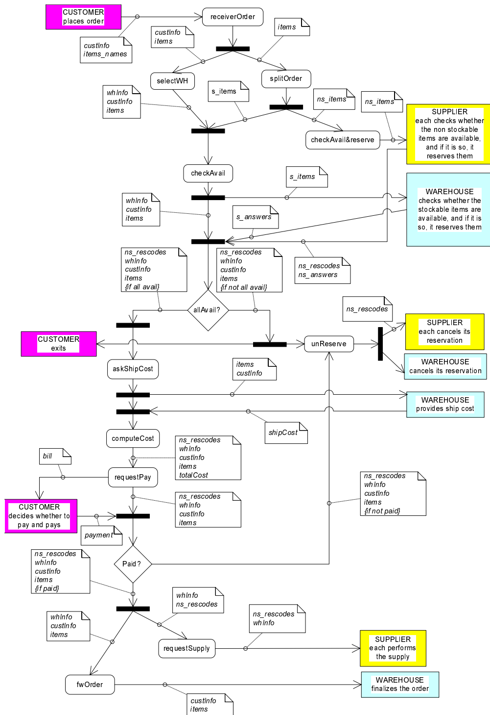
FIG. 5.26 – Workflow du magasin dans l'application « Foodshopping ».
