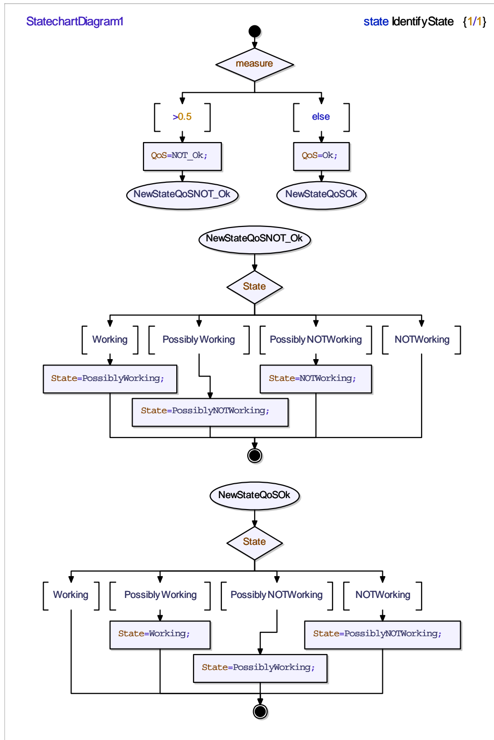
FIG. B.10 – Diagramme de machine à état du composant Monitoring (2/2).
