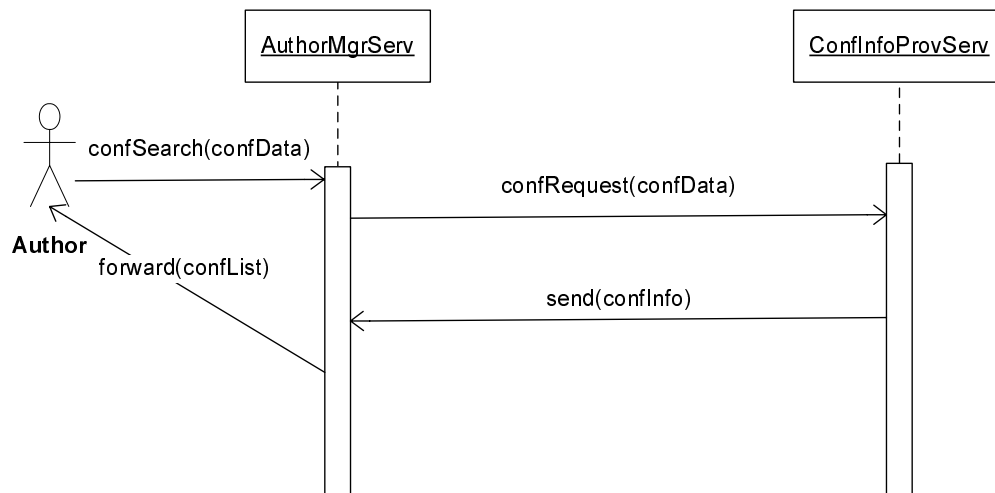
FIG. 5.1 – Recherche de conférences.
