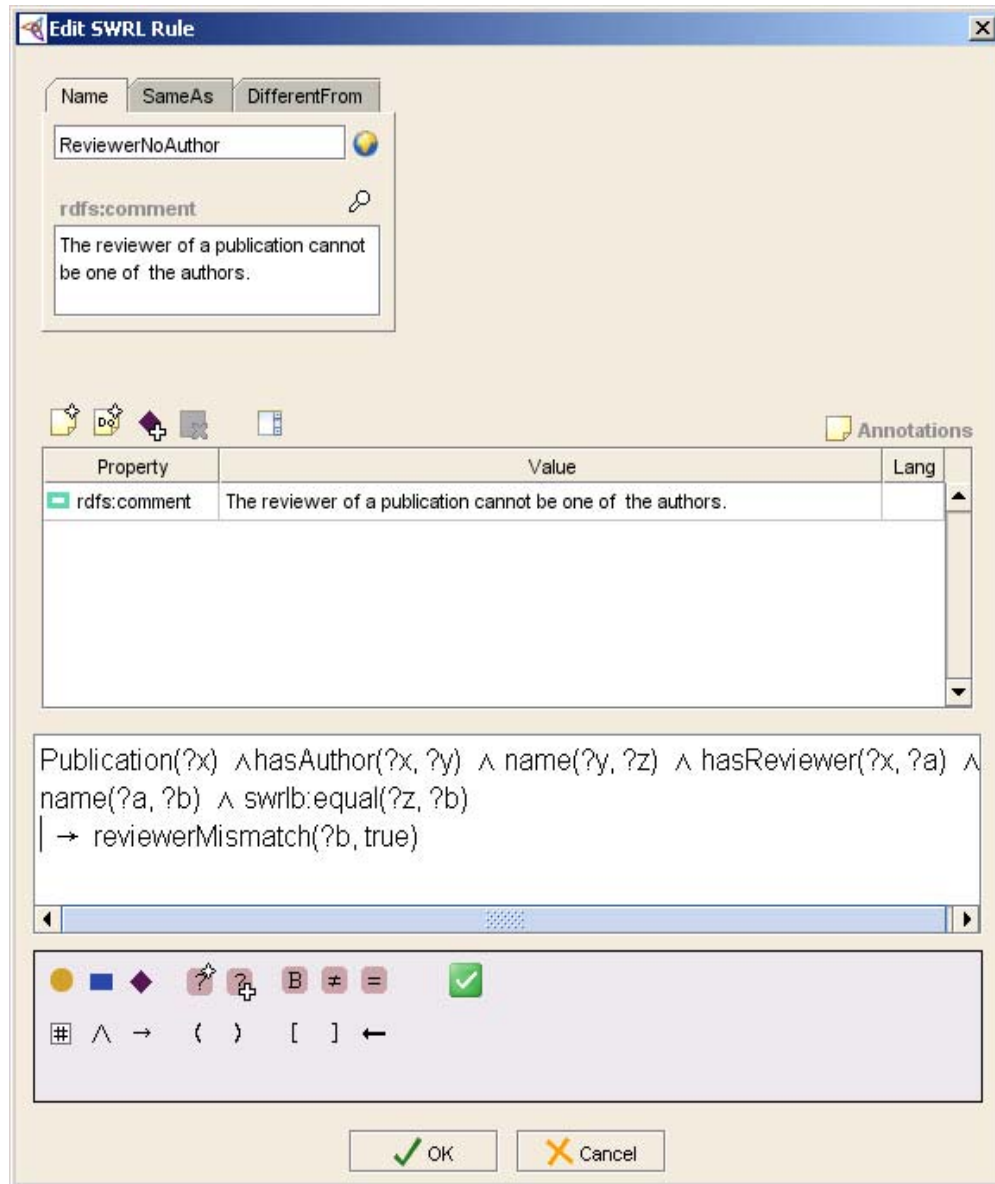
FIG. 6.12 – Dysfonctionnement dans l'affectation des papiers : Papier dont le lecteur et aussi auteur.
