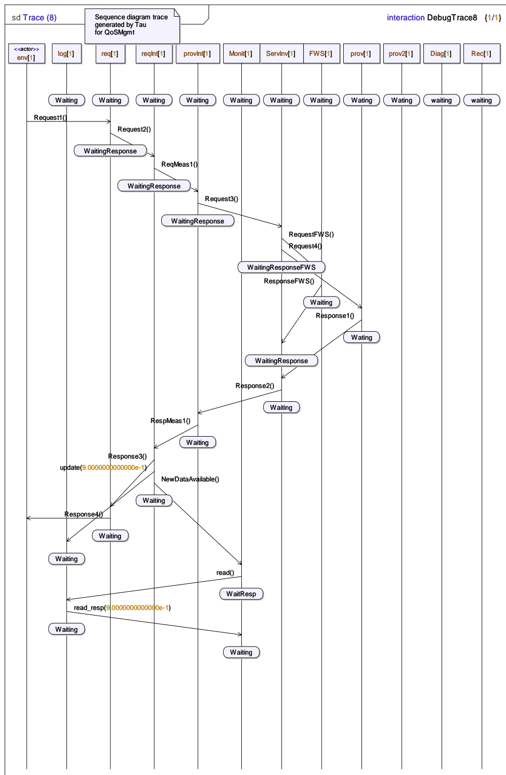
FIG. 6.26 – Simulation de l'architecture de gestion de la QoS (1/3).
