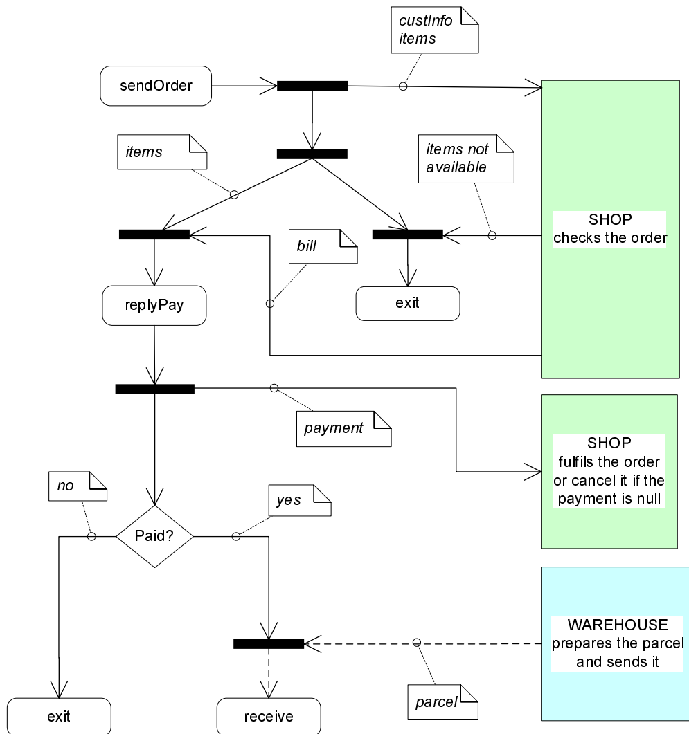
FIG. 5.25 – Workflow du client dans l'application « Foodshopping ».
