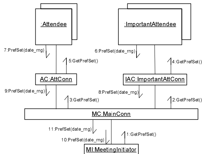
FIG. 2.9 – Utilisation des diagrammes de collaborations UML pour représenter une application de gestion de réunions selon le style C2.
