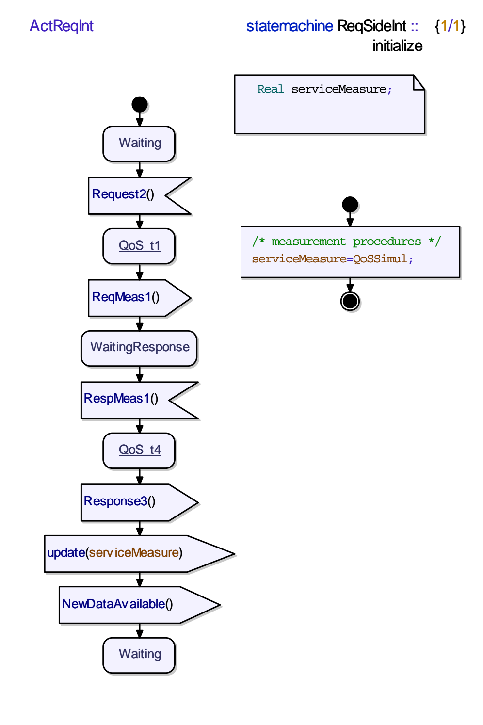
FIG. B.3 – Diagramme de machine à état de l'intercepteur du côté du WS demandeur.
