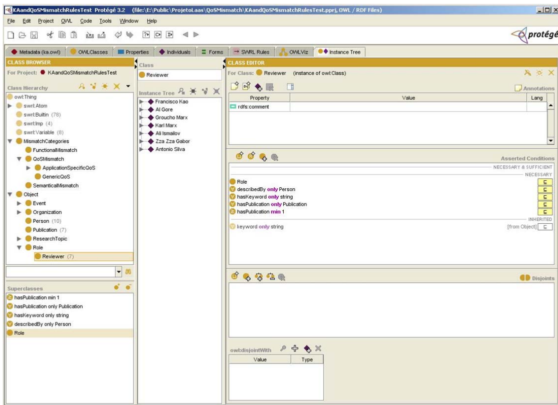
FIG. 6.6 – Propriétés de la classe Reviewer .
