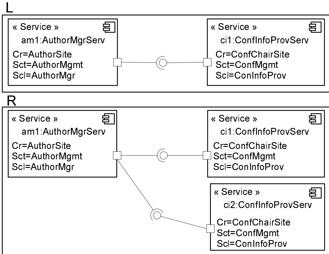
FIG. 5.11 – Application de la règle de duplication de services Web.
