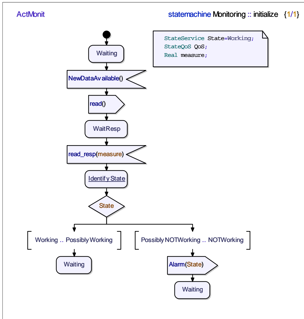
FIG. B.9 – Diagramme de machine à état du composant Monitoring (1/2).
