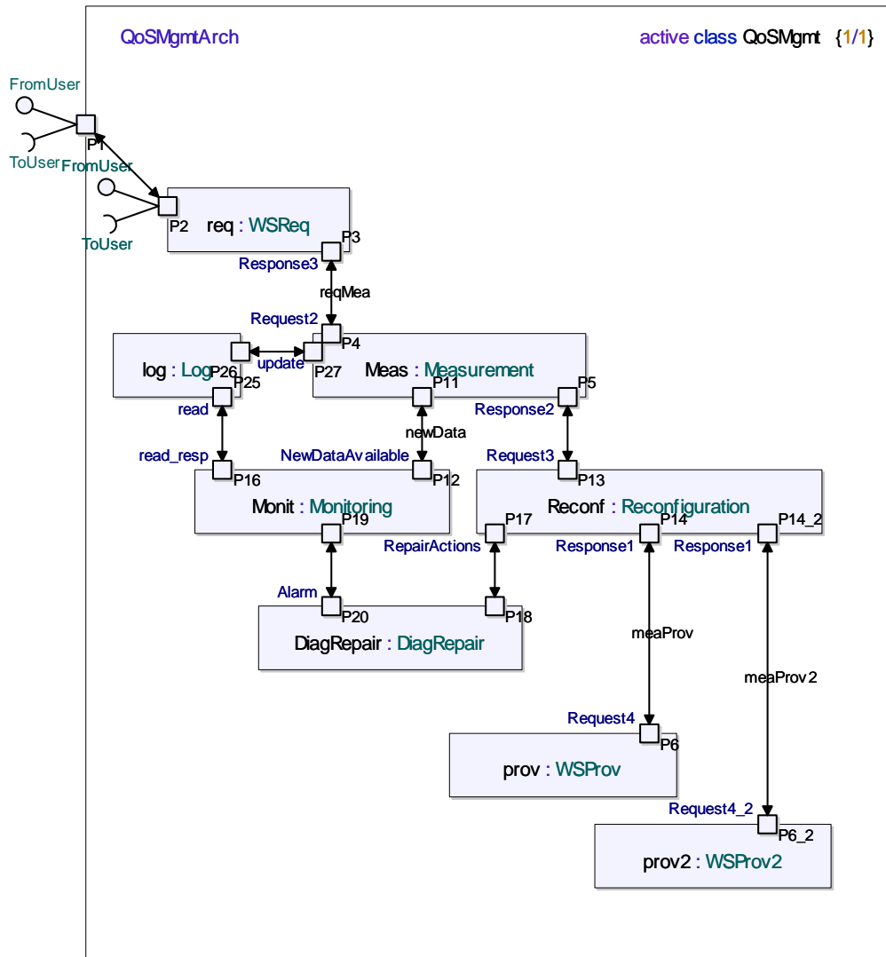
FIG. 6.22 – Diagramme de structure composite global.
