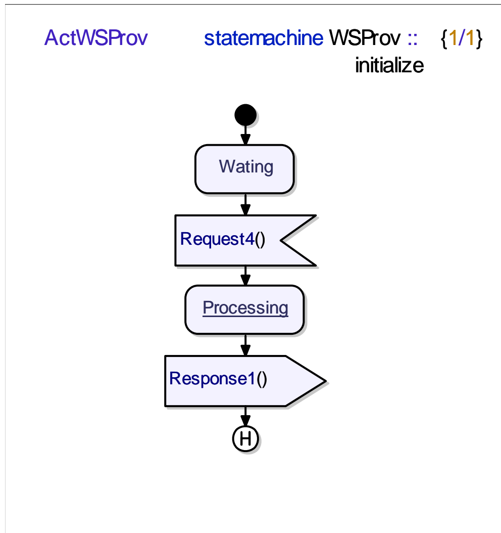
FIG. B.13 – Diagramme de machine à état du premier service Web fournisseur.
