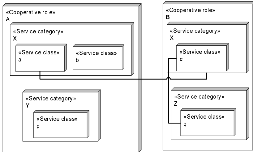
FIG. 4.3 – Description graphique d’une application de services Web modélisée par les notions de Rôle coopératif , Catégorie de service et Classe de service
