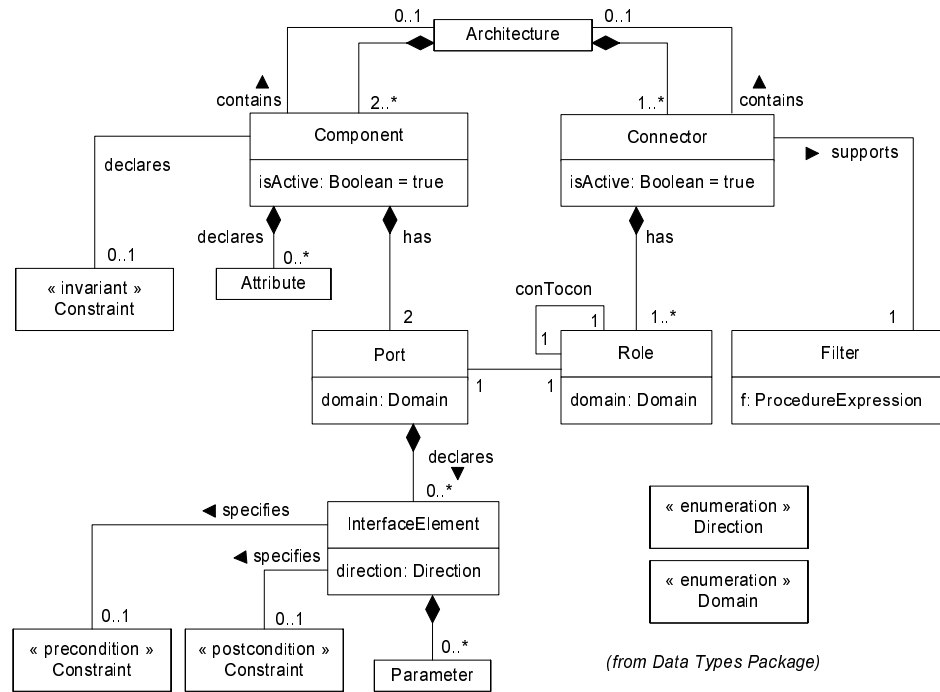
FIG. 2.10 – Syntaxe abstraite caractérisant le paquet C3.
