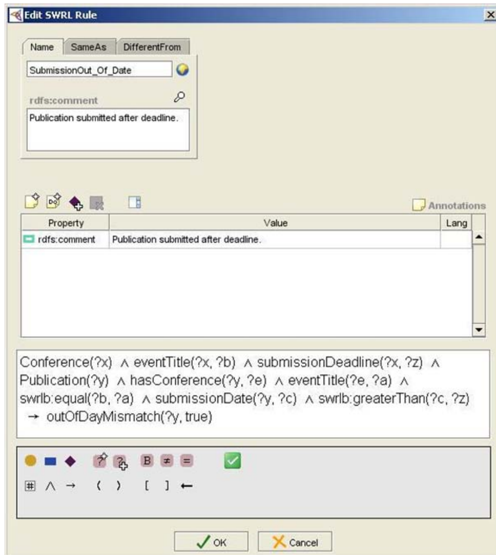
FIG. 6.13 – Dysfonctionnement dans la soumission des papiers : La date de soumission ne respect pas le « deadline ».
