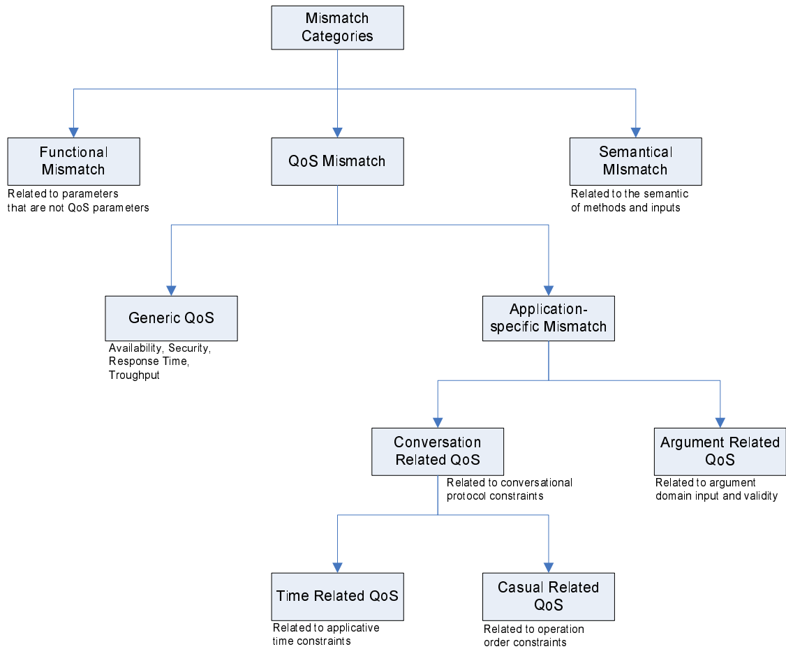
FIG. 6.1 – Classification générale des dysfonctionnements.
