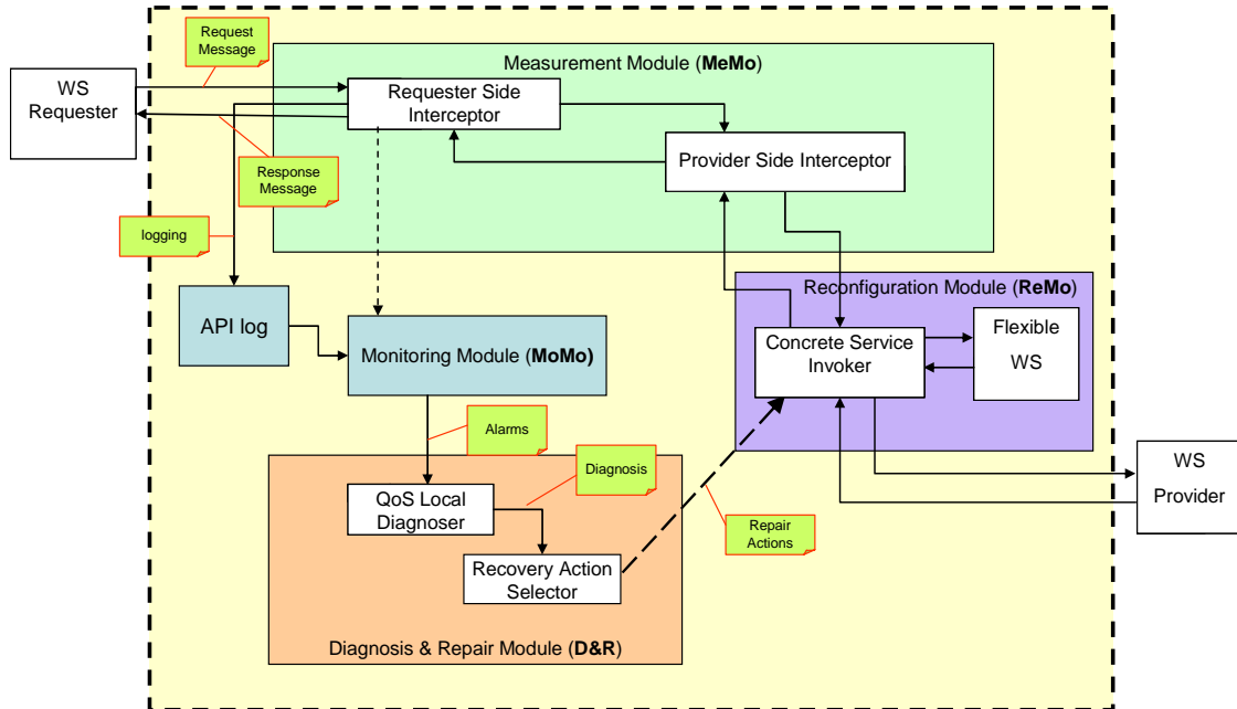
FIG. 6.20 – Architecture de gestion de la QoS.
