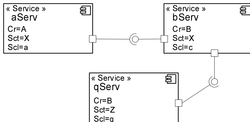
FIG. 4.4 – Description graphique des interactions entre services Web
