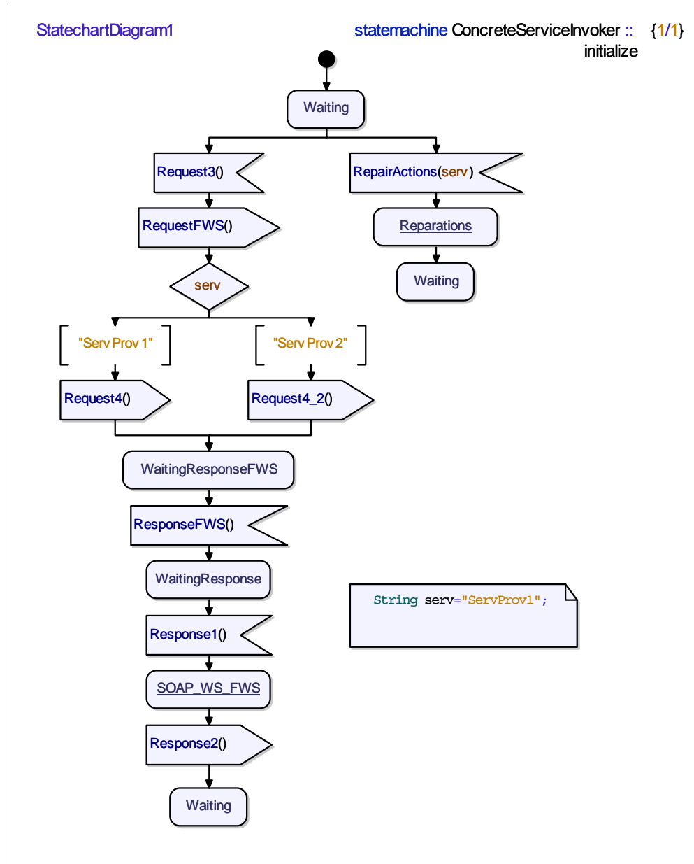
FIG. B.5 – Diagramme de machine à état de l'intercepteur Concrete Service Invoker (1/2).
