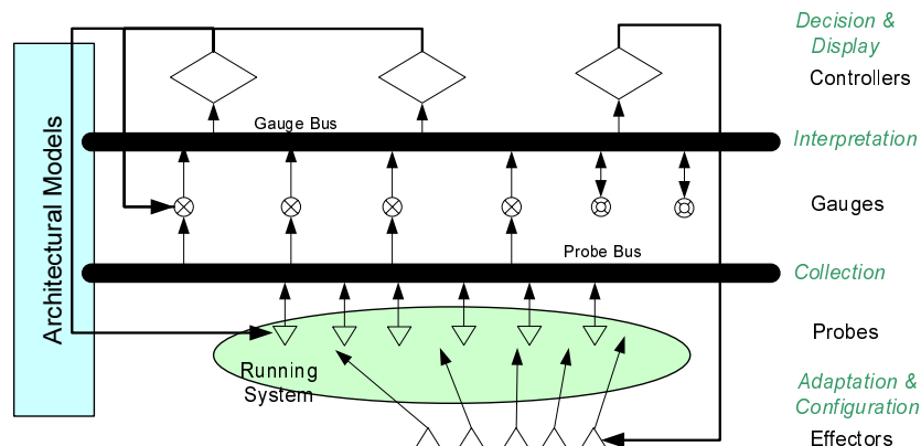
FIG. 3.11 – Architecture de l'infrastructure pour l'exécution de systèmes « self-healing », Wile et Egyed (2004).
