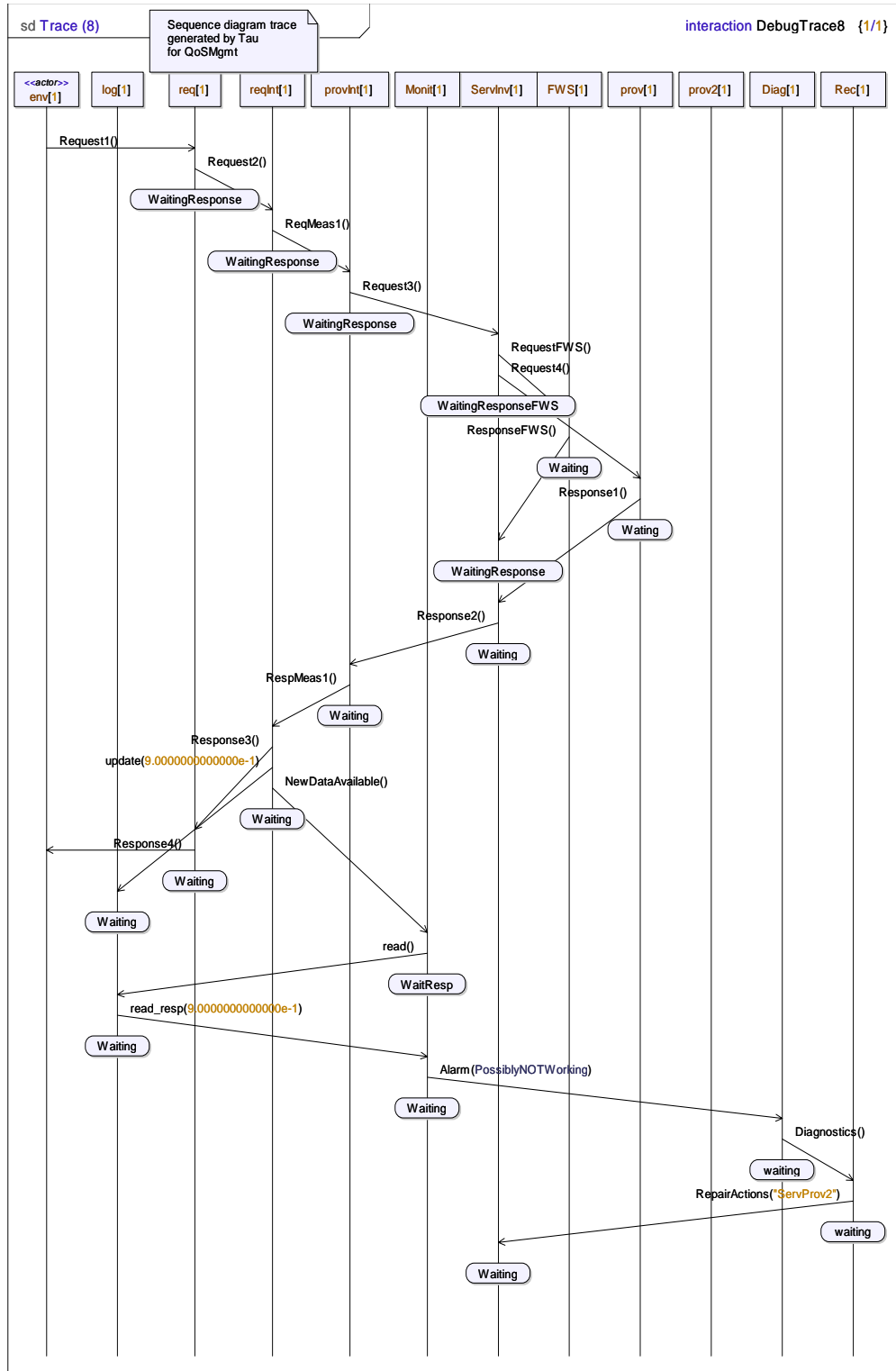
FIG. 6.27 – Simulation de l'architecture de gestion de la QoS (2/3).
