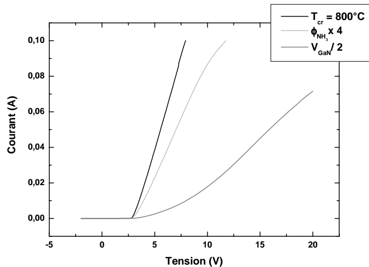
Figure 16 : Caractéristiques courant-tension des jonctions p-n.
