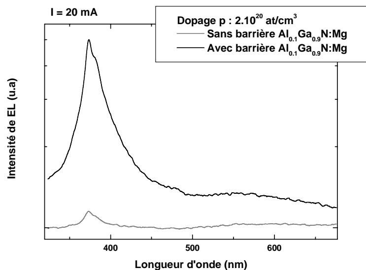
Figure 29 : Spectre d'électroluminescence des jonctions p-n avec et sans barrière \text{Al}_{0.1}\text{Ga}_{0.9}\text{N} à 20mA et à 300K.
