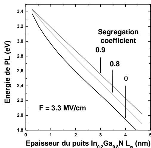
Figure 18 : Energie de PL en fonction de la largeur du puits quantique.
