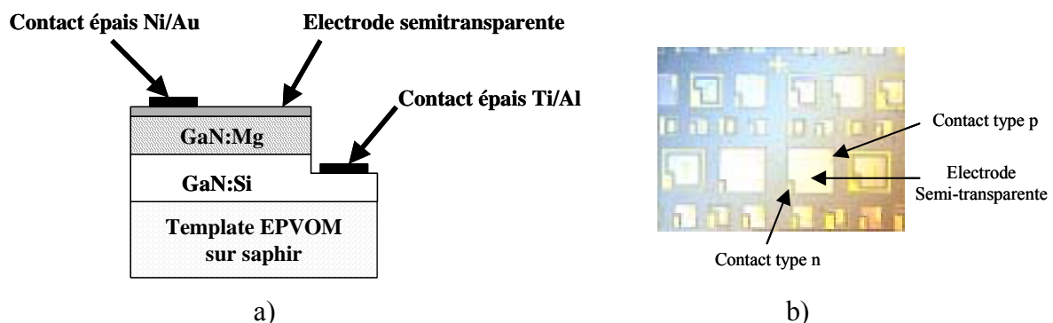
Figure 5: a) Représentation schématique de la structure des jonctions p-n et de leur différents contacts réalisés. b) Image au microscope optique de la surface d'une jonction p-n après procédé technologique.
