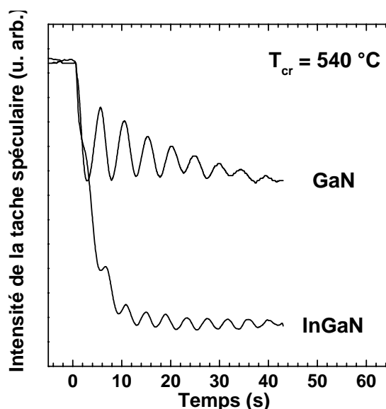
Figure 4 : Oscillations d'intensité de la tache spéculaire dans le cas de l'épitaxie de GaN ou de l'alliage InGaN à la température de croissance de 540^\circ\text{C} .
