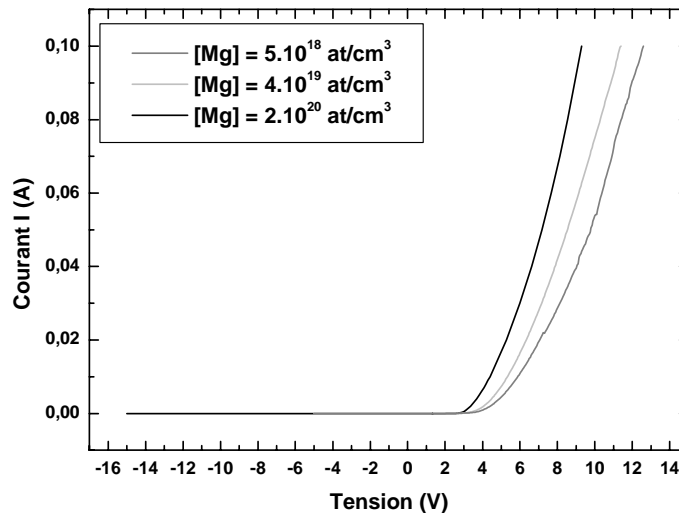
Figure 10 : Caractéristiques courant-tension des jonctions p-n pour différentes concentrations en Mg.
