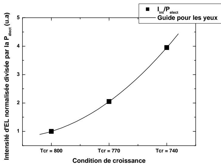
Figure 21 : Intensité d'EL normalisée par rapport à la jonction p-n standard divisée par la puissance électrique.
