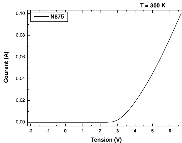
Figure 5 : Caractéristiques courant-tension de la DEL émettant à 441nm.
