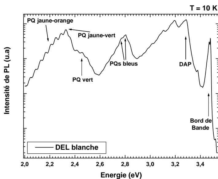
Figure 12 : Spectre de PL de la DEL blanche à large spectre.
