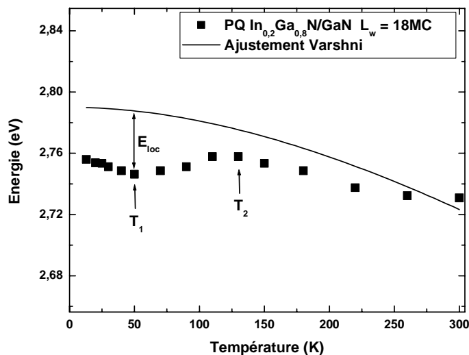
Figure 14 : Énergie de PL en fonction de la température d'un puits quantique \text{In}_{0,20}\text{Ga}_{0,8}\text{N}/\text{GaN} , ainsi que l'ajustement avec la formule de Varshni.
