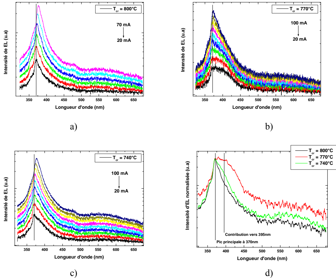
Figure 23: a)b)c) Spectre d'EL en fonction du courant des jonctions p-n étudiées dans ce paragraphe. d) Comparaison des spectres d'EL normalisés à 20 mA des trois homojonctions.
