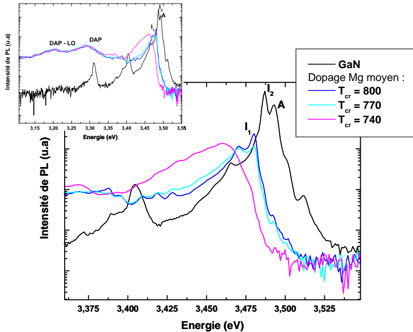
Figure 17 : Spectres de photoluminescence des jonctions p-n épitaxiées avec un flux de Mg identique mais des températures de croissance différentes.
