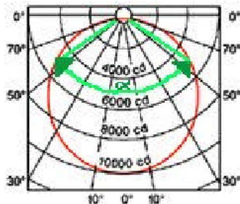
Figure 5 : Représentation schématique de l'angle d'émission d'une DEL [4].
