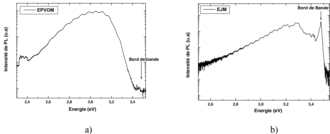
Figure 2 : Spectre de PL à 10K de couches de GaN de type p réalisées a) en EPVOM et b) en EJM.
