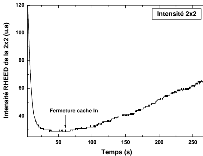
Figure 22 : Intensité de la reconstruction 2x2 en fonction du temps lors de la croissance de l'alliage \text{In}_x\text{Ga}_{1-x}\text{N} suivie d'une barrière GaN, tous deux épitaxiés à la température de croissance de 540^\circ\text{C} .
