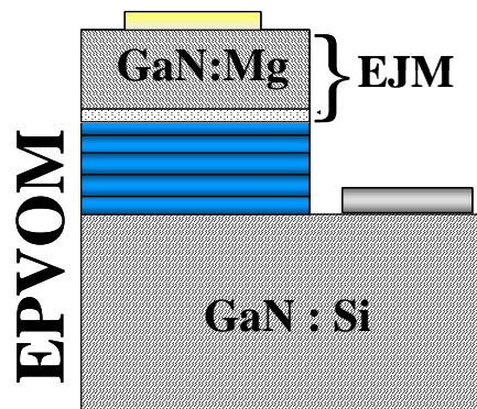
Figure 1 : Structure de la DEL hybride EPVOM/EJM.
