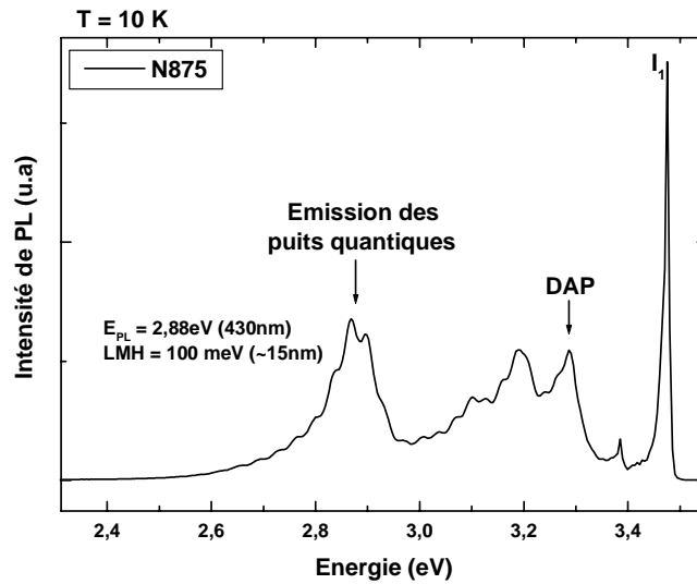
Figure 3 : Spectre de PL à 10K de la DEL émettant à 440nm.
