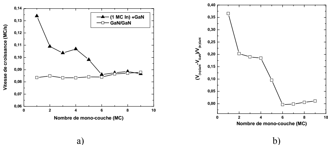
Figure 19 : a) Vitesse de croissance déterminée par mesure de RHEED de GaN (carré vide) et de GaN après déposition d'une MC d'In à la surface (triangle noir). b) Profil de composition en In déduit des mesures de vitesse de croissance.
