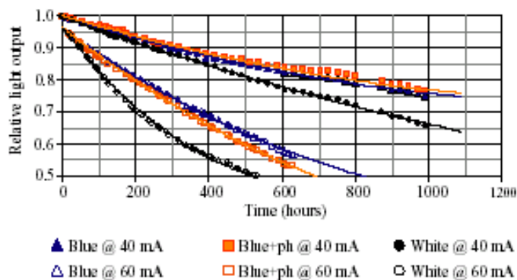
Figure 21 : Flux lumineux normalisé pour trois types de groupements de DELs (DELs blanches en noir) en fonction du temps.[24]
