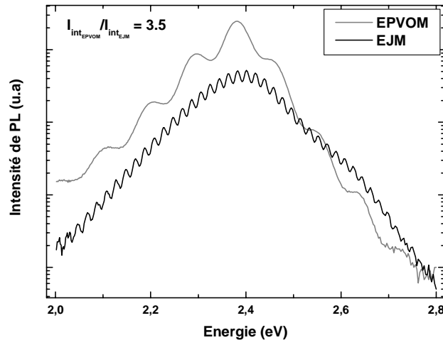
Figure 1: Spectre de PL à 300K de puits quantique (Ga,In)N/GaN épitaxiés en EPVOM et en EJM.
