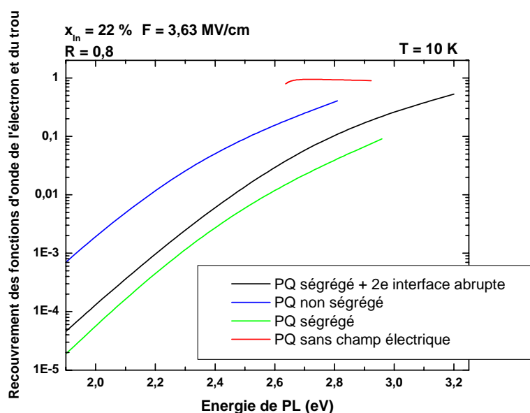
Figure 6 : Calcul du recouvrement des fonctions d'onde de l'électron et du trou en fonction de l'énergie de transition pour des largeurs de puits de 5 à 20MCs.
