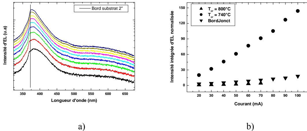
a) Spectre d'EL de la jonction p-n au bord de l'échantillon 2 pouces épitaxié à 740°C (BordJonct) en fonction de la longueur d'onde.
