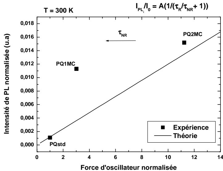
Figure 14 : Intensité intégrée de PL normalisée, par rapport à celle du PQstd à 10K, des trois puits quantiques Al_{0,1}Ga_{0,9}N/Al_{0,2}Ga_{0,8}N (carrés noirs) en fonction de la force d'oscillateur théorique normalisée ainsi que l'ajustement théorique (courbe noire) à 300 K.
