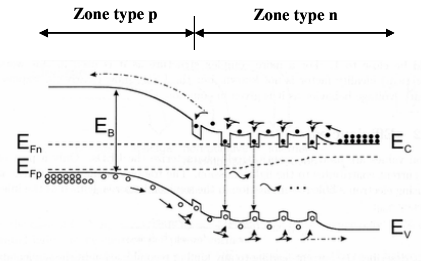
Figure 1 : Schéma d'une DEL nitride à puits quantiques en fonctionnement [1]. Les puits quantiques sont considérés dans la zone de type n en raison du dopage résiduel de type n.
