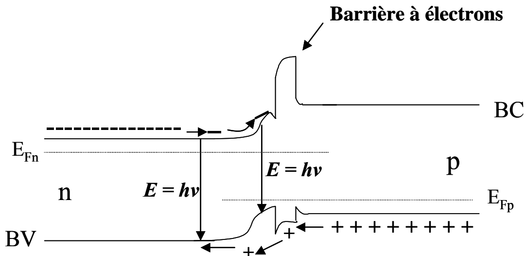
Figure 27 : Schéma de bande d'une jonction p-n en fonctionnement comportant une barrière pour les électrons à la jonction.[28]
