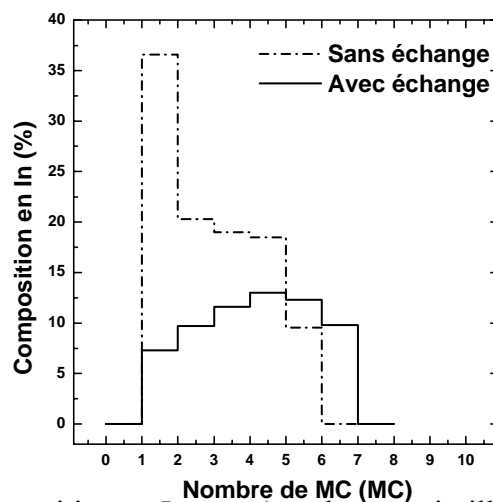
Figure 20 : Profils de composition en In sans (courbe en pointillés) et avec la prise en compte des échanges entre la n-1^{\text{ième}} et la n^{\text{ième}} mono-couche ( R = 0.8 ).
