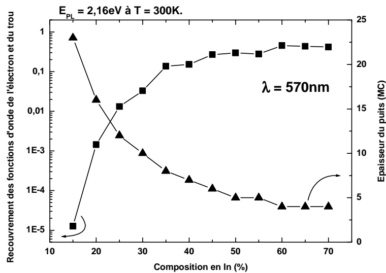
Figure 13 : Calcul du recouvrement des fonctions d'onde de l'électron et du trou d'un puits quantique \text{In}_x\text{Ga}_{1-x}\text{N}/\text{GaN} émettant à 2.16eV à 300K en fonction de la composition en In (carré), ainsi que l'épaisseur de puits correspondante (triangle).
