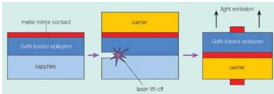
Figure 17: Procédure de la configuration utilisé par l'entreprise Osram pour augmenter le rendement d'extraction de leur DELs [15].
