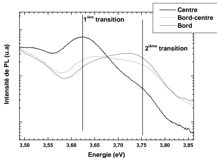
Figure 1 : Spectre de PL de l'échantillon PQ2MC suivant la position du laser à la surface de l'échantillon 2pouces.
