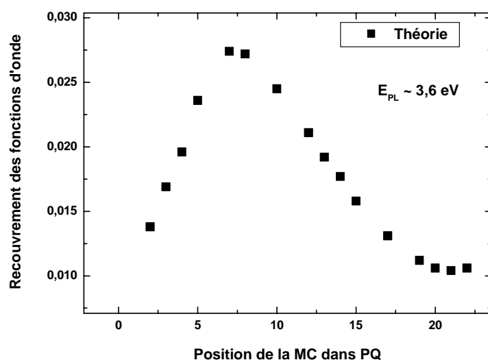
Figure 10 : Force d'oscillateur d'un puits quantique Al_{0,1}Ga_{0,9}N/Al_{0,2}Ga_{0,8}N de 24MC en fonction de la position de la MC de GaN à l'intérieur du puits.
