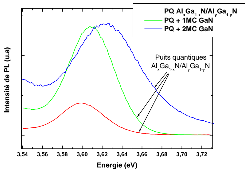
Figure 11 : Spectres de PL de GaN et des trois puits quantiques \text{Al}_{0,1}\text{Ga}_{0,9}\text{N}/\text{Al}_{0,2}\text{Ga}_{0,8}\text{N} avec 0, 1 ou 2 MC de GaN insérées à la 6 ième MC du puits.
