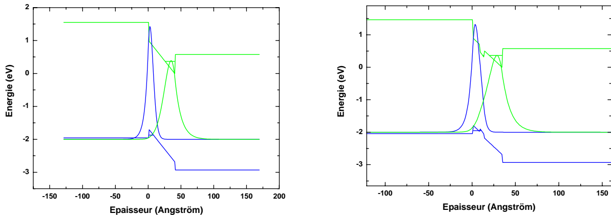
Figure 17 : Schéma de bande d'un puits quantique \text{In}_{0.2}\text{Ga}_{0.8}\text{N}/\text{GaN} standard à gauche. A droite, schéma de bande d'un puits quantique \text{In}_{0.2}\text{Ga}_{0.8}\text{N}/\text{GaN} avec insertion de 2MC d' \text{In}_{0.3}\text{Ga}_{0.7}\text{N} .
