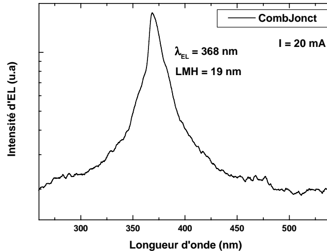
Figure 32 : Spectre d'électroluminescence de la jonction p-n combinant une couche de GaN:Mg optimisée et une couche d' \text{Al}_{0,1}\text{Ga}_{0,9}\text{N}:\text{Mg} .
