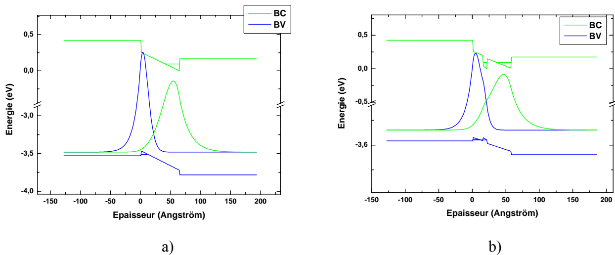
Figure 9 : a) Schéma de bande d'un puits quantique \text{Al}_{0.1}\text{Ga}_{0.9}\text{N}/\text{Al}_{0.2}\text{Ga}_{0.8}\text{N} de 25MC. b) Schéma de bande d'un puits quantique \text{Al}_{0.1}\text{Ga}_{0.9}\text{N}/\text{Al}_{0.2}\text{Ga}_{0.8}\text{N} avec l'insertion de 2 MC de GaN à l'intérieur du puits \text{Al}_{0.1}\text{Ga}_{0.9}\text{N} .
