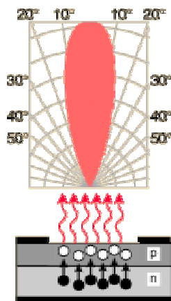
Figure 9 : Une LED émet de la lumière sous forme d'un cône. L'angle entre la normale à la surface de la LED et le bord du cône dépend de la différence d'indice entre le semi-conducteur et l'air.
