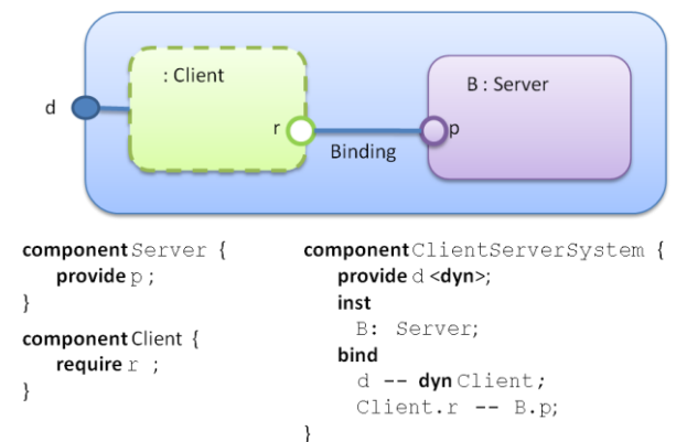
Figure 29. Exemple d'instanciation dynamique avec Darwin
