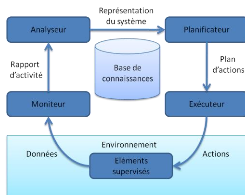
Figure 5. Architecture d'un gestionnaire "autonome" proposée par IBM
