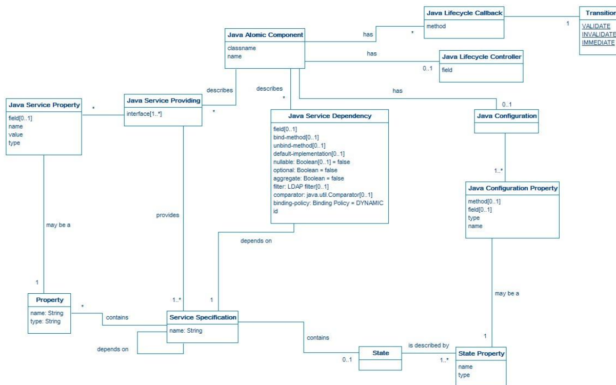
Figure 73. Modèle des types de composants atomiques implémentés en Java
