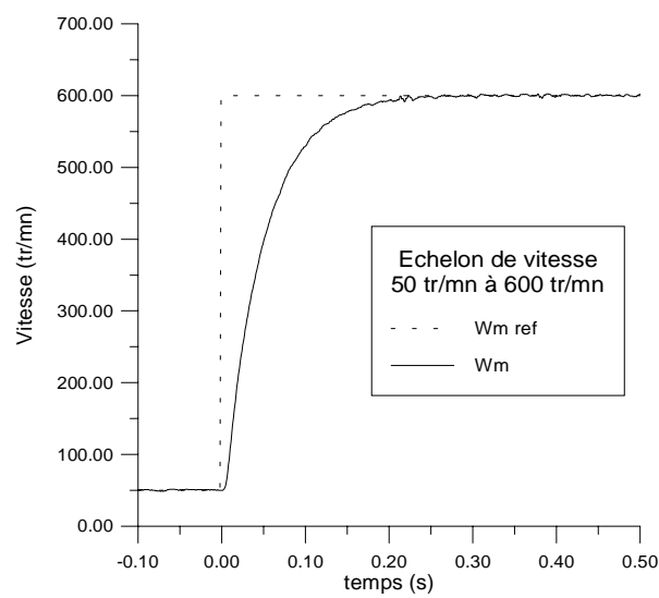
Figure 5.21 Vitesse de la machine, IRFO
