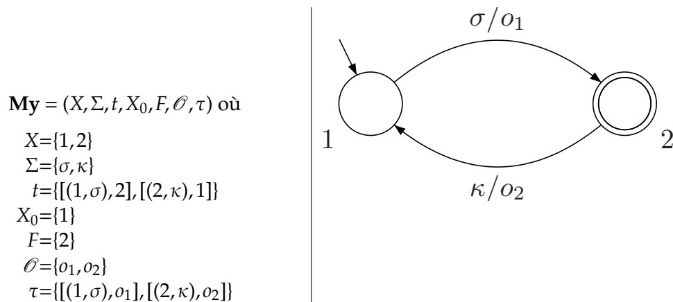
FIGURE 2.8 – Deux représentations de My (un automate de Mealy)
