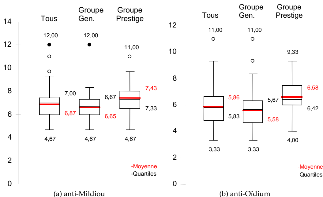
FIGURE 1.1 – Boîte de Tuckey du nombre annuel moyen de traitements (années 2004,2005,2006 sur un échantillon de 100 exploitations bordelaises). « Groupe Gen. » renvoie aux appellations vin Bordeaux générique et « Groupe Prestige » aux appellations haut de gamme, voir la caractérisation de chaque groupe tab. 1.1
