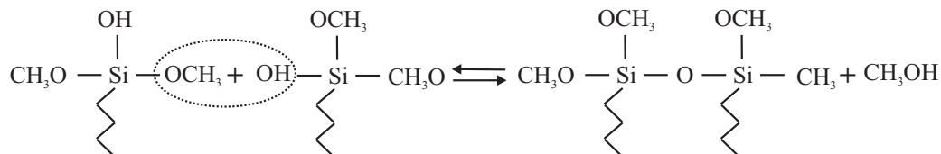
FIG. II.6 – Réaction de déalcoolisation.
