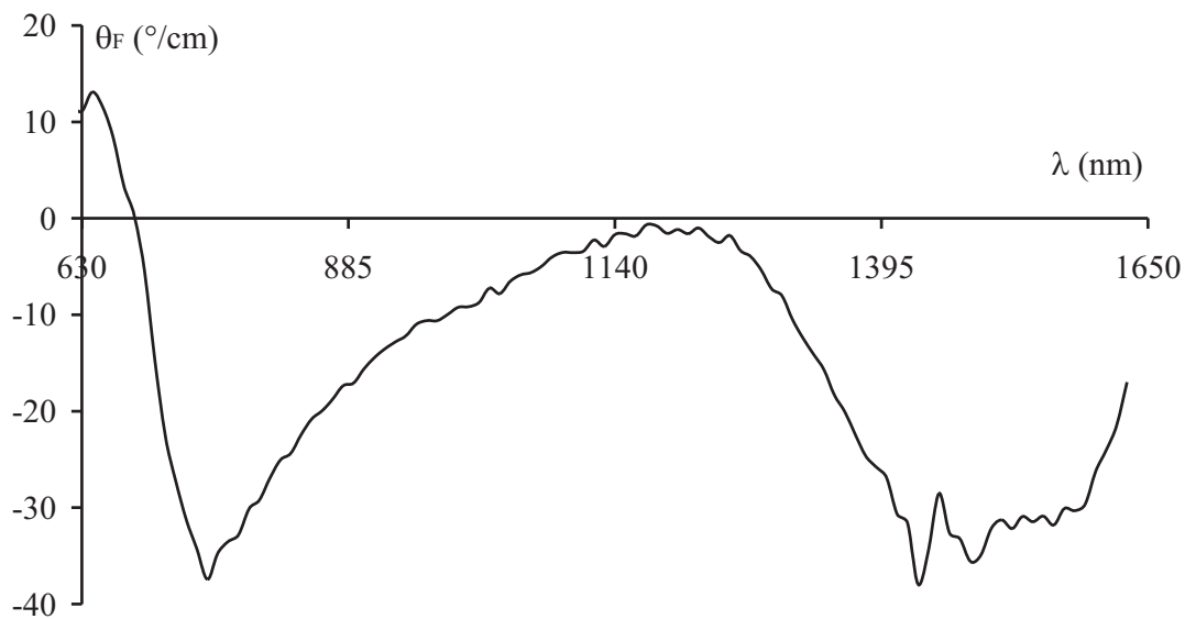
FIG. IV.7 – Variation de la rotation Faraday spécifique de nanoparticules de ferrite de cobalt en fonction de la longueur d'onde. La concentration en particules est de 0,2\% .
