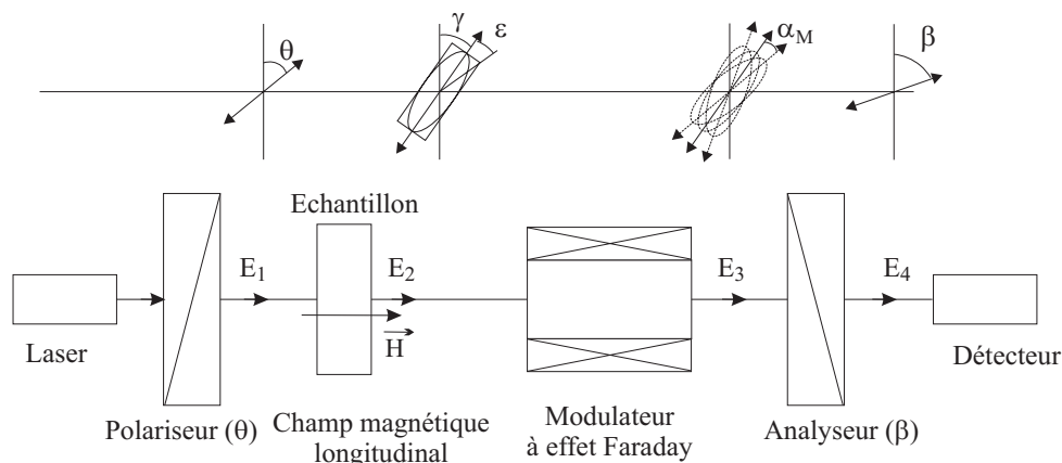
FIG. II.31 – Montage optique pour la détermination de l'inclinaison \gamma .
