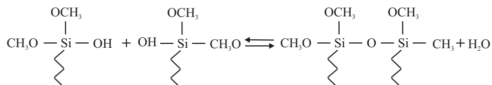
FIG. II.5 – Réaction de déshydratation.
