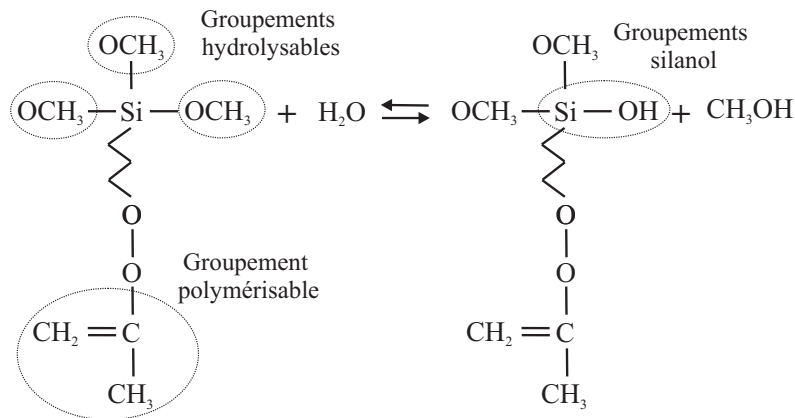
FIG. II.2 – Réaction d'hydrolyse du méthacryloxypropyltriméthoxysilane MAPTMS.
