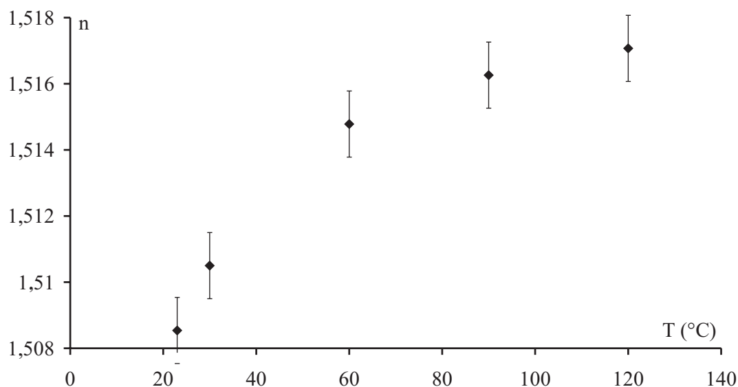
FIG. III.8 – Variation des indices de réfraction n de la matrice \text{SiO}_2/\text{ZrO}_2 non dopée, ayant subi un pré-traitement thermique durant 60 minutes, avec la température de recuit.
