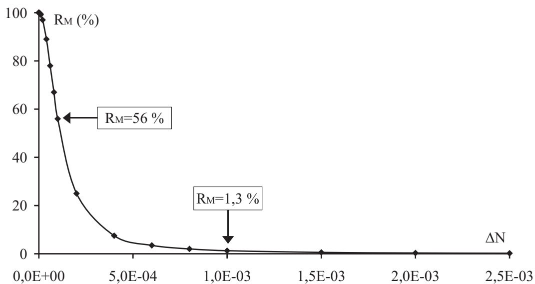
FIG. III.20 – Evolution du taux de conversion TE-TM en fonction de la biréfringence modale, pour une rotation Faraday spécifique de 250 °/cm à \lambda = 820 nm.
