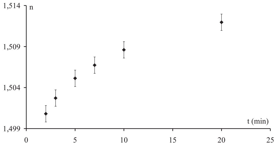
FIG. III.6 – Variation de l'indice de réfraction du matériau en fonction de la durée d'insolation UV à chacune de deux longueurs d'onde 365 nm et 254 nm. Il s'agit d'un traitement « doux » à la puissance 1 mW/cm 2 .
