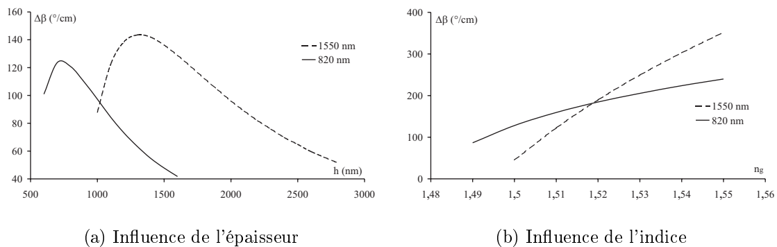
FIG. I.9 – Evolution de la différence de phase géométrique correspondant au mode fondamental pour un guide planaire isotrope à saut d'indice déposé sur pyrex ( n=1,472 ) : en fonction de l'épaisseur avec indice valant 1,51 (cas a) et en fonction de l'indice pour une épaisseur de 1100 nm (cas b). Dans tous les cas, l'épaisseur est prise inférieure à l'épaisseur de coupure du deuxième mode TE, garantissant un guide monomode.
