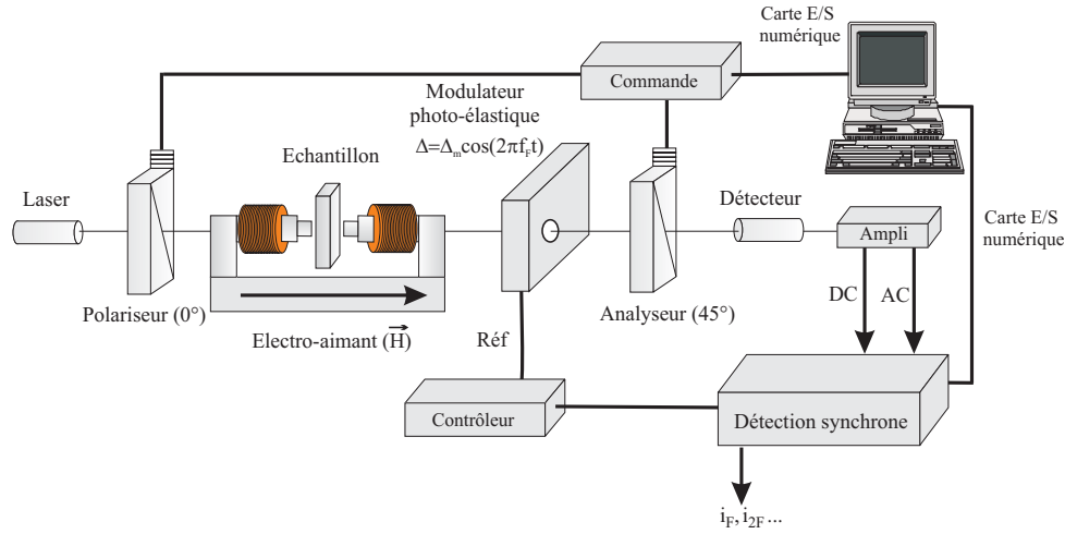
FIG. II.33 – Dispositif expérimental utilisant le modulateur photoélastique.
