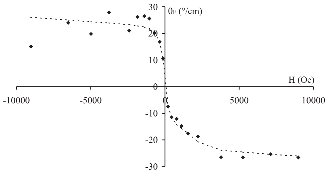
FIG. I.17 – Rotation Faraday mesurée en espace libre, transversalement au plan d'une couche mince constituée d'une matrice SiO_2/TiO_2 dopée en Maghémite et déposée sur Pyrex. (Source : F. Royer, Thèse de Doctorat, INPG, Grenoble, 2004)
