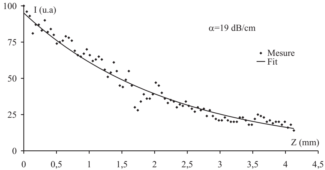
FIG. IV.27 – Intensité normalisée de la lumière, captée par la caméra CCD placée en face de la couche mince, en fonction de la distance de propagation.
