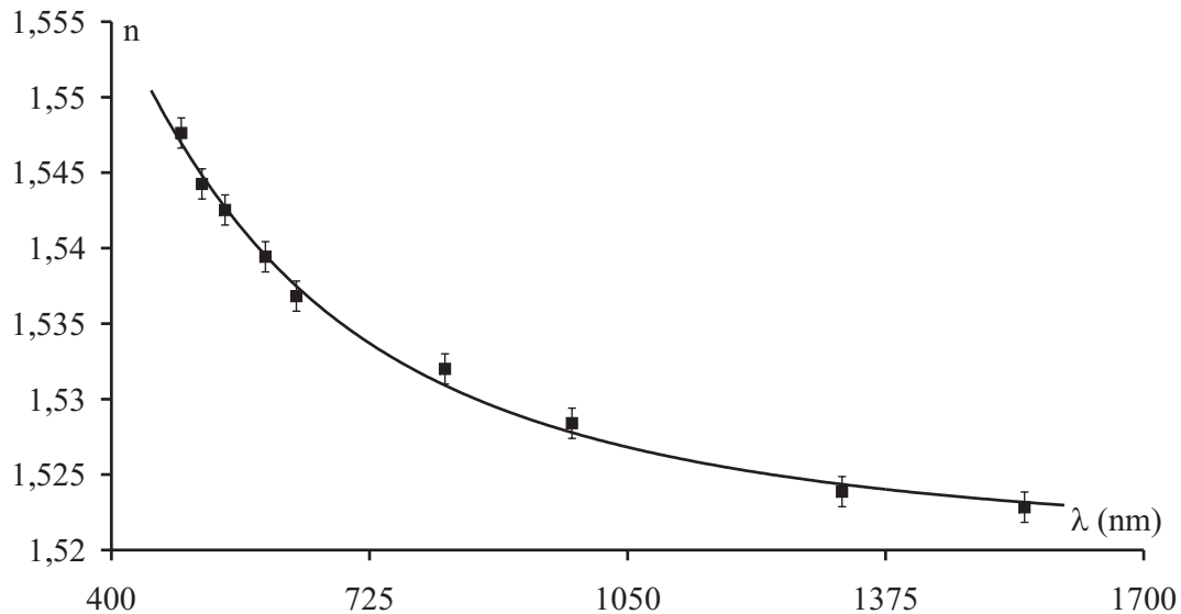
FIG. III.5 – Variation de l'indice du matériau en fonction de la longueur d'onde d'une couche mince constituée d'une matrice 10 :3 :3. Cette évolution de l'indice suit la loi de dispersion de Cauchy.
