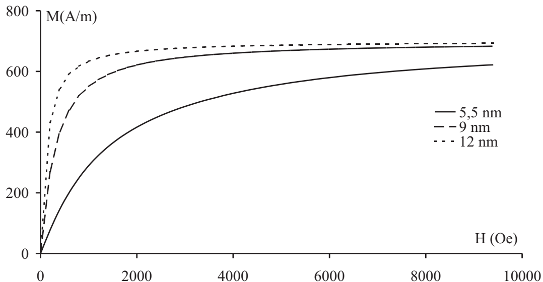
FIG. IV.3 – Courbes d'aimantation de trois différents échantillons de ferrofluide de ferrite de cobalt de même concentration \phi = 0,2\% .
