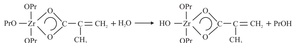
FIG. II.4 – Réaction d'hydrolyse de l'alcoxyde de zirconium complexé.
