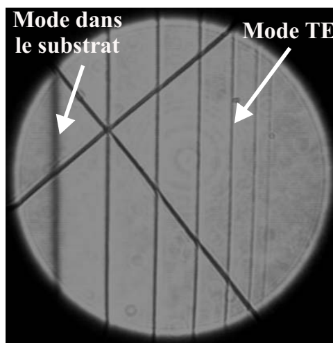
FIG. III.21 – Photo prise par une caméra CCD placée en face du faisceau réfléchi de la base du prisme en contact avec la couche mince. Les lignes noires correspondent aux modes TE propageant dans le guide d'onde.
