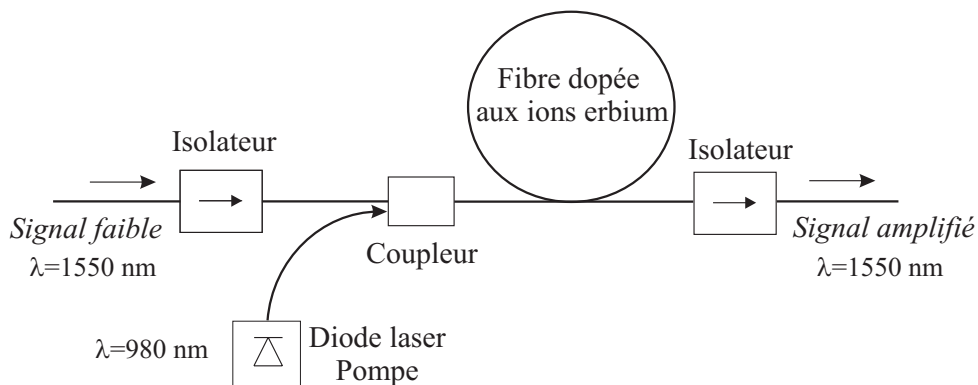
FIG. I.2 – Principe de fonctionnement des amplificateurs à fibre EDFA.
