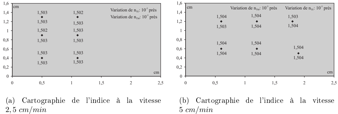
FIG. III.10 – Cartographie de l'indice à deux différentes vitesses de tirage. Les losanges correspondent aux points testés sur la lame. A chaque point sont indiquées les valeurs d'indice issues du calcul M-lines, au dessus du point pour les modes TE et en dessous pour les TM.
