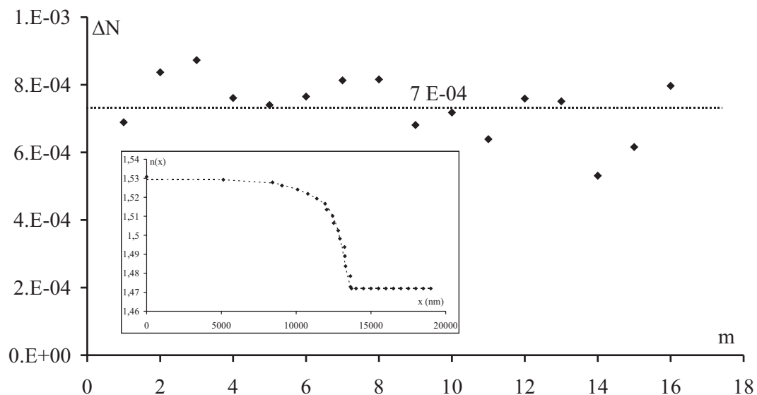
FIG. III.15 – Profil à gradient d'indice, correspondant à une couche mince élaborée à une vitesse de tirage de 7\text{ cm/min} , avec l'évolution de la biréfringence modale avec l'ordre de mode.
