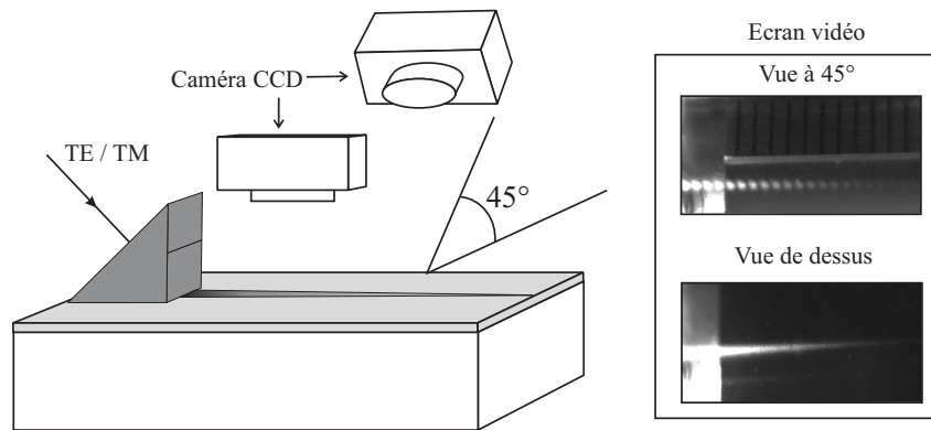
FIG. II.29 – Dispositif de diffusion en surface. Si la caméra est placée en face à la couche, on observe le trait de guidage. Si la caméra est placée à 45^\circ , on observe des franges d'interférences qui apparaissent dans le faisceau.
