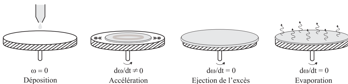
FIG. II.11 – Les 4 étapes de dépôt par la technique spin-coating . \omega est la vitesse de la rotation du substrat
