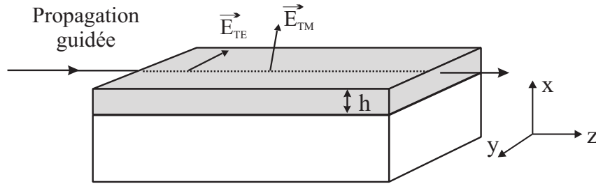
FIG. II.27 – Représentation de la propagation guidée de l'onde. Deux modes de propagation possibles : TE et TM
