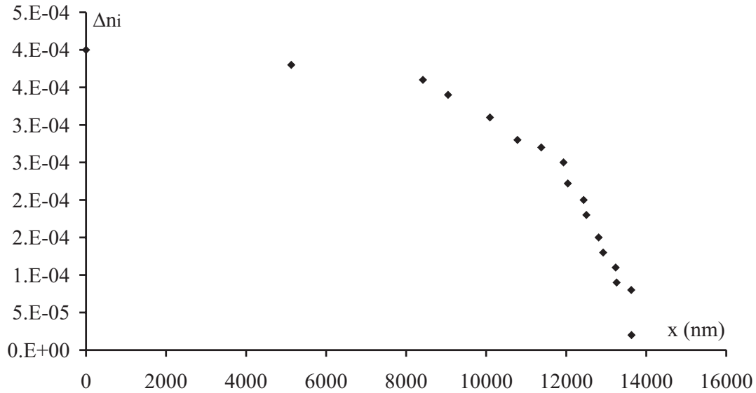
FIG. III.17 – Modèle de gradient d'anisotropie intrinsèque en fonction de la profondeur du guide à étudier.
