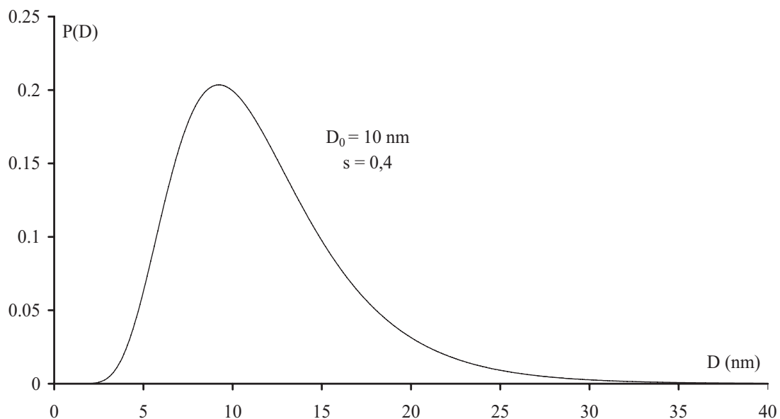
FIG. II.9 – Distribution en diamètre de type log-normale.
