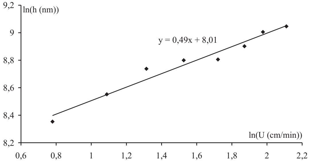
FIG. III.1 – Variation du logarithme de l'épaisseur en fonction du logarithme de la vitesse de tirage. La mesure est effectuée à 633 nm.
