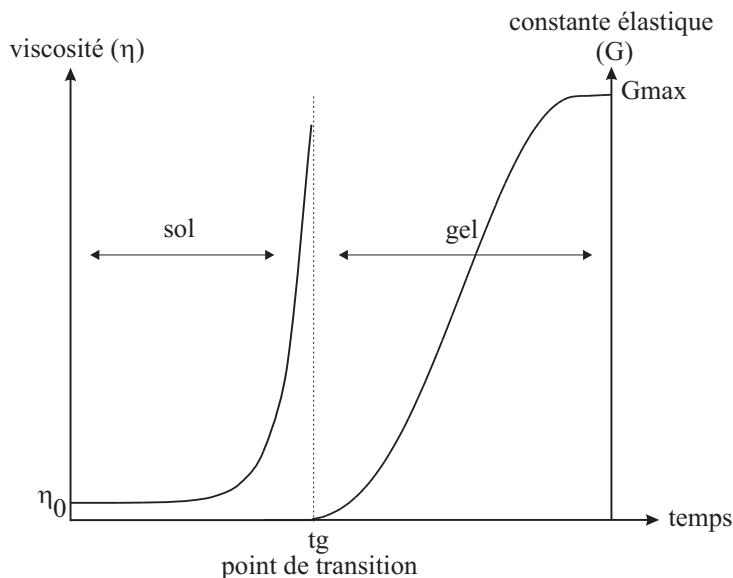
FIG. II.8 – Evolution de la viscosité en phase « sol » et de la constante élastique en phase « gel » en fonction de temps.
