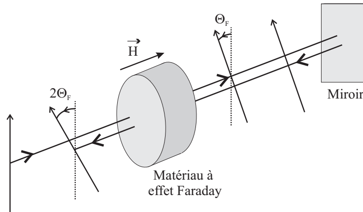
FIG. I.5 – Évolution de l'état de polarisation d'une onde rectiligne lors d'un aller-retour au sein d'un matériau soumis à un champ magnétique.
