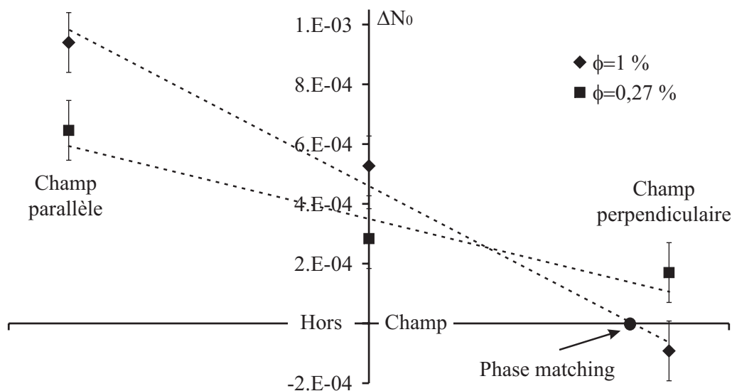
FIG. IV.22 – Biréfringence de mode fondamentale \Delta N_0 = N_{TE_0} - N_{TM_0} en fonction de l'orientation du champ de gélification de 0,5\text{ T} d'amplitude, pour deux différentes concentrations. La longueur d'onde d'étude est 820 nm .
