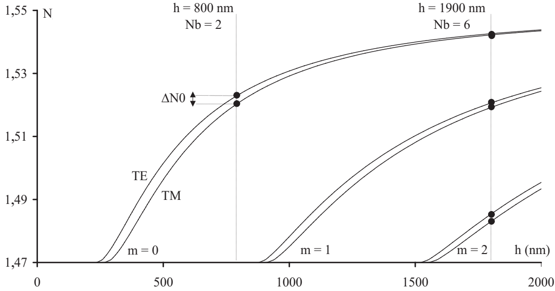
FIG. I.8 – Représentation graphique des équations de dispersion I.16 et I.17 pour \lambda = 633 \text{ nm} . Il s'agit d'un guide d'indice 1,55 déposé sur un substrat de pyrex (indice 1,47). Pour h = 800 \text{ nm} le guide est monomode TE-TM. Pour h = 1900 \text{ nm} le guide possède 3 modes TE-TM.
