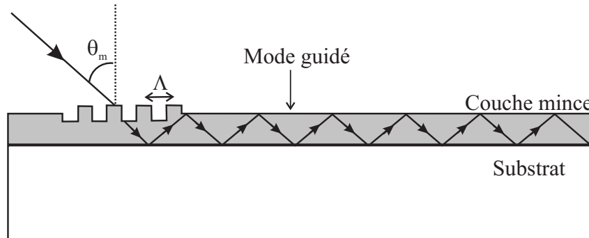
FIG. II.19 – Illustration du couplage par réseau. \Lambda est le pas du réseau et \theta_m est l'angle d'incidence.
