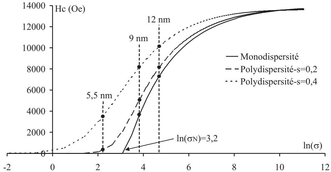
FIG. IV.18 – Représentation du champ coercitif en fonction de \sigma . Les traits continu et pointillé correspondent respectivement des assemblées monodisperse et polydisperse de nanoparticules ( s = 0,2 et 0,4 ) monodomaines, uniaxes soumises à un champ magnétique appliqué.
