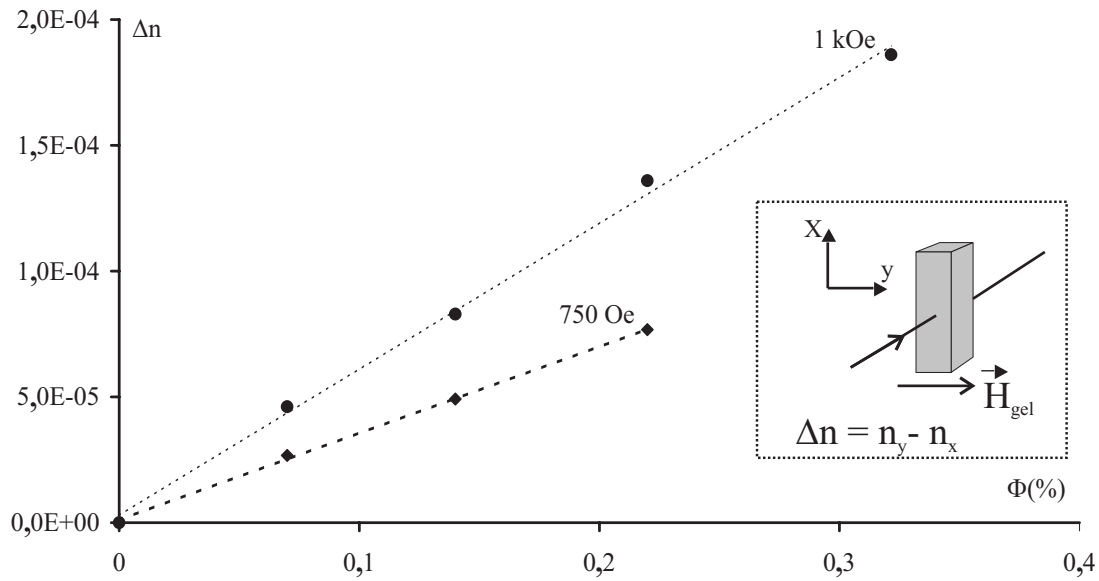
FIG. I.15 – Anisotropie linéaire permanente \Delta n au sein d'un gel dopé en nanoparticules de Maghémite. Evolution en fonction de la concentration volumique \phi en nanoparticules pour deux valeurs différentes du champ de gélification. (Source : D. Jamon, Thèse de Doctorat, Université Jean Monnet, St-Étienne, 2000)
