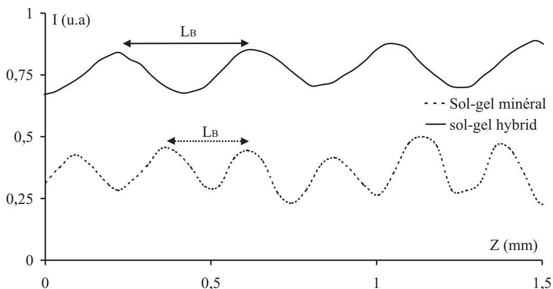
FIG. III.19 – courbe de l'intensité de la lumière en fonction de la distance de propagation de lumière dans la couche mince.
