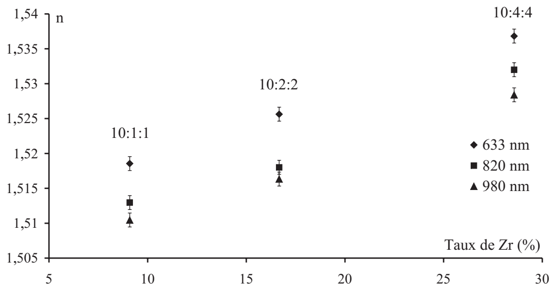
FIG. III.4 – Variation de l'indice de réfraction du matériau en fonction du taux de zirconium. Les valeurs sont mesurées par la techniques M-lines à trois différentes longueurs d'onde.
