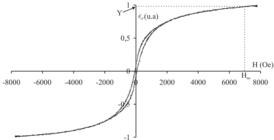
FIG. II.34 – Courbe d'ellipticité mesurée à 820 nm, à l'aide du modulateur photoélastique pour un guide d'onde dopé (couche mince et substrat).
