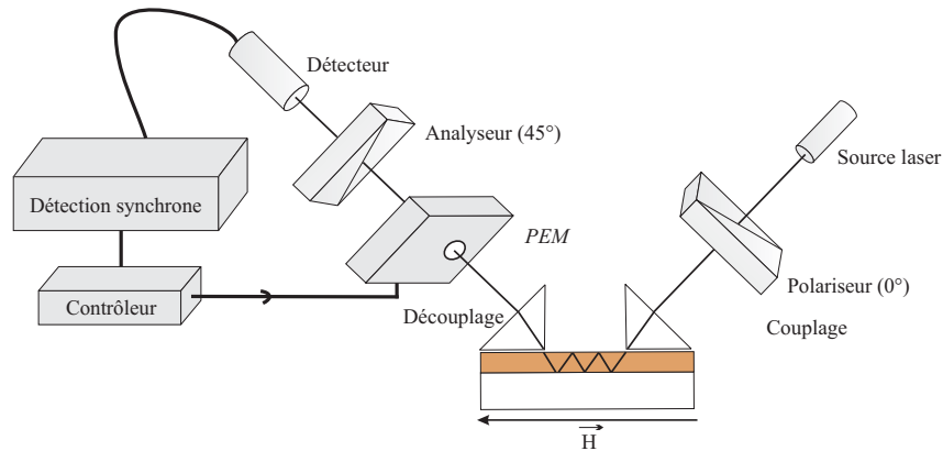
FIG. IV.28 – Dispositif de mesure de la conversion de mode TE-TM par modulation de champ.
