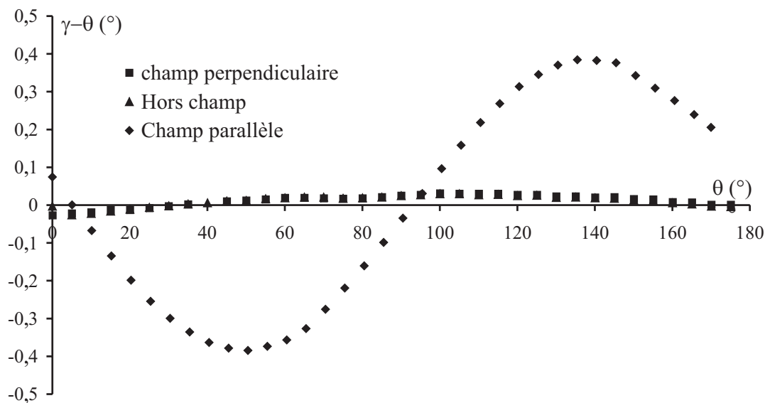
FIG. IV.24 – Représentation de la biréfringence planaire en terme de \gamma - \theta , pour des échantillons constitués d'une matrice \text{SiO}_2/\text{ZrO}_2 dopée par des nanoparticules de Cobalt ( \phi = 1\% ). \theta est l'orientation de la polarisation incidente, \gamma celle de sortie.
