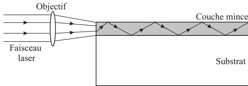
FIG. II.17 – Injection de lumière par la tranche, dans une couche mince.
