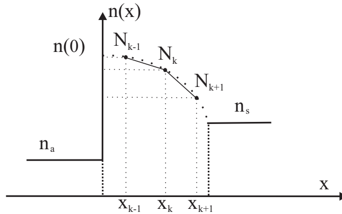
FIG. II.24 – Exemple de profil à gradient d'indice avec son interpolation linéaire entre chaque point tournant consécutif.
