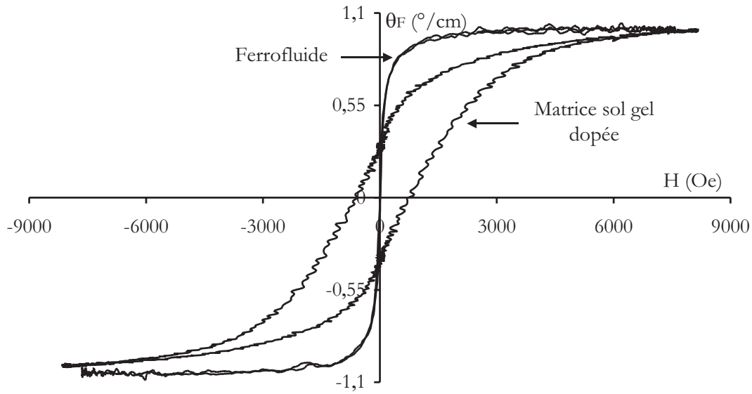
FIG. IV.12 – Evolution de la rotation Faraday normalisée en fonction du champ magnétique pour une dispersion dans un ferrofluide et dans une matrice \text{SiO}_2/\text{TiO}_2 . La mesure est effectuée à la longueur d'onde 820 nm.
