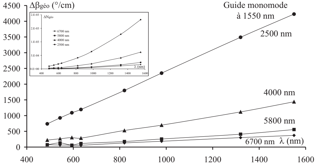
FIG. III.11 – Evolution de la différence entre les constantes de propagation \Delta\beta correspondante à la biréfringence géométrique fondamentale pour un guide planaire déposé sur pyrex ( n=1,472 ) en fonction de la longueur d'onde, pour différentes valeurs d'épaisseur.
