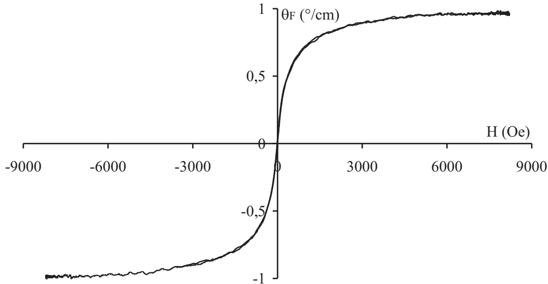
FIG. IV.14 – Allure de la rotation Faraday d'une matrice sol gel dopée par des nanoparticules de Magnémité. La mesure est effectuée 633 nm.
