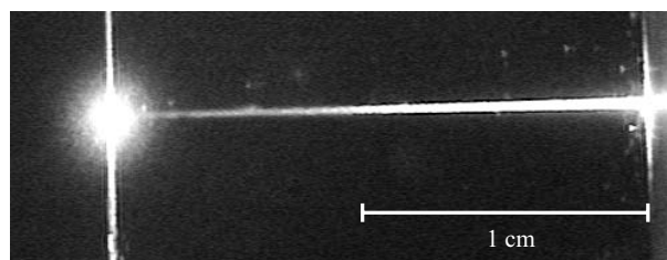
FIG. IV.26 – Visualisation du trait de guidage dans une couche mince dopée à 0,09 %. La mesure est réalisée à la longueur d'onde 820 nm.
