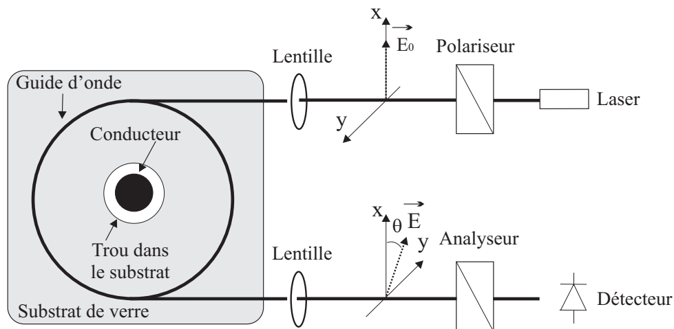
FIG. I.3 – Configuration conventionnelle du capteur de courant à effet Faraday.
