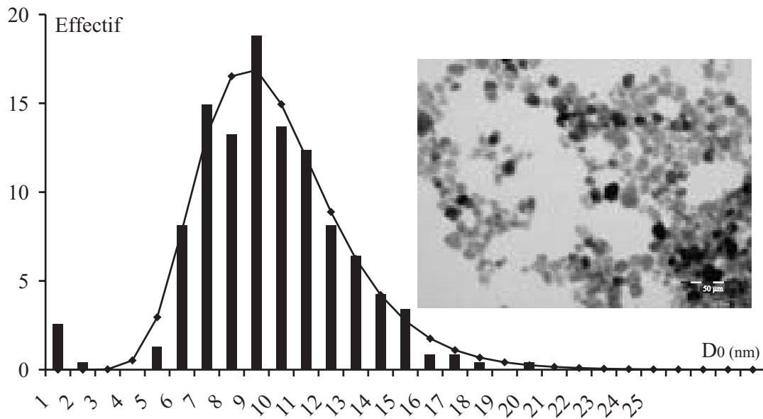
FIG. II.10 – Distribution en diamètre de l'échantillon S333. Le résultat est obtenu à partir de la photo placée en insert.
