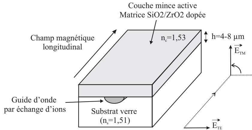
FIG. IV.30 – Illustration du composant à réaliser.
