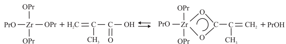
FIG. II.3 – Réaction de complexation de l'alcoxyde de zirconium avec l'acide méthacrylique.
