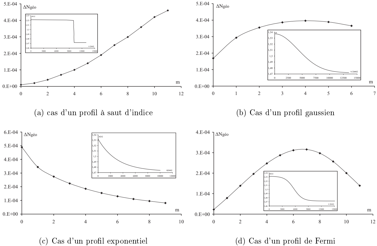
FIG. III.12 – Evolution de la biréfringence géométrique en fonction de l'ordre de mode, selon quatre différents profils d'indice.
