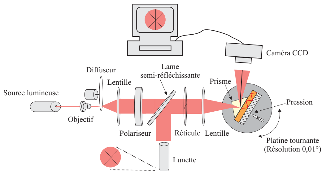
FIG. II.22 – Banc de mesure de spectroscopie de lignes noires. Un faisceau convergent de lumière éclaire le prisme. Il y a couplage ce qui apparaît comme une ligne noire sur l'écran.
