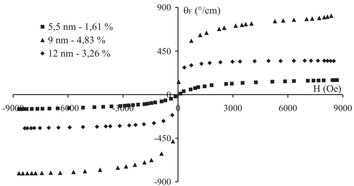
FIG. IV.2 – Rotation Faraday spécifique de trois différents échantillons de ferrite de Cobalt. Evolution en fonction du champ magnétique appliqué. La longueur d'onde de mesure est 820 nm.
