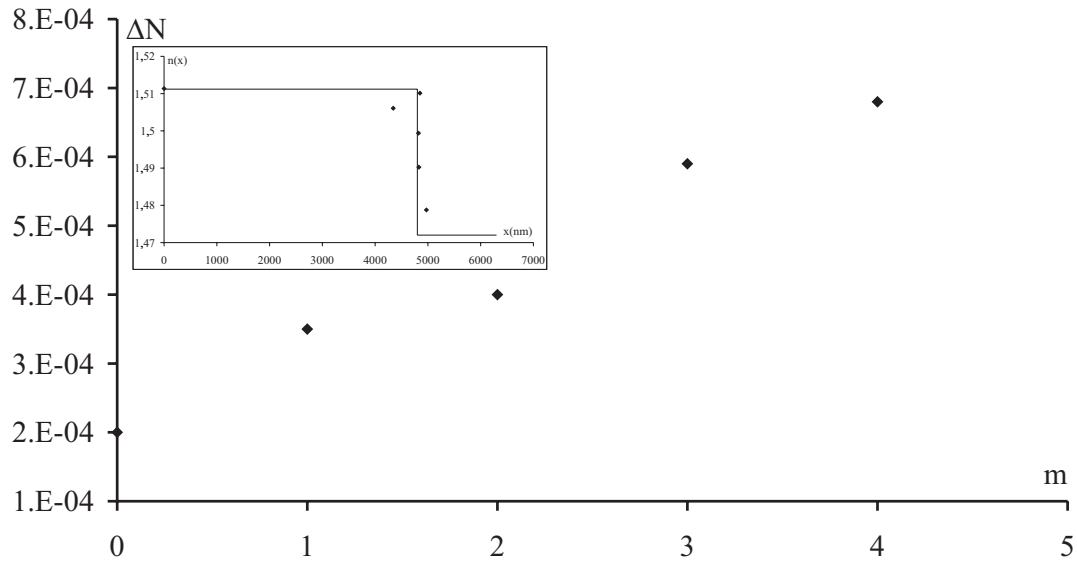
FIG. III.14 – Evolution de la biréfringence modale en fonction de l'ordre de mode pour une couche d'épaisseur 4,8\mu\text{m} possédant un profil à saut d'indice .
