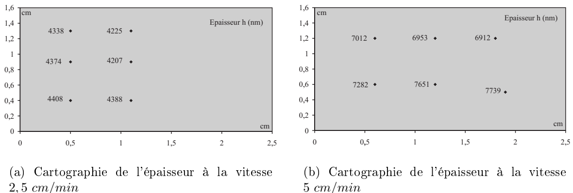
FIG. III.2 – Cartographie de l'épaisseur à deux différentes vitesses de tirage. Les losanges correspondent au points testés sur la lame. A chaque point est indiquée la valeur d'épaisseur.
