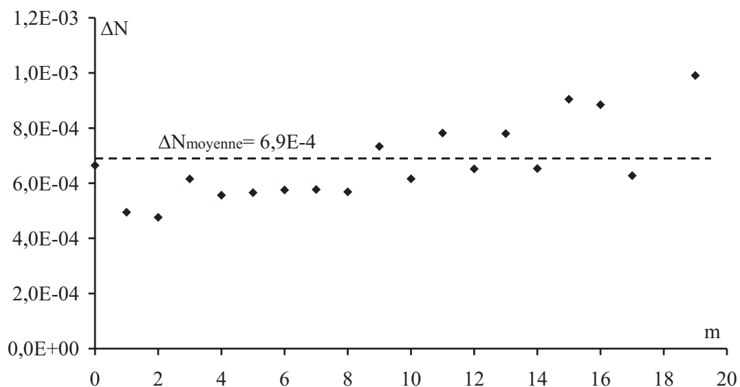
FIG. III.18 – Evolution de la biréfringence modale calculée par la méthode WKB en fonction de l'ordre de mode, pour un profil à gradient d'indice.
