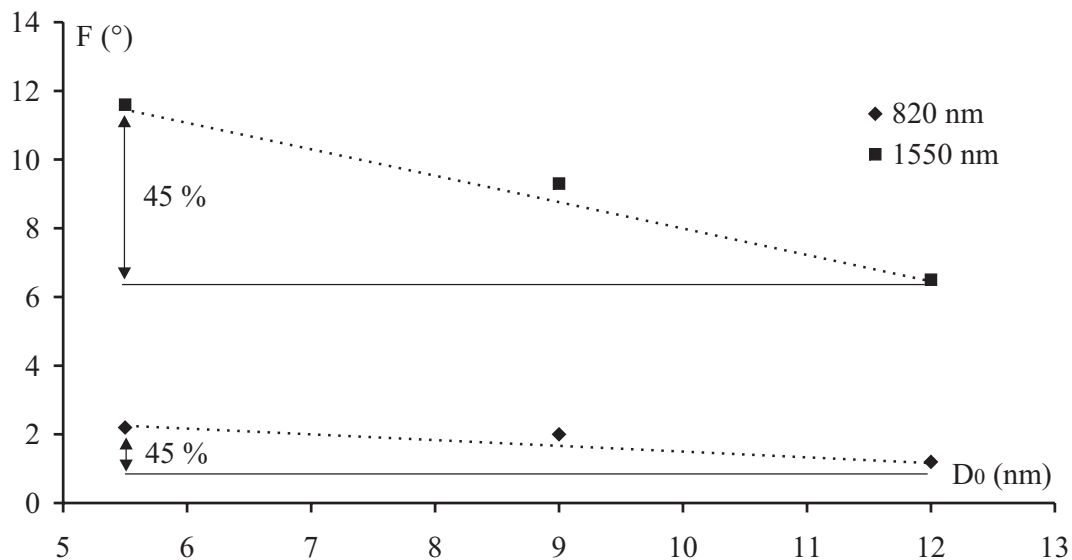
FIG. IV.9 – Variation du facteur mérite F de rotation Faraday avec le diamètre moyen de différents échantillons utilisés ; à deux différentes longueurs d'onde : 820 \text{ nm} et 1550 \text{ nm} .
