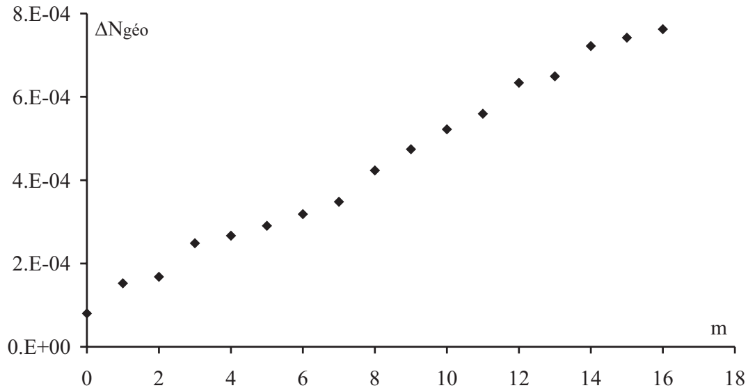
FIG. III.16 – Evolution de la biréfringence géométrique, calculée par la méthode WKB pour le profil de figure III.15, en fonction de l'ordre de mode.
