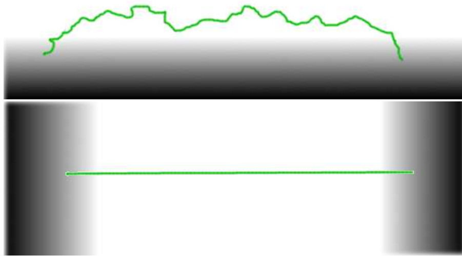
FIG. 9: Comparaison entre les géométries expérimentale et modèle. En haut : la géométrie expérimentale : une molécule d'ADN étirée à 70% et attachée par ses extrémités sur une surface réfléchissante. En bas : la géométrie utilisée dans le modèle : un cylindre entre deux surfaces réfléchissantes.
