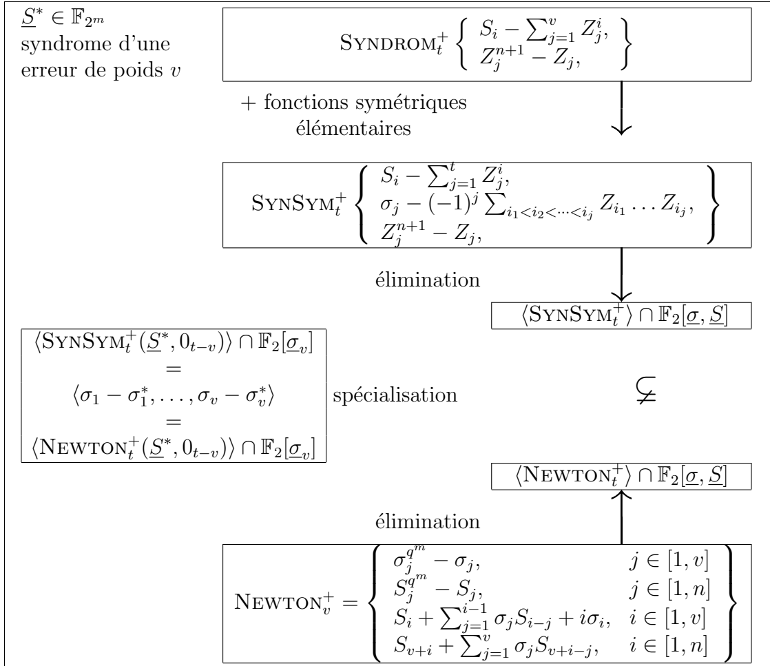
FIG. 6.1 – Idéaux zéro-dimensionnels utilisés pour le décodage des codes cycliques.
