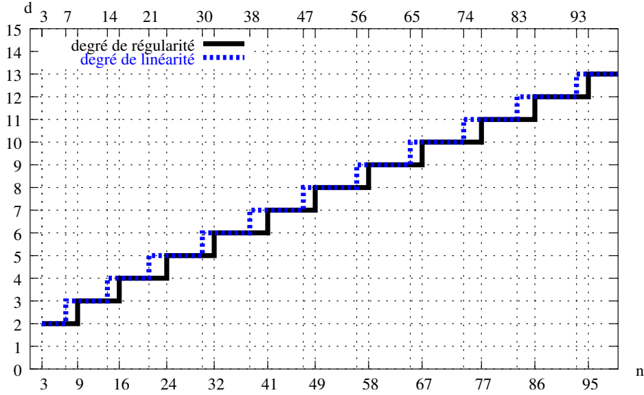
FIG. 5.1 – Comparaison des degrés de régularité et de linéarité, équations quadratiques
