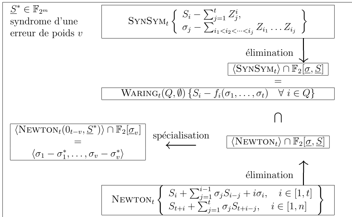
FIG. 6.2 – Idéaux de dimension positive utilisés pour le décodage des codes cycliques
