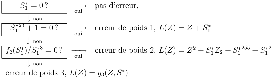
FIG. 2.2 – Algorithme de décodage du code de Golay de longueur 23.
