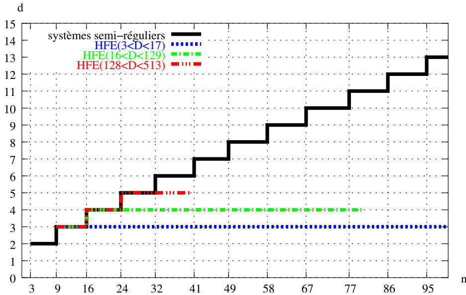
FIG. 5.3 – d -Régularité des systèmes HFE
