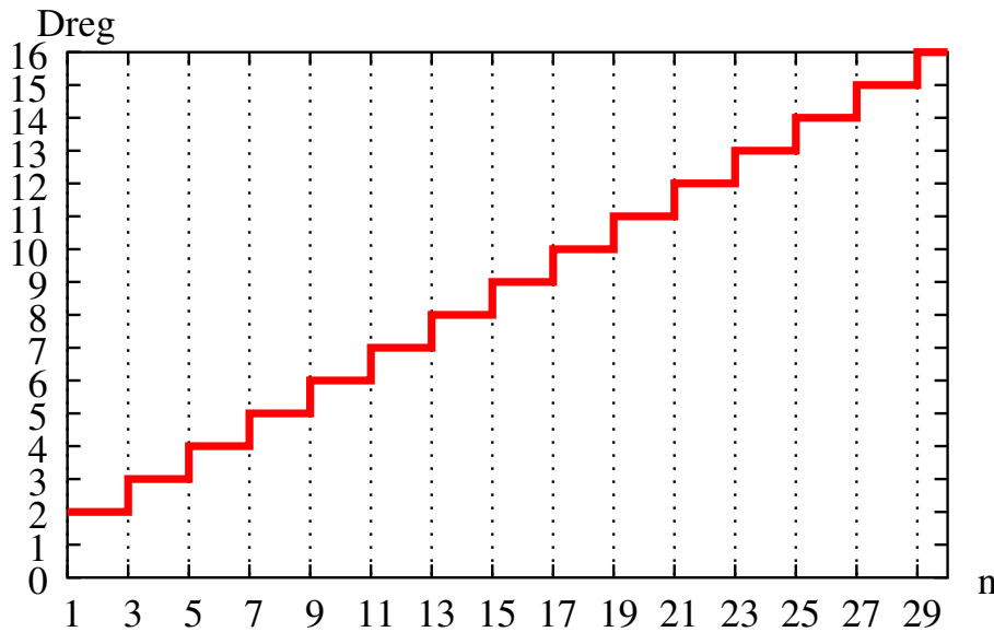
FIG. 3.1 – H(I) pour m = n + 1 polynômes quadratiques
