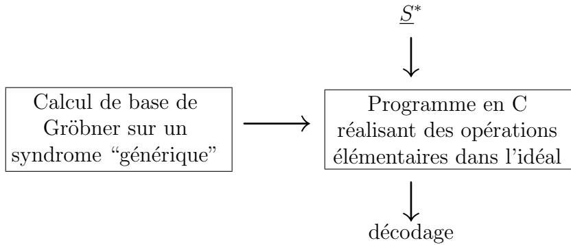
FIG. 6.5 – Méthode de la trace du pré-calcul
