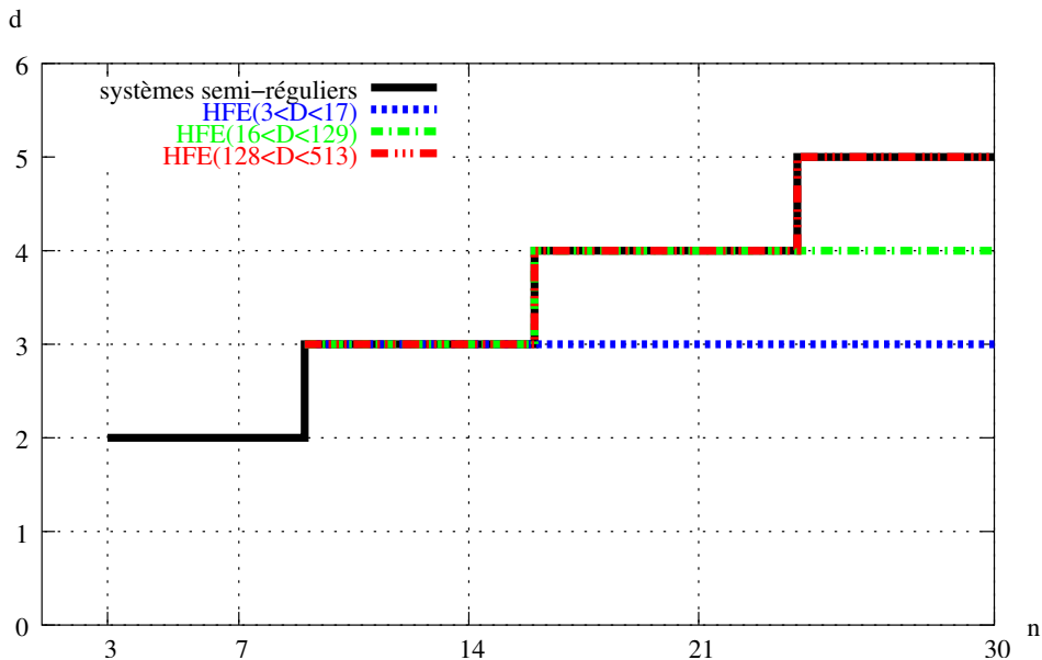
FIG. 5.2 – Comparaison des systèmes HFE et des systèmes aléatoires
