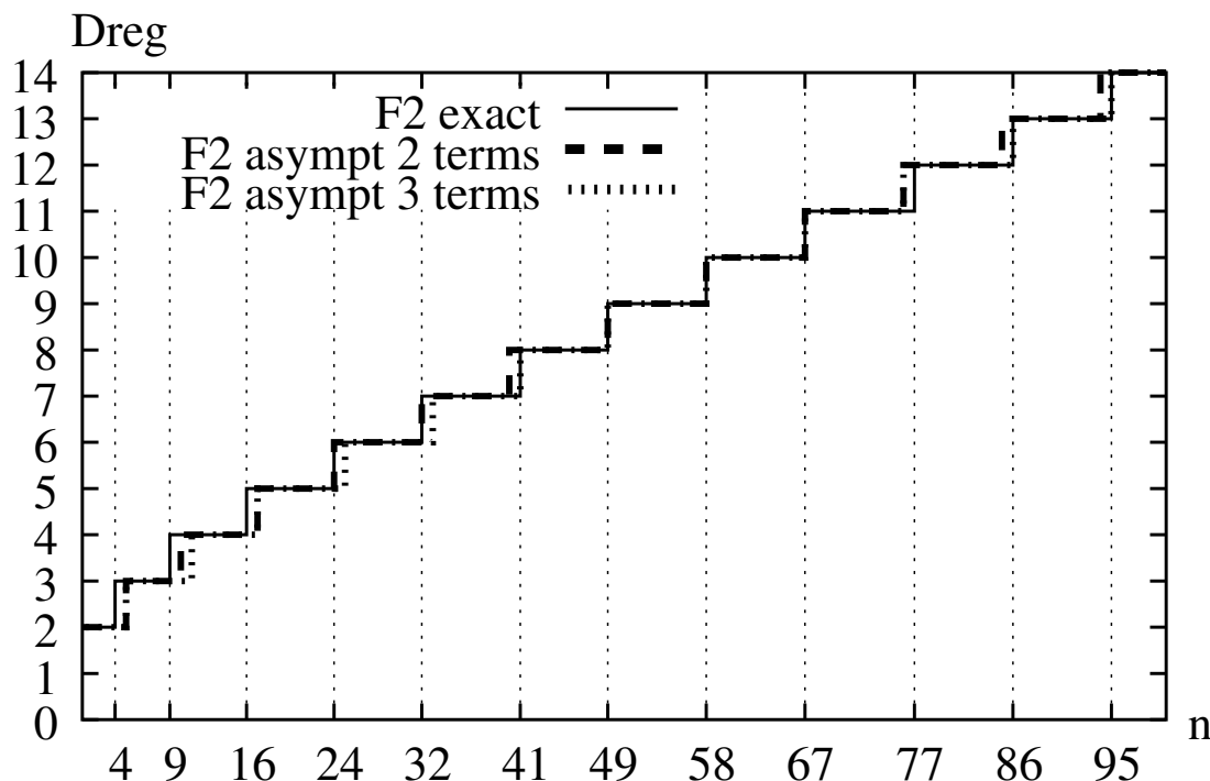
FIG. 4.1 – Comparaison de la régularité et de son développement asymptotique pour m = n équations quadratiques sur \mathbb{F}_2 .
