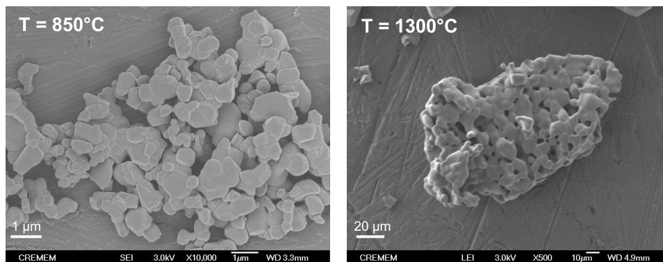
FIGURE IV.6 – Clichés MEB des échantillons ZnO : 6% Co recuits respectivement à 850°C (gauche) et 1300°C (droite) sous air.
