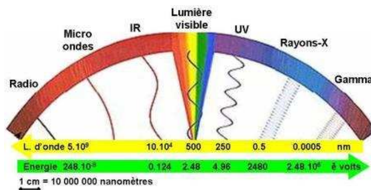
FIGURE I.4 – Spectre électromagnétique.
