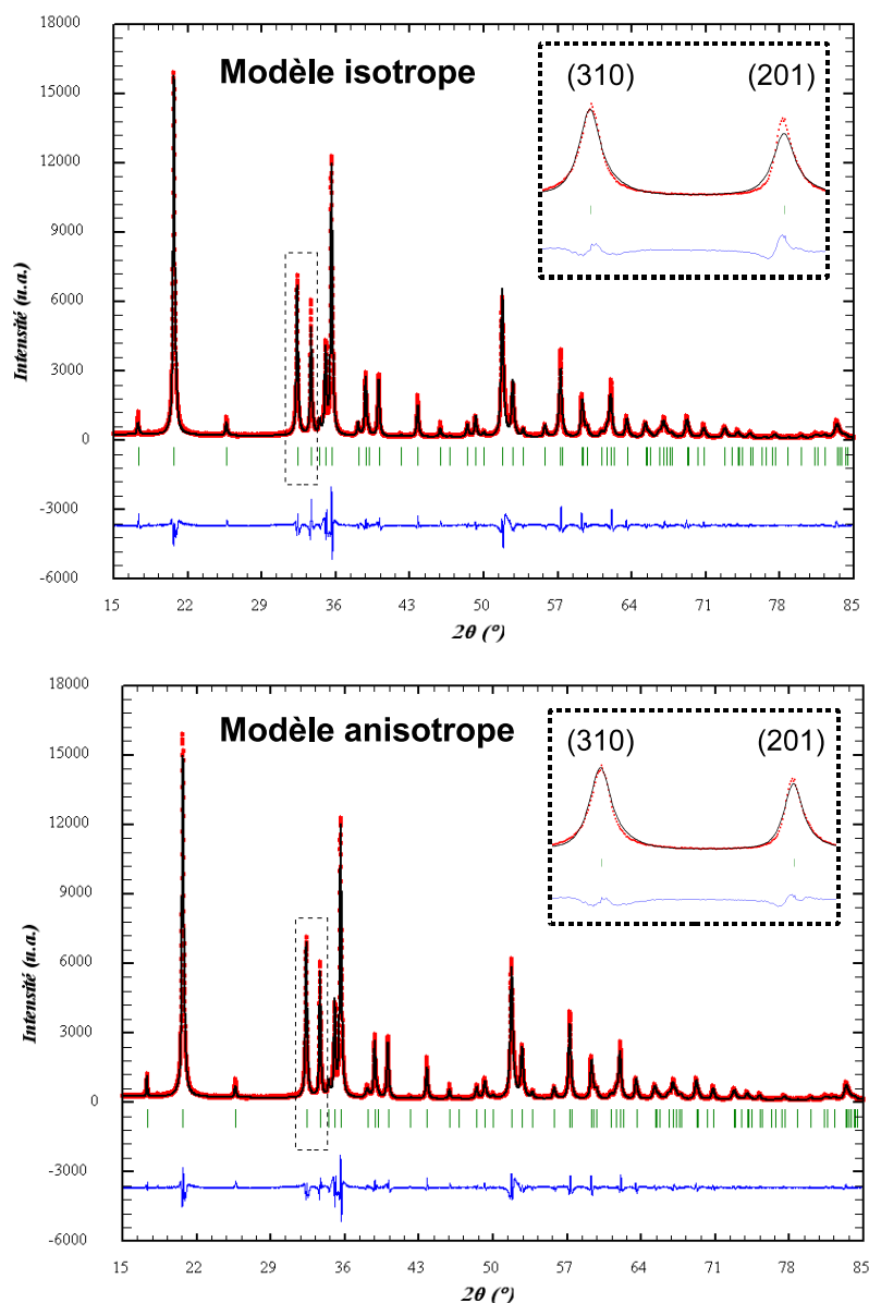
FIGURE III.4 – Diffractogrammes expérimentaux et calculés par affinements Le Bail (modèles isotrope et anisotrope) de la phase \text{Zn}(\text{OH})_{2-x}\text{F}_x synthétisée à pH égal à 6 (en rouge le diffractogramme observé, en noir le diffractogramme calculé et en bleu la différence).
