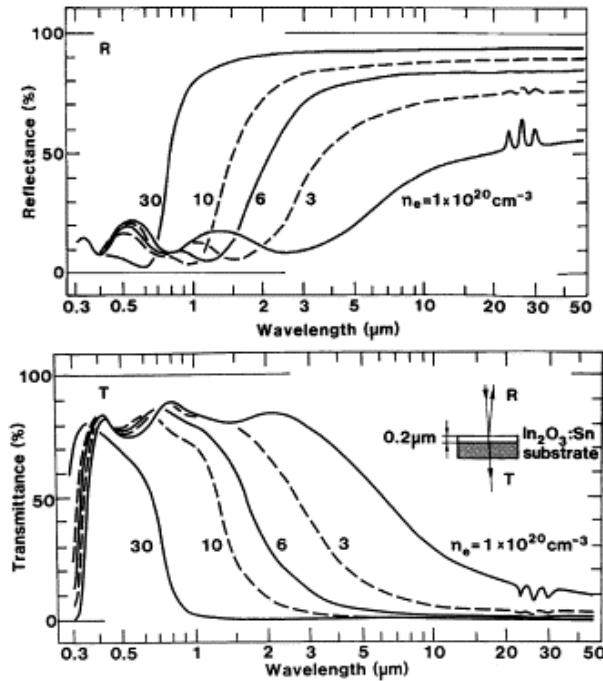
FIGURE I.10 – Réflectivité et transmittance de films d'ITO ( \text{In}_2\text{O}_3 : \text{Sn} ). Les courbes sont présentées pour différentes densités de porteurs. [38].
