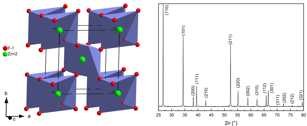
FIGURE III.1 – Structure cristallographique du fluorure \text{ZnF}_2 (gauche) et diffractogramme des rayons X correspondant (droite) sur lequel les indices de Miller des raies de diffraction sont indiqués.
