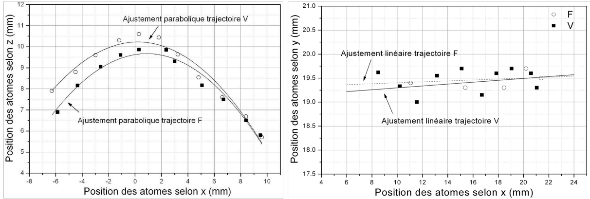
FIG. 3.15 : Trajectoires des deux nuages d'atomes au niveau de la zone interférométrique pour les deux nuages issus des sources F et V : à gauche dans le plan vertical ( OXZ ) et à droite dans le plan horizontal ( OXY ).
