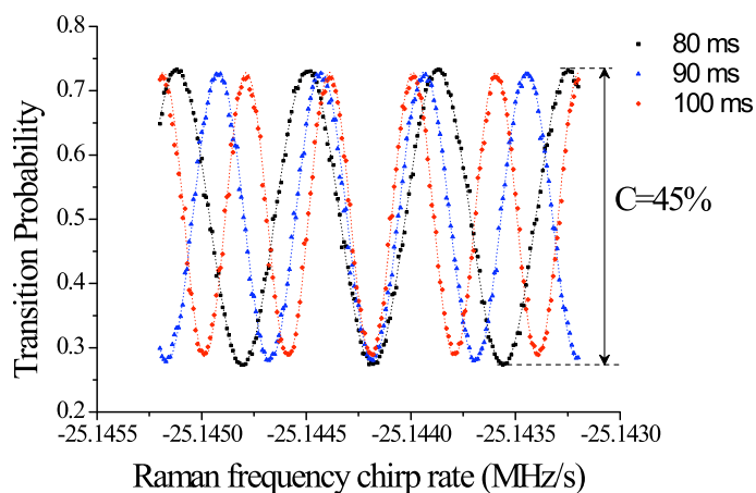
FIG. 4.6 : Interférogrammes réalisés en changeant la rampe de fréquence appliquée sur la différence de fréquence entre les faisceaux lasers Raman.
