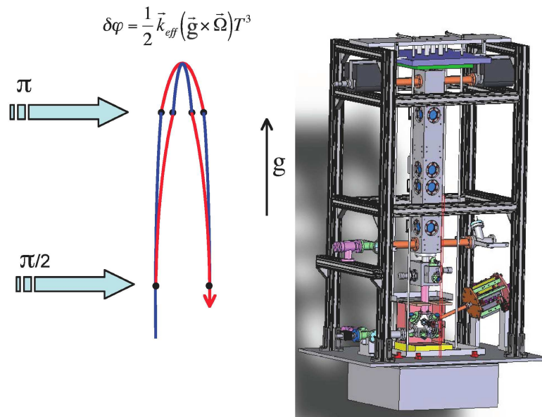
FIG. 5.2 : Schéma du nouveau gyromètre à quatre impulsions.
