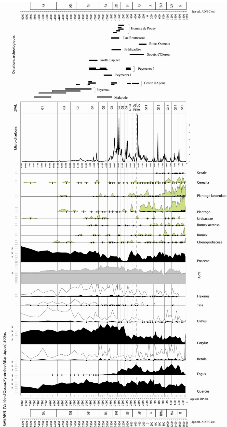
Figure 195 : Diagramme palynologique de la tourbière de Gabarn, 300 m (vallée d'Ossau, Pyrénées-Atlantiques) 300m. (GALOP 2006).
