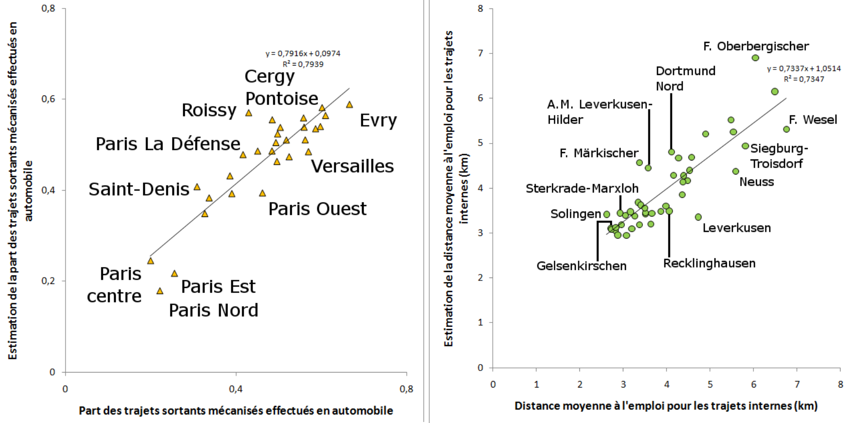
FIGURE 6.8 – Modèles linéaires liant un attribut de mobilité quotidienne et des indicateurs socio-économiques, géographiques et morphologiques. Gauche : part des trajets sortants réalisés en automobile (Ile-de-France). Droite : distance moyenne à l'emploi pour les trajets internes (Rhin-Ruhr).
