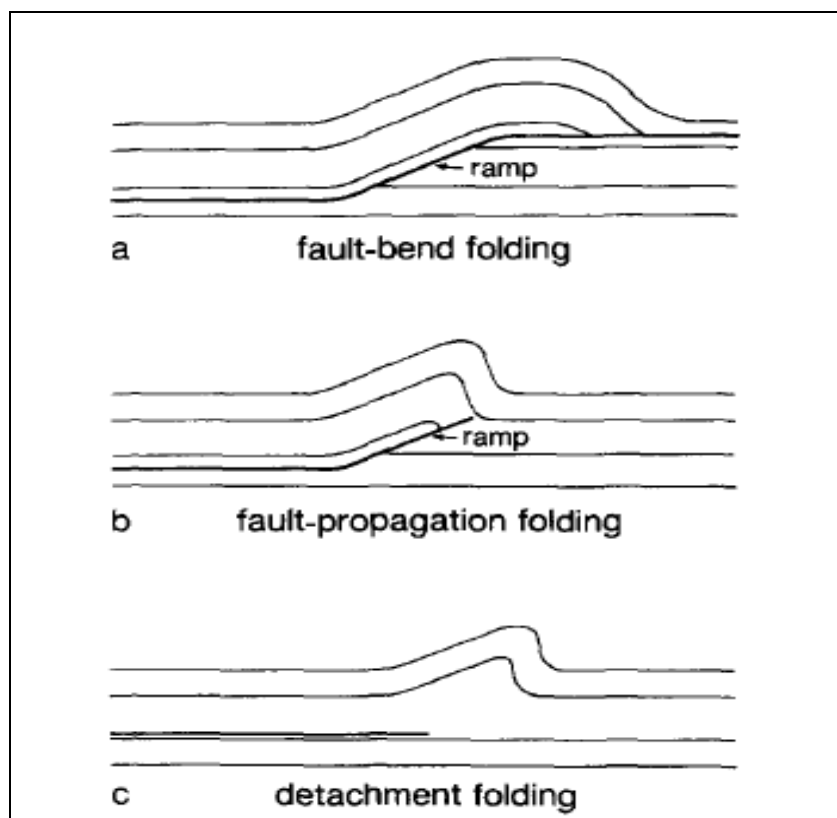
Figure 3: Les trois principaux types d'interactions pli/faille (d'après Suppe, 1983 ; 1985 ; Jamison, 1987 et Mercier et al., 1996).
