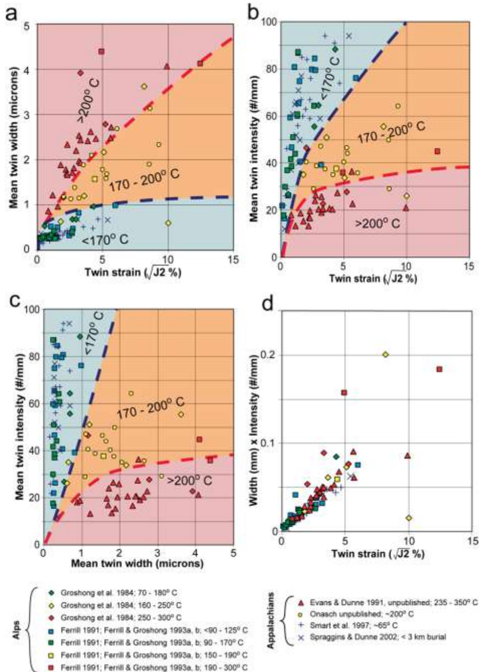
Figure 11: Graphiques des caractéristiques du maclage, à partir d'échantillons des Alpes et Appalaches. Les codes de couleur sont en fonction de la température de déformation déduite du maximum d'enfouissement ou des indicateurs métamorphiques. (a) Épaisseur moyenne des macles versus déformation par maclage, (b) densité de maclage versus déformation par maclage, (c) densité de maclage versus épaisseur moyenne des macles, (d) produit de l'épaisseur moyenne des macles et de densité de maclage (rapport cristaux maclés par cristaux non maclés) versus la déformation par maclage. Points incluant des données du tableau 1 de Ferrill (1991), Spraggins et Dunne (2002; données brutes), et Smart et al. (1997; données brutes). Des données microthermométriques non publiées d'inclusions fluides de M.A. Evans ont été utilisées pour contraindre les 65^\circ\text{C} , la température des échantillons de Smart et al. (1997) et la température de 235^\circ\text{C} définie à partir des données d'Evans et Dunne (1991). Les lignes rouges et bleues séparent les domaines de données caractérisées par la déformation à la température de 170 , 170-200 , et 200^\circ\text{C} . D'après Ferrill et al. (2004).
