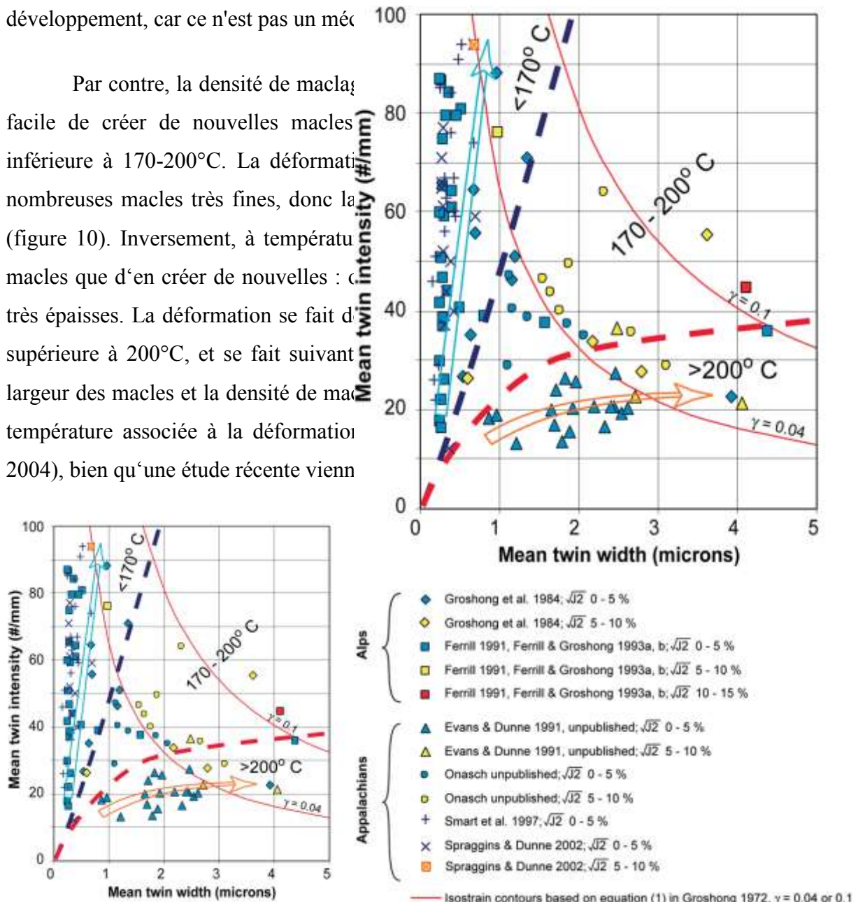
Figure 10: Graphique de l'intensité moyenne de macles versus l'épaisseur moyenne des plans de macle. Les couleurs sont en relation avec le degré de déformation. Les flèches orange et bleue illustrent respectivement le sens d'augmentation de la déformation pour 200° et 170°. D'après Ferrill et al. (2004).
