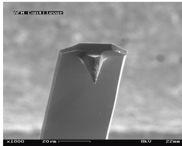
Figure 2 - 8 : Pointe sonde d'un AFM
