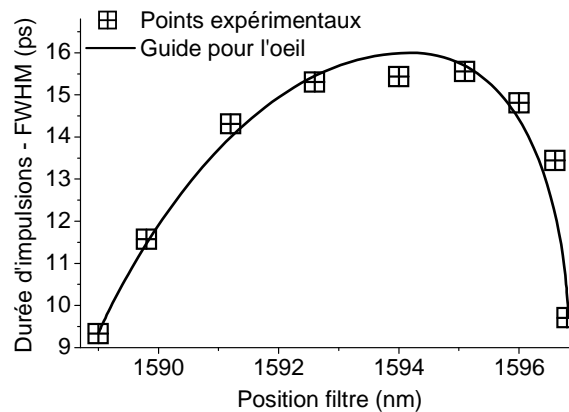
Figure 4 - 11 : Durée d'impulsions (ajustements gaussiens) en fonction de la position du filtre
