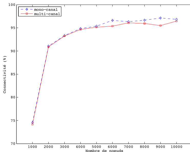
Figure 3.4. Impact de la cardinalité sur la connectivité de la structure de clusters
