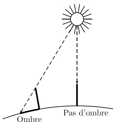
Figure 5 : Dessin prototypique d'élèves à qui l'on demande d'expliquer pourquoi au solstice d'été deux gnomons ne projettent pas la même ombre en deux endroits différents de la Terre situés le long du même méridien (Merle 1994, Farges & al. 2002, Ducourant 2007).
