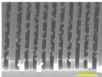
Figure 4.7 – Illustration de la formation de résidus après gravure du matériau hybride avec un masque en TiN et remise à l'air pendant 48 h.
