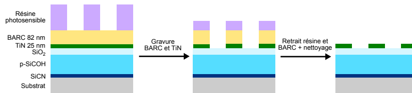
Figure 2.24 – Schéma des étapes de gravure du BARC et du TiN et du retrait résine et BARC (technologie 45 nm).
