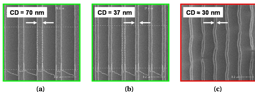
Figure 3.10 – Image en vue de dessus du masque en TiN après une sur-dose lors de l'exposition de la résine et une sur-gravure : (a) zone aux dimensions relâchées; (b) largeur minimale mesurée et (c) zone où les lignes ne sont plus continues.
