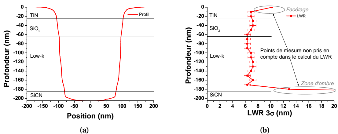
Figure 2.23 – (a) Profil d'une tranchée après gravure d'un niveau de métal et (b) mesures de LWR en fonction de la profondeur de la tranchée.
