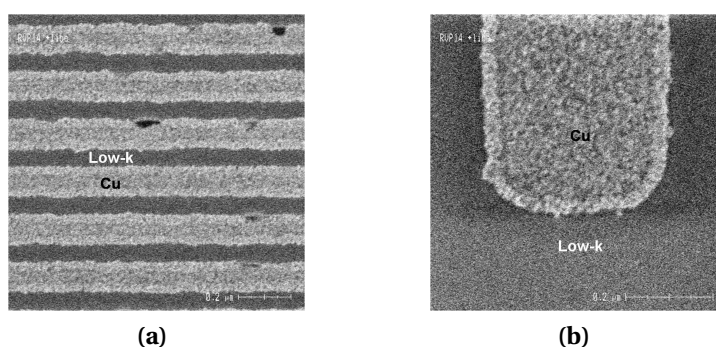
Figure 4.24 – Images au CD-SEM de lignes de cuivre après retrait des porogènes, avec purge en hélium avant le procédé.
