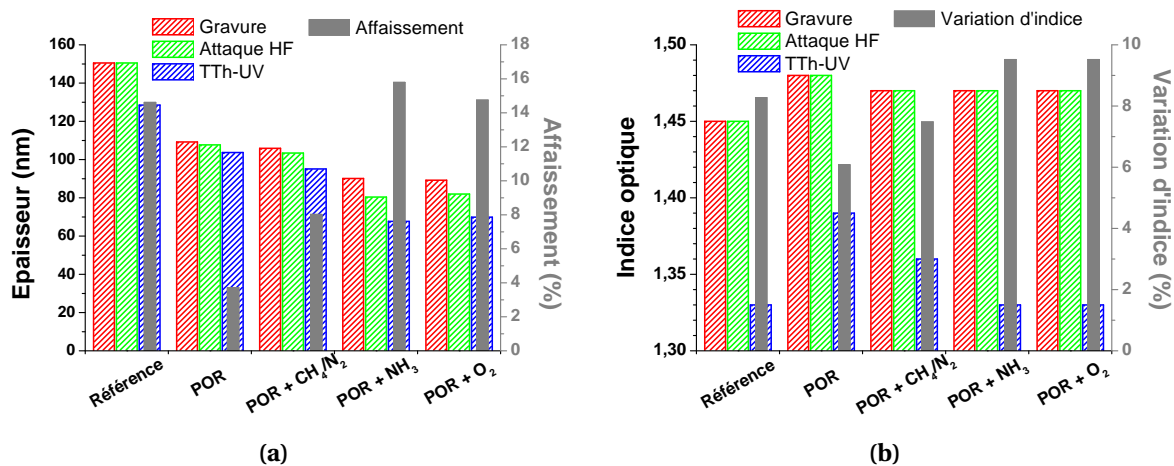
Figure 4.13 – (a) Épaisseur et (b) indice optique du matériau hybride après procédés plasma, attaque HF et recuit thermique assisté par UV.
