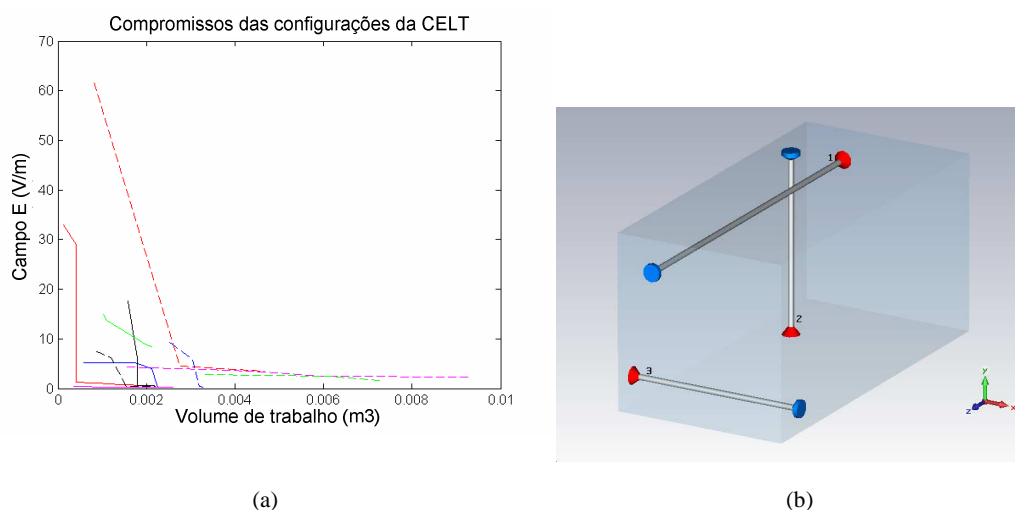
Figura 81 - Otimização híbrida da CELT protótipo (a) Fronteiras Pareto (b) melhor configuração de linhas de transmissão.
