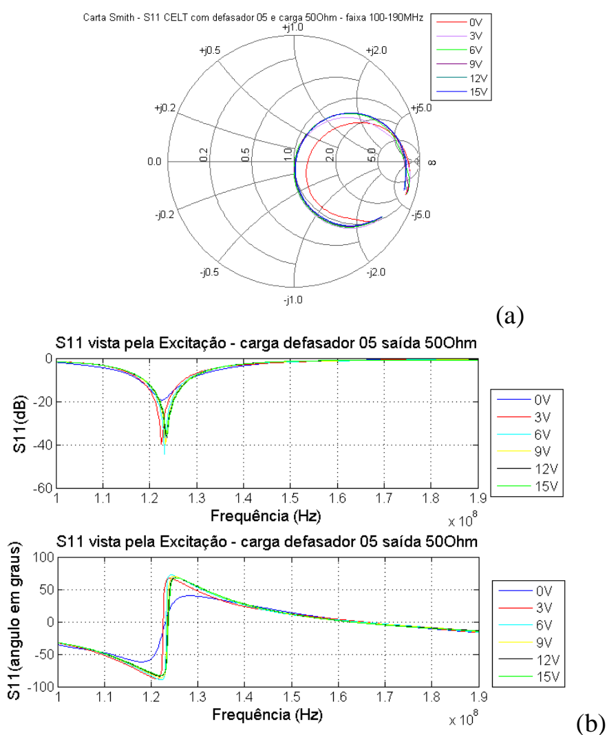
Figura 69 - Caracterização da câmara com defasador SO-05 na saída e carga 50 Ω (100MHz-190MHz) (a) Carta de Smith (b) S11 Módulo e Ângulo
