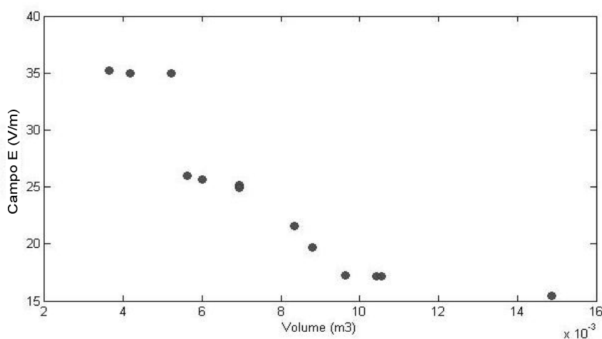
Figura 78 - Compromisso entre volume de trabalho e campo E.
