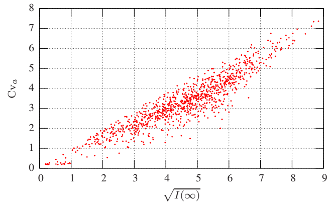
FIG. 4.11: Mesure de la variabilité du trafic dans le cas de la superposition de 2 sources ON-OFF hétérogènes. En abscisse, il s'agit de la racine carrée de la limite à l'infini de l'indice de dispersion calculée à l'aide des coefficients de variation des trafics incidents. En ordonnée, il s'agit du coefficient de variation du trafic agrégé mesuré par simulation.
