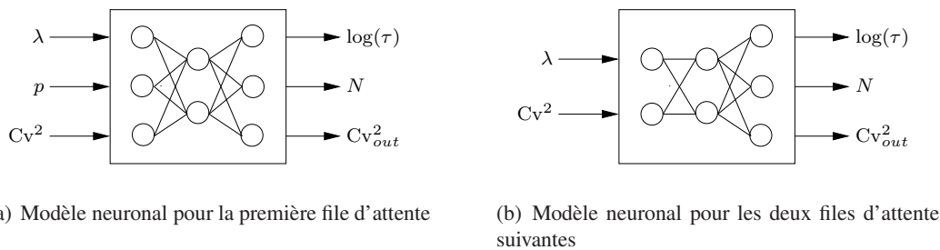
FIG. 5.2: Entrées et sorties des réseaux de neurones pour l'estimation de la QoS dans 3 files d'attente en série.
