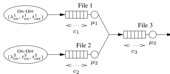
FIG. 5.8: Deux files alimentées deux sources ON-OFF hétérogènes, s'agrégeant dans une troisième file
