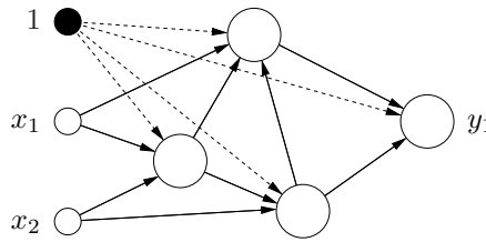
FIG. 2.3: Un exemple de réseau feed-forward .
