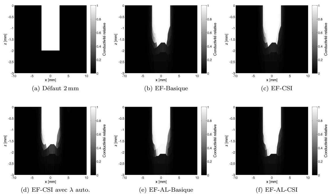
FIG. H.3 – Reconstructions pour le défaut de 2 mm
