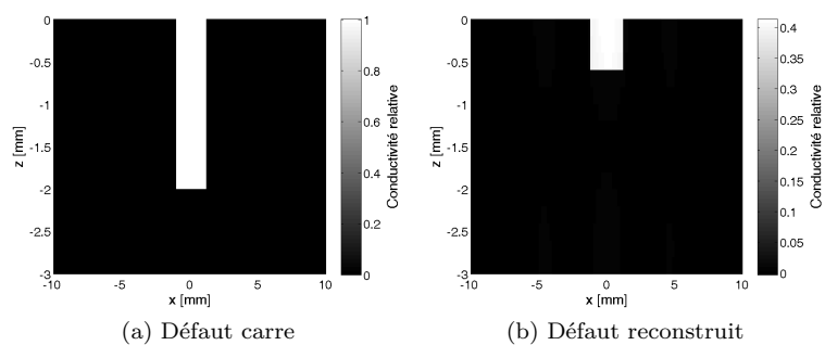
FIG. G.4 – Reconnstructions avec la méthode EDF-EPM pour le défaut carré
