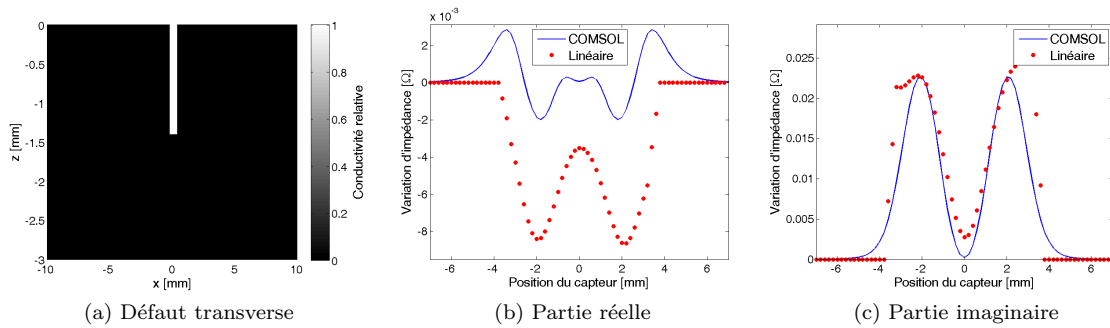
FIG. A.4 – Défaut et données simulées pour un défaut transverse de 1.4 mm
