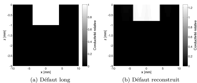
FIG. G.3 – Reconnstructions avec la méthode EDF-EPM pour le défaut long
