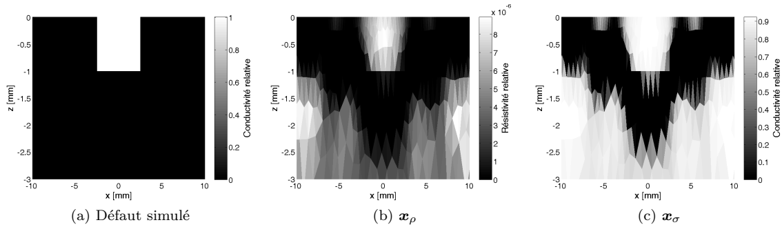
FIG. I.6 – Reconstructions pour la méthode EF-CI-Basique pour le défaut de 1 mm de profondeur avec régularisation sur x_\rho
