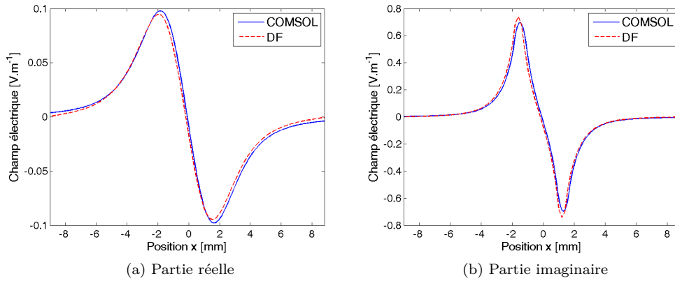
FIG. III.4 – Comparaisons du champ électrique sur la ligne horizontale à l'altitude z = 0,5 mm : parties réelle (a) et imaginaire (b)
