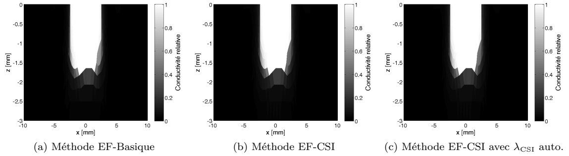
FIG. VIII.19 – Comparaison entre les méthodes de reconstruction pour le défaut de 2 mm de profondeur avec le même \lambda_{CSI} final
