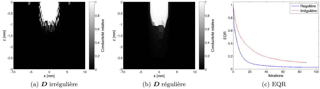
FIG. VIII.6 – Effet de la matrice D sur la reconstruction par EF-Basique pour le défaut de 1 mm de profondeur
