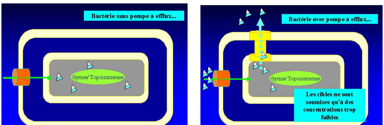
Figure 6. Resistance aux fluoroquinolones par mécanisme de rejet actif de la molécule (efflux).
