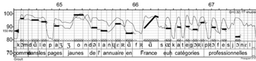
FIGURE 3.6 – Prosogramme (extrait de [Mertens 04])
