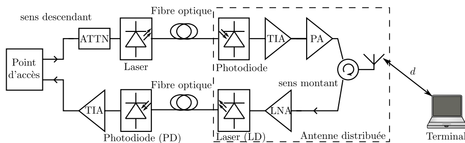
FIGURE 2.7 – Présentation de l'architecture bidirectionnelle.
