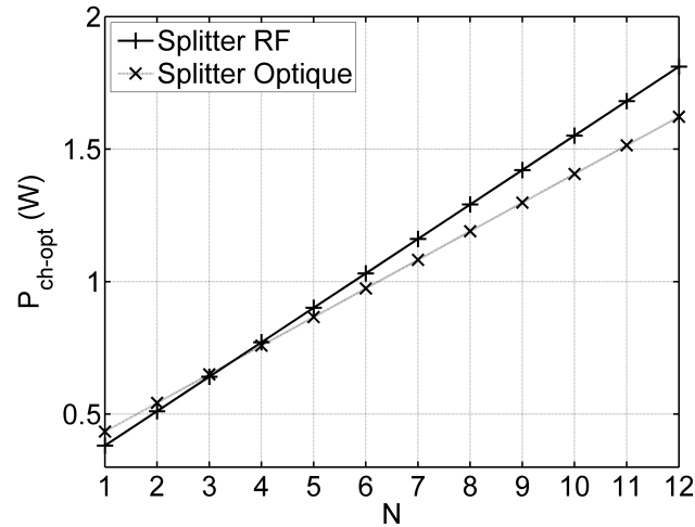
FIGURE 2.10 – Puissance consommée par l’ensemble de la chaîne optique en fonction du nombre d’antennes distribuées pour une puissance totale rayonnée de 14 dBm.
