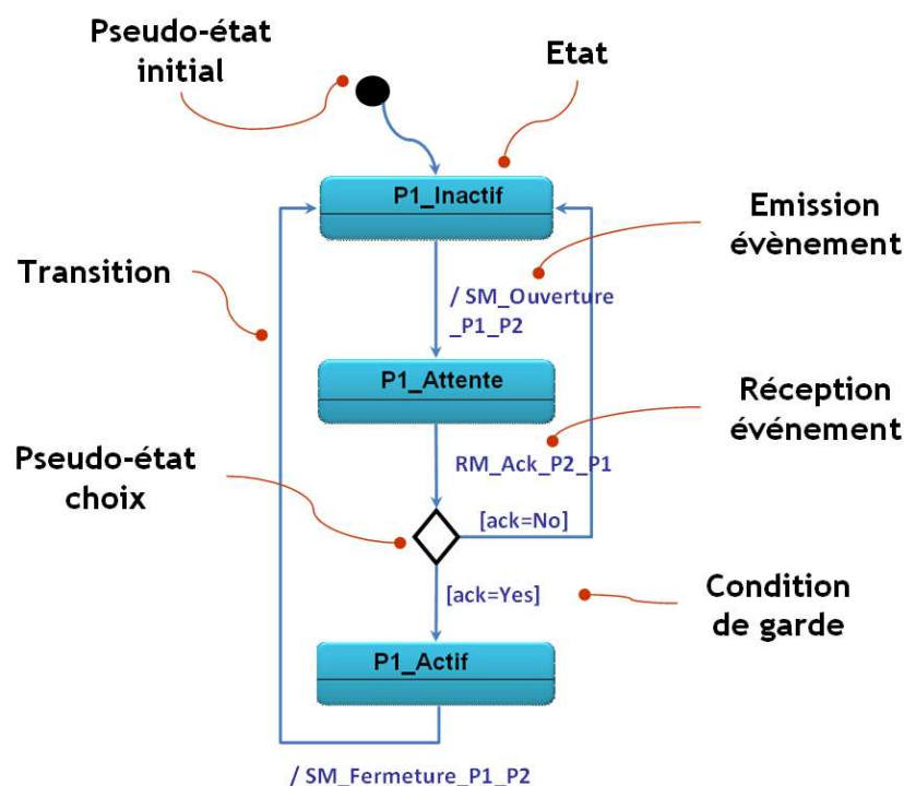
Figure 3.41: Exemple de machine d'états UML
