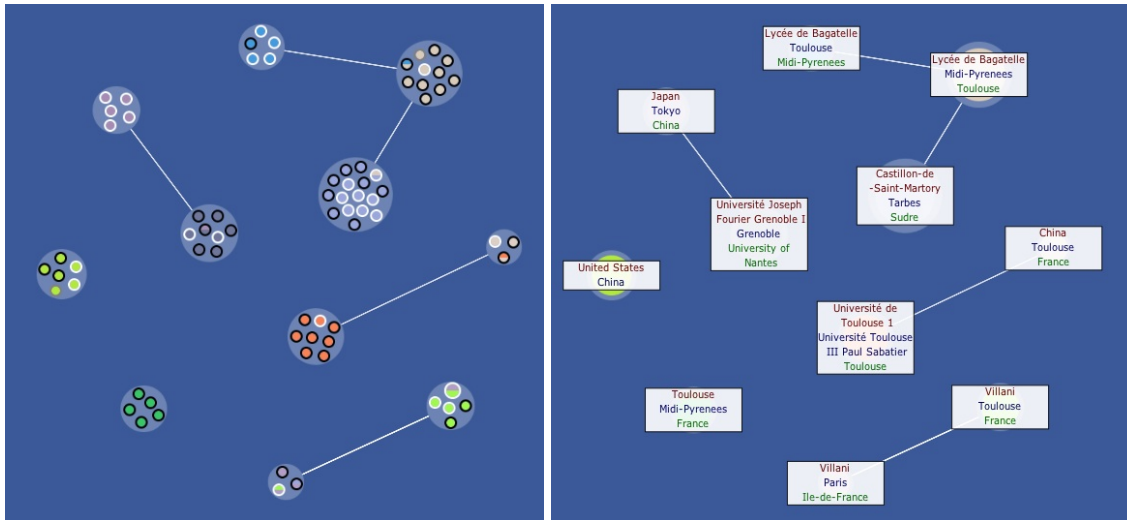
FIGURE 4.10 – Captures d’écran de l’interface de l’application Facebook. A gauche, la vue présentant le détail par individu. A droite, la vue par communautés seulement. Les 3 mots clés les plus pertinents sont associés à chaque communauté.
