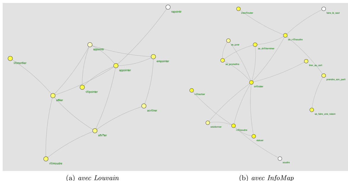
FIGURE 3.5 – Exemple de communautés trouvées avec des algorithmes à communautés relatives, dont la topologie interne ne semble pas très pertinente intuitivement. Ces communautés ont été trouvées dans un graphe de terrain avec, de gauche à droite, l’algorithme Louvain et l’algorithme InfoMap.
