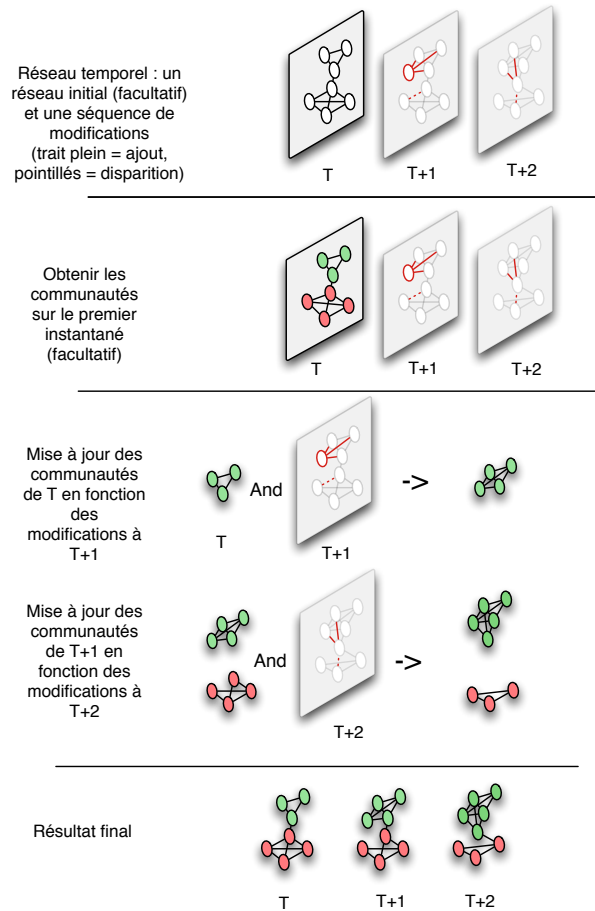
FIGURE 2.15 – Illustration de l'approche par détection de communautés sur des réseaux temporels.
