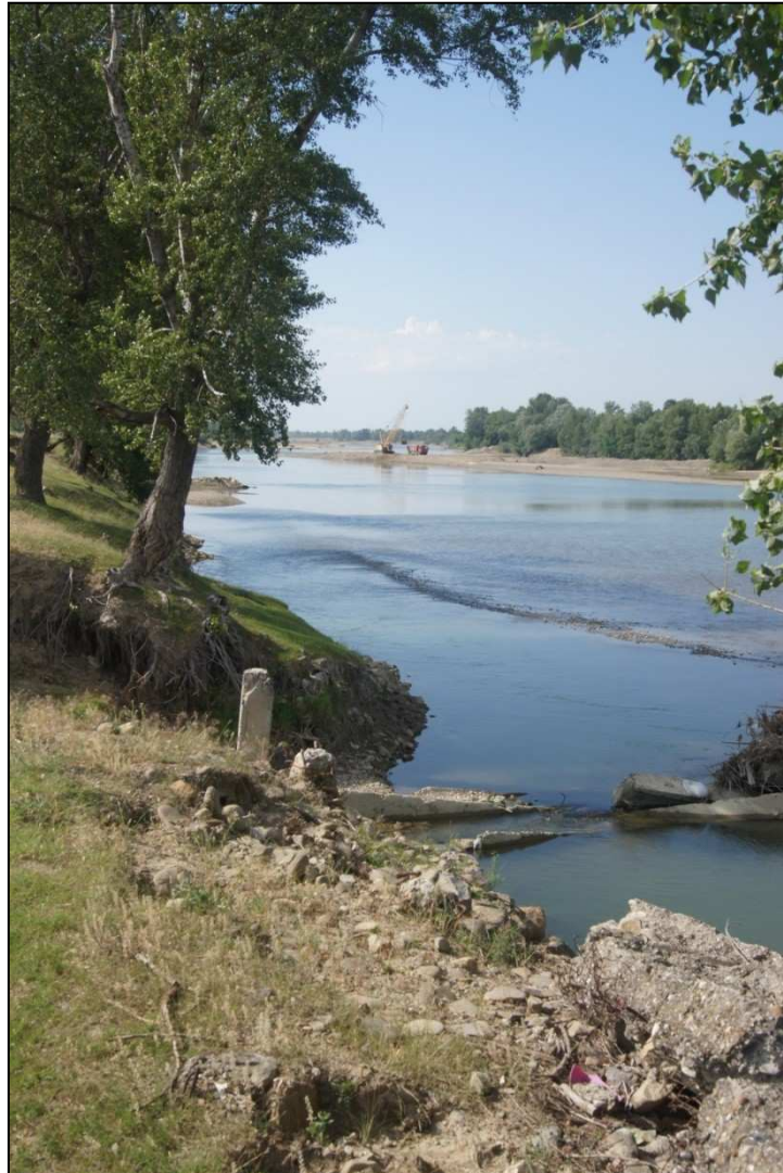
Figure 3- 56: Aménagement des berges pour lutter contre l'érosion latérale sur le Siret inférieur entre les villages de Biliеști et de Suraia, vu vers l'amont. Au premier plan, aménagements détruits et à l'abandon ; à l'arrière-plan, une excavatrice dans le lit mineur (Photographie: F. Salit, juin 2012) (Localisation Figure 3- 48)
