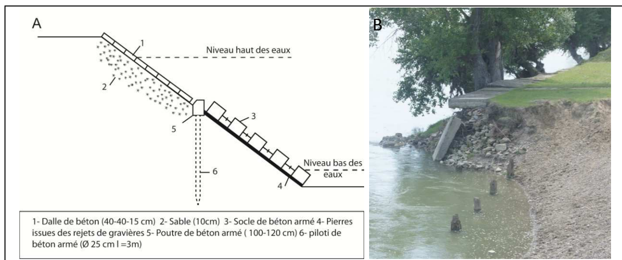
Figure 2- 30: A – Schéma de travaux de protection des berges (traduit d'après Manoliu, 1973). B – Ouvrages de protection des berges sur le Siret inférieur entre Biliști et Suraia (F. Salit, juin 2012)
