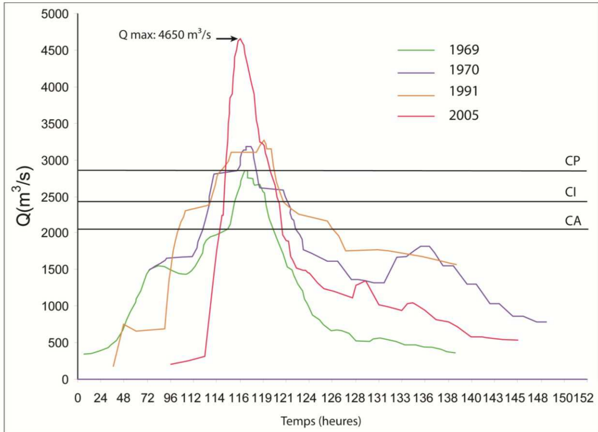
Figure 3- 16: Hydrogramme comparé des crues les plus importantes du Siret à la station de Lungoci de 1969 à 2005 (Source : INHGA)
