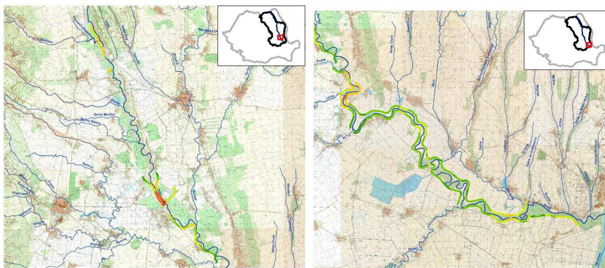
Figure 3- 52: Localisation des digues provoquant une accélération des vitesses d'écoulement sur le Siret inférieur pour un événement d'intensité égale à la crue de 2005. De l'amont (à gauche) à l'aval (à droite) Vert : 0-1 m/s ; Vert clair : 1-1,5 m/s ; Orange : 1,5-2 m/s ; Rouge : +2,5 m/s (d'après Ministerul Mediului, 2009a)
