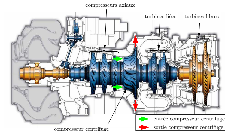
Fig 1.4: Exemple d'architecture Turbomeca
