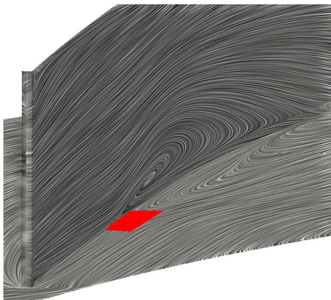
Fig 6.2: Prélèvement c_q = 1\% – Topologie stationnaire, avant décrochage.
