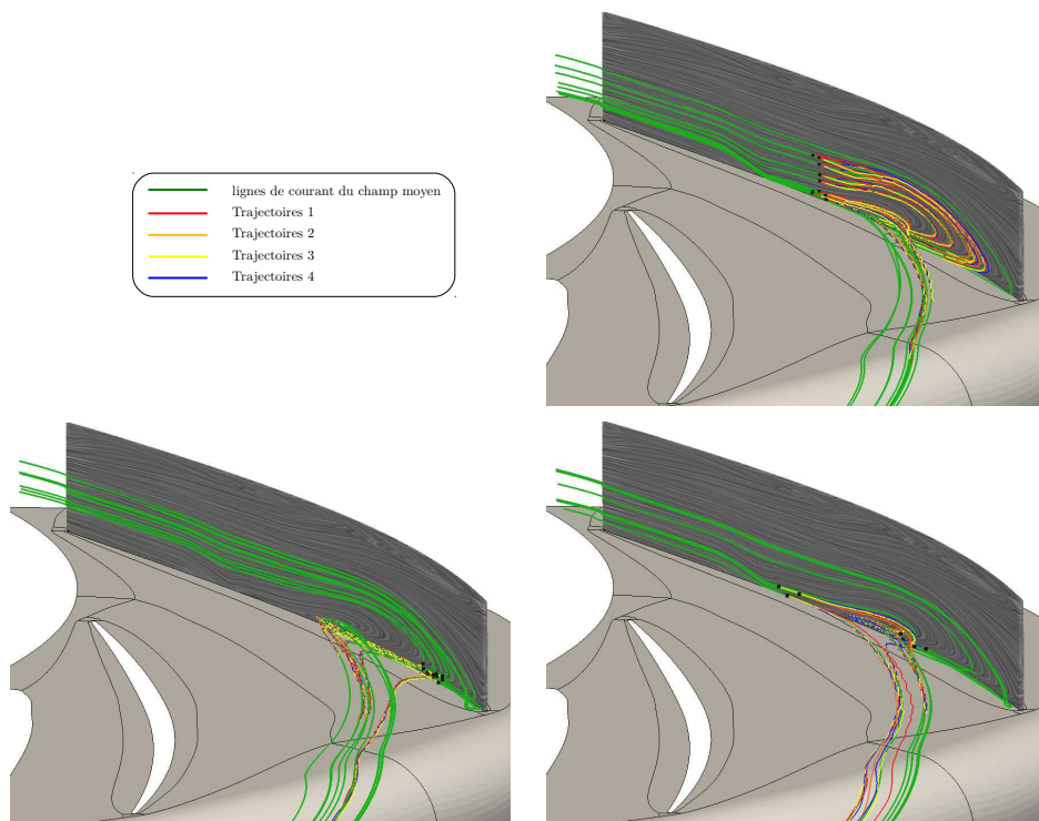
Fig 6.24: Comparaison de lignes de courant moyennes et de trajectoires de particules – Instationnaire proche pompage, c_q=1\%
