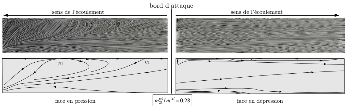
Fig 5.39: Spectre pariétal sur les faces en pression et en dépression des aubages du diffuseur – RANS, rendement max.
