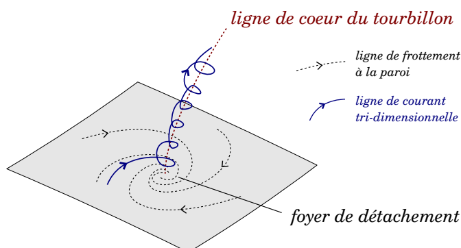
Fig 4.6: Tourbillon s'échappant d'un foyer de détachement
