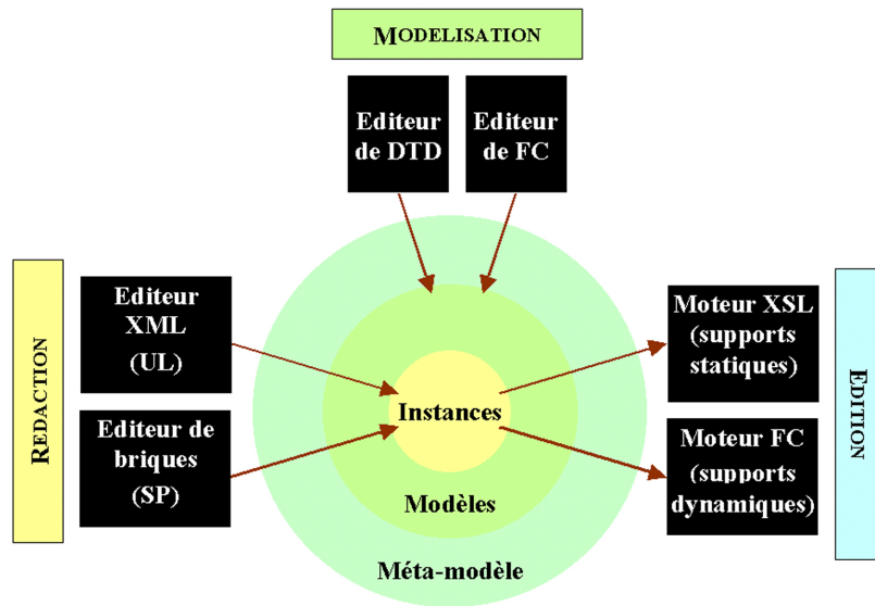
FIG.43 : Eléments d'architecture pour l'implémentation du méta-modèle SP/UL
