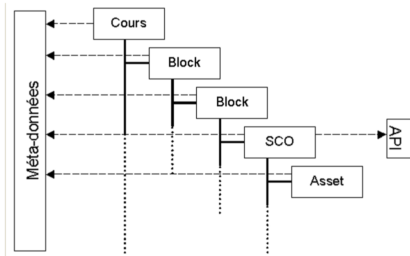
FIG.9 : Structuration des contenus dans SCORM
