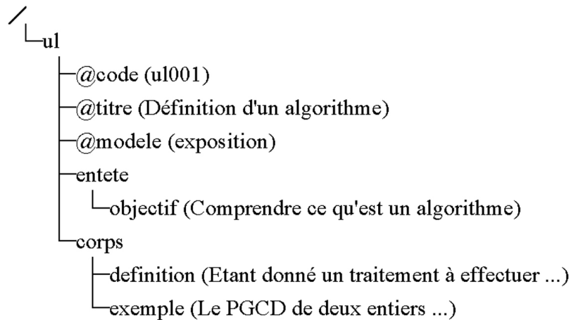
FIG.41 : exemple de représentation de document XML sous forme d'arbre
