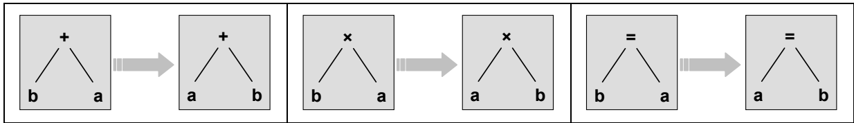
Figure 3-12 : Les règles de normalisation des arbres d'expression : la commutativité de l'addition, de la multiplication et de l'égalité.
