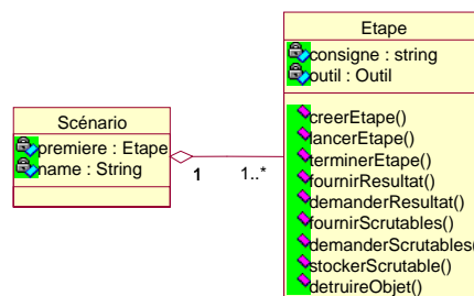
Figure 4.4 – Les classes pour un scénario
