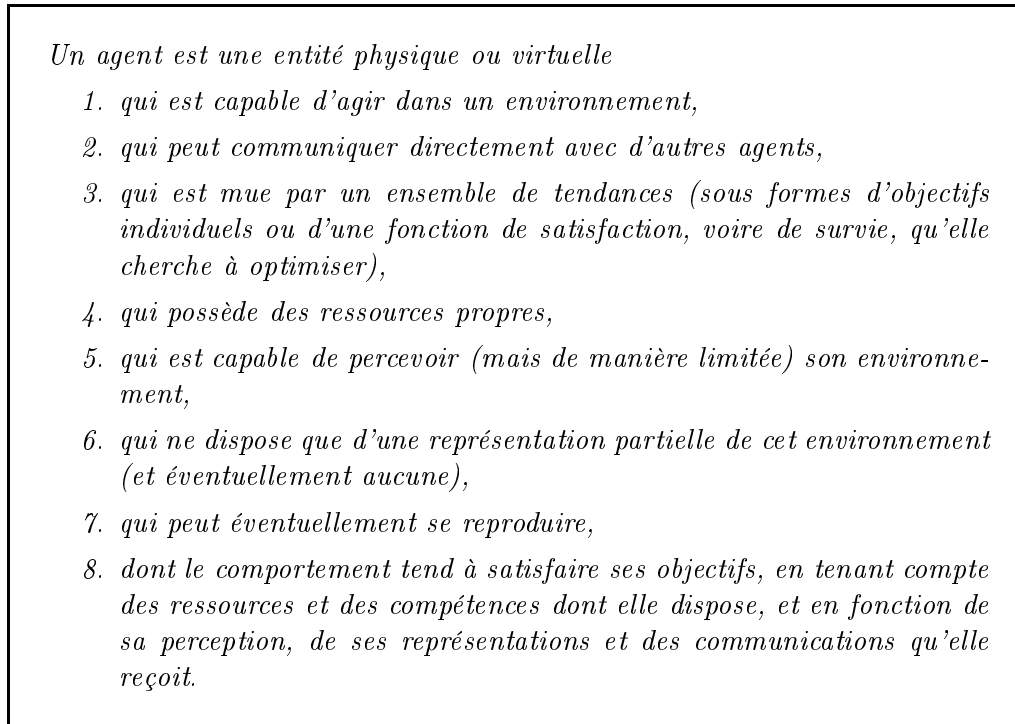
Figure 2.3 – Définition d'agent
