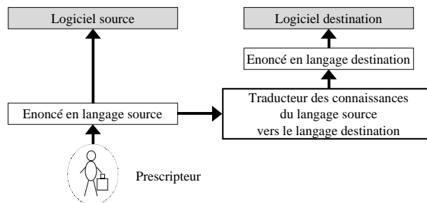
Figure 3.24 – Utilisation d'un traducteur spécifique.
