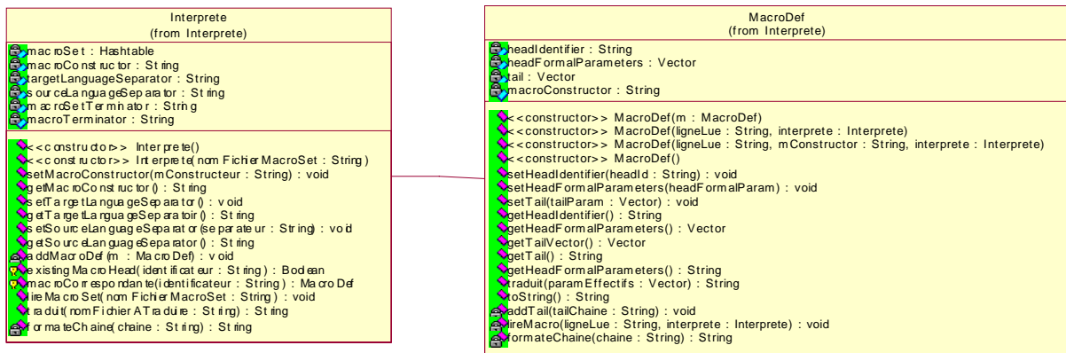
Figure 4.11 – Classes de l'interprète
