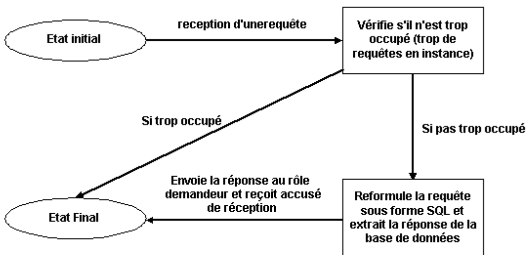
Figure 5.8 : Etats et transitions de r_SI (agent superviseur des interactions)
