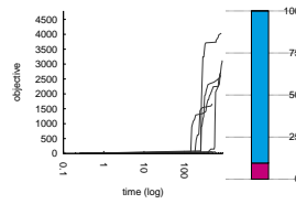
1.149 mario_mario_t_hard_1 with EBLNS
