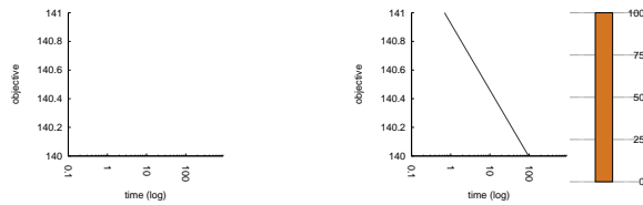
1.99 rcpsp_14 EBLNS
