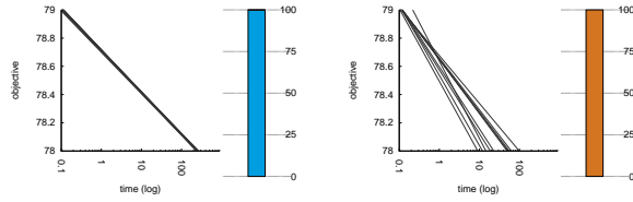
1.94 rcpsp_13 EBLNS
