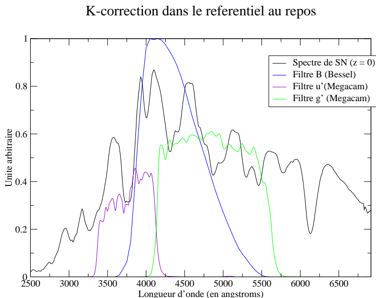
FIG. 4.3 – K-correction dans le référentiel au repos : on voit que le filtre B de Bessel choisi par convention pour l'estimateur de distance cosmologique, chevauche deux filtres effectifs de Megacam. Il faut donc estimer le flux qu'on aurait obtenu dans le filtre B à partir des flux mesurés dans les filtres u' et g'. De plus, dans le cas réel, on ne dispose que d'un seul spectre pris proche du maximum ; pour estimer la K-correction pour une phase quelconque p , on doit donc dans un premier temps chercher le spectre connu le plus analogue près du maximum et ensuite utiliser un spectre de référence de cette supernova connue proche de la phase p étudiée.
