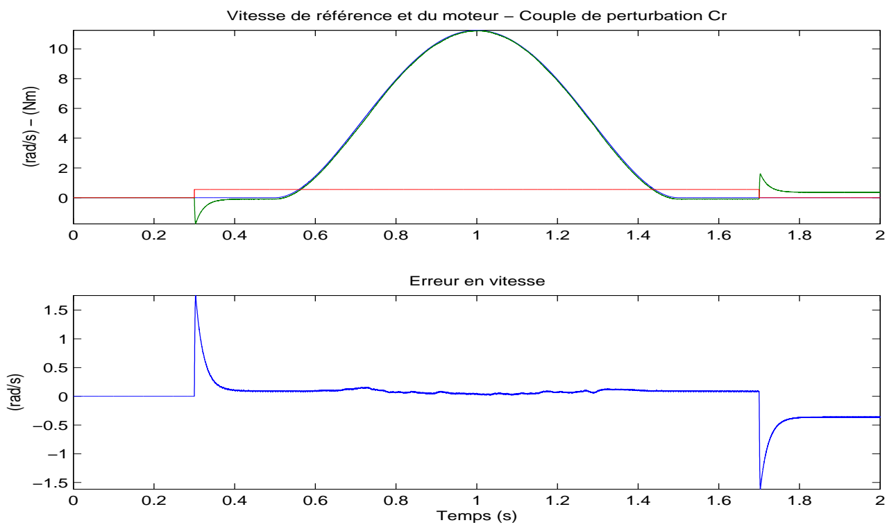
FIG. 5.4 – MG1 en vitesse - Vitesse - C_r = 0.55Nm - Simulations
