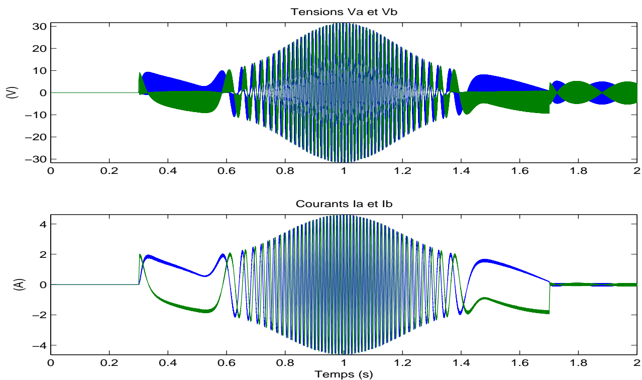
FIG. 5.5 – MG1 en vitesse - Tensions et courants - C_r = 0.55Nm - Simulations
