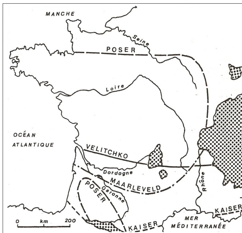
FIG. 2.21 – Limites méridionales du pergélisol du sud de l'Europe au cours du Dernier Maximum Pléiglaciaire selon différents auteurs [TEXIER (1996)]
