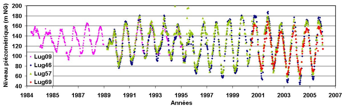
FIG. 3.36 – Piézométrie au droit du stockage de Lussagnet
