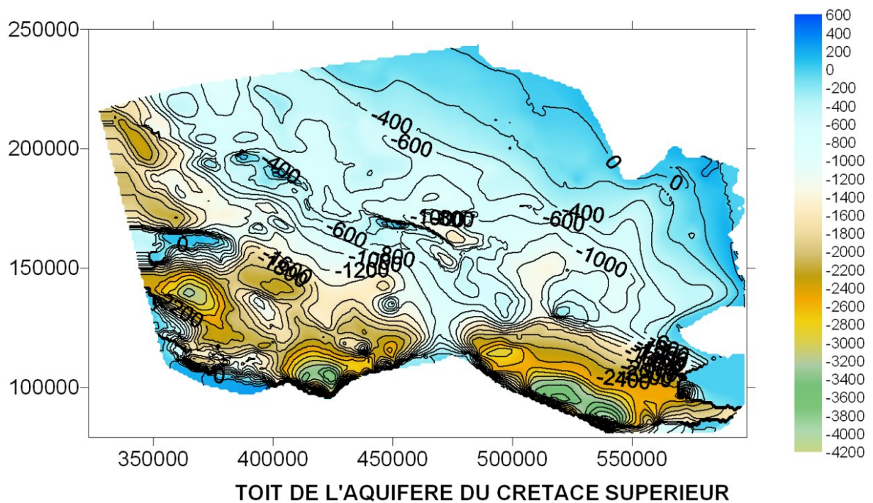
FIG. H.2 – Cartes du toit des aquifères du Paléocène et du Crétacé supérieur (en m NG)
