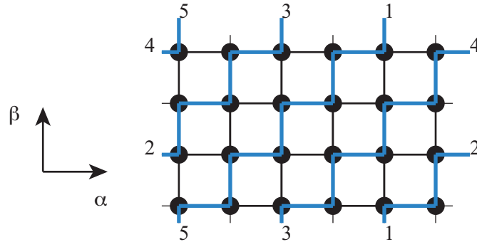
Fig. 3. Un cycle hamiltonien du tore à 6 \times 4 sommets.
