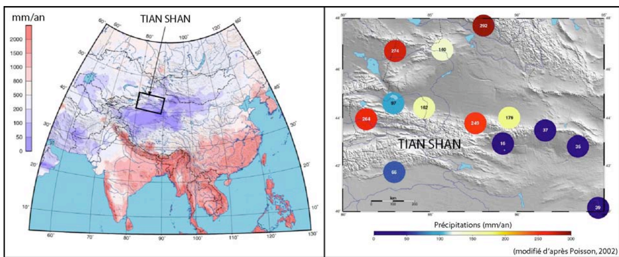
Fig.II. 5 : Précipitations annuelles A) en Asie (d'après Legates & Willmott, 1990) et B) au niveau du Tian Shan (données de l'U.C.A.R. : University Corporation for Atmospheric Research – Boulder, Colorado, USA)
