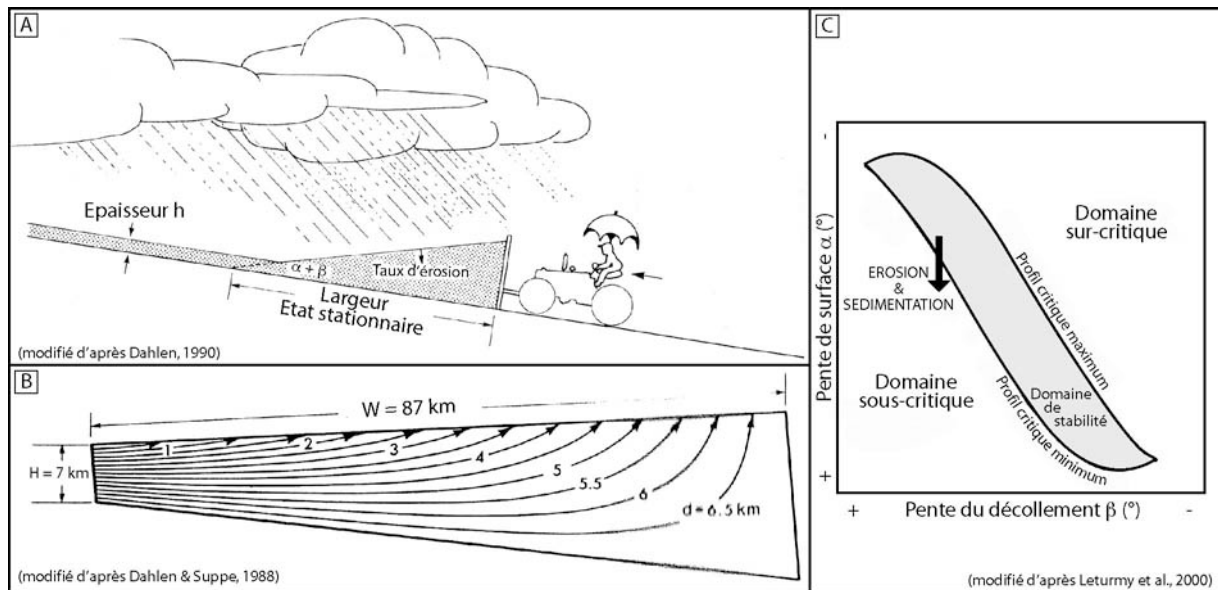
Fig.I. 13 : Erosion et modèle de prisme critique. A) Prisme critique ayant atteint un état d'équilibre dynamique entre le flux entrant et le flux sortant (d'après Dahlen, 1990). B) Modélisation des trajectoires des roches au sein du prisme de Taiwan (d'après Dahlen & Suppe, 1988). Considérant un flux en entrée de 500 \text{ km}^2/\text{Ma} , un taux d'érosion de 2,9 \text{ km}/\text{Ma} , une largeur de prisme égale à 87 \text{ km} , les trajectoires des roches dessinent des courbes dont la longueur dépend de la profondeur de l'échantillon. En moyenne, une roche typique réside 2 à 3 \text{ Ma} dans le prisme. C) Explication de l'effet de l'érosion sur la dynamique des prismes d'accrétion critique grâce au diagramme des domaines de stabilité (d'après Leturmy et al., 2000).
