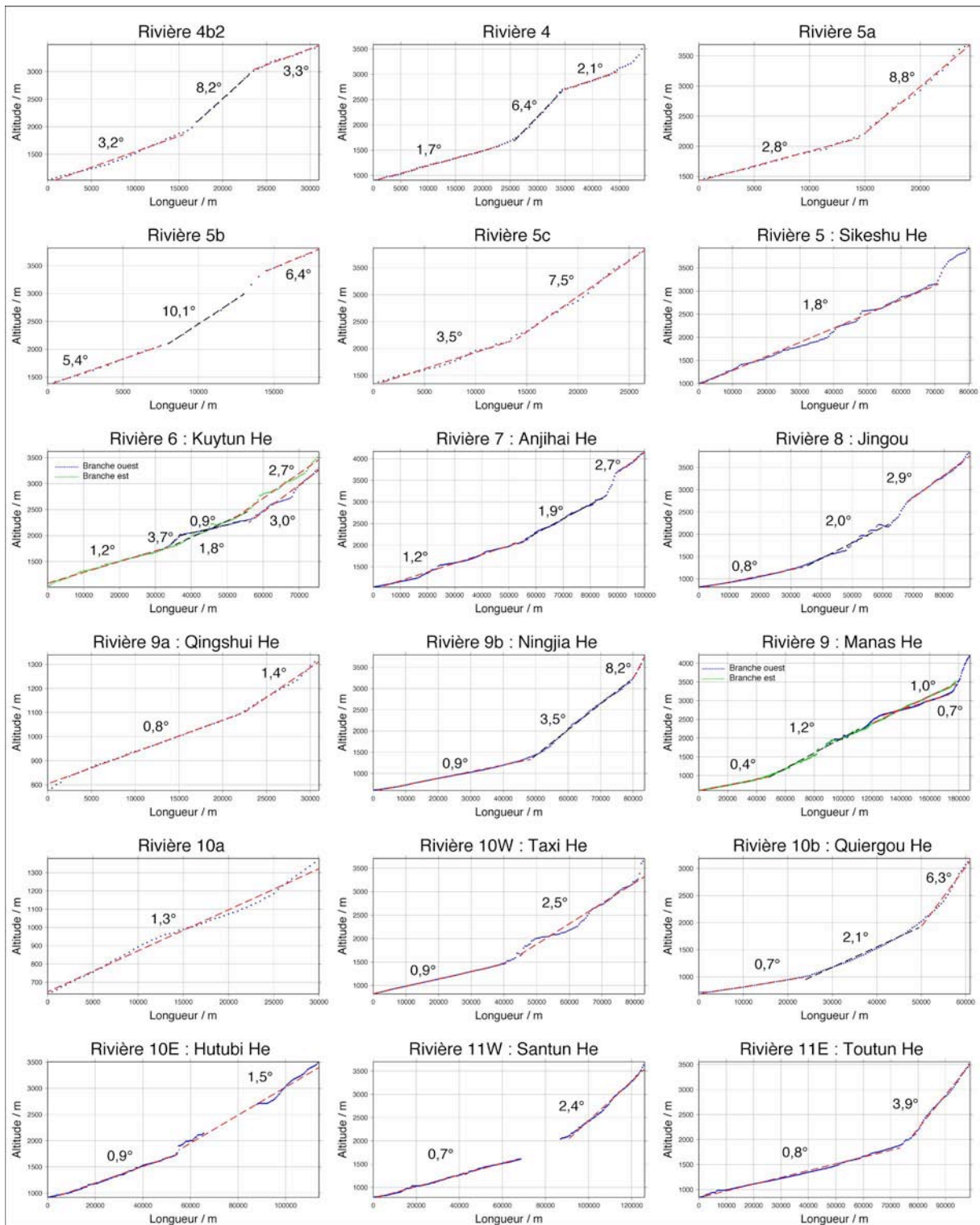
Fig.II. 28 : Profils « déroulés » des rivières du piémont nord du Tian Shan. Un profil déroulé correspond au profil « vrai » suivi par la rivière (par opposition à un profil projeté sur une direction quelconque). Les pentes du profil correspondent véritablement aux pentes d'écoulement des rivières. Noter la remarquable linéarité des segments fluviaux par portion de la chaîne dans laquelle ils s'écoulent. Les profils sont issus de MNT NASA-SRTM à 90 m filtrés à 500 m. Les pointillés de couleurs correspondent à la régression linéaire de chacune des portions du profil.
