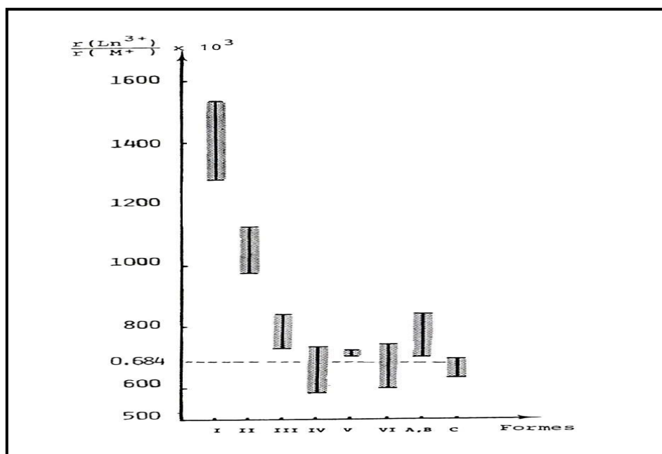
Figure I.26 : Représentations des domaines d'observation de différentes formes cristallines des phosphates \text{M}_2\text{O}.\text{Ln}_2\text{O}_3.4\text{P}_2\text{O}_5 (110).
