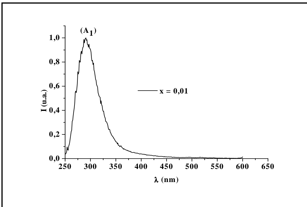
Figure IV-A8 : Spectre d'émission ( \lambda_{\text{exc.}} = 230 nm) du verre \text{Na}_{0,99}\text{Ag}_{0,01}\text{La}(\text{PO}_3)_4 à T = 300 K
