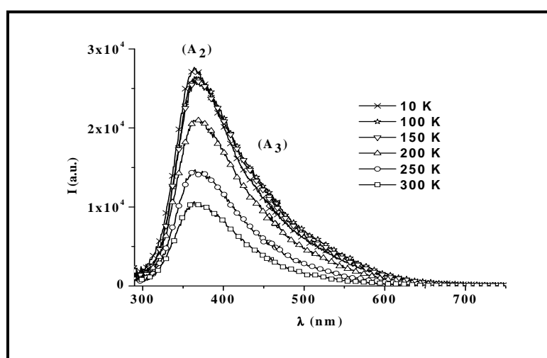
Figure IV-A20 : Evolution de l'intensité des émissions ( A_2 ) et ( A_3 ) en fonction de la température pour le verre de composition x = 0,5 , \lambda_{exc.} = 245 nm
