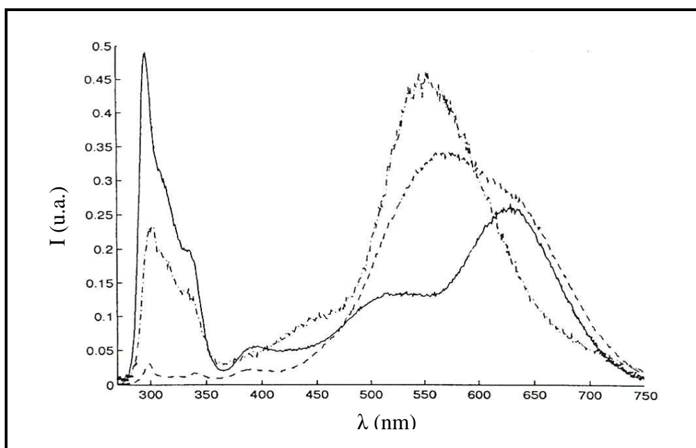
Figure I.15 : Spectres d'émission du cristal \text{SrF}_2 : \text{Ag}^+ irradiés après excitation à 221 nm. à T = 3 \text{ K} (---), T = 80 \text{ K} (---), T = 80 \text{ K} (—) après recuit du cristal irradié à 500 \text{ }^\circ\text{C} (58).
