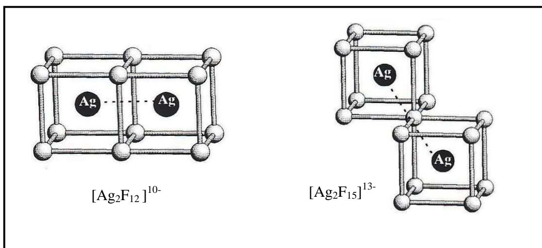
Figure I.13 : Les différents clusters présents dans \text{SrF}_2 : \text{Ag}^+ (52).
