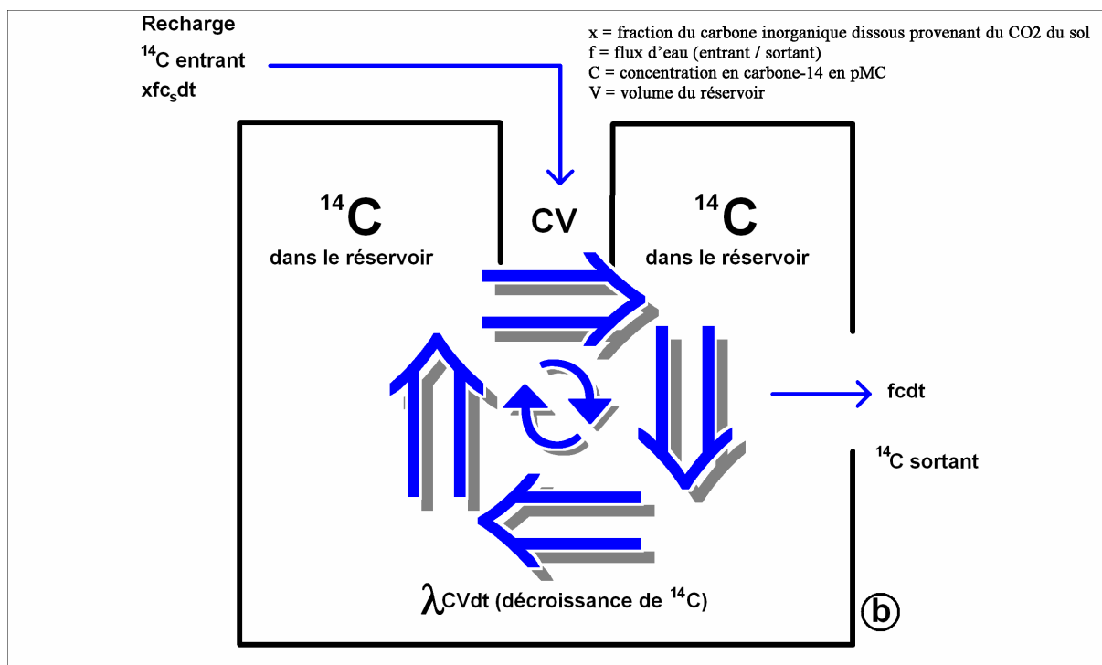
Figure 63. (a) Synthèse du CO 2 du sol de la zone d'étude et (b) Présentation schématique d'un réservoir non stratifié dans le cadre du modèle de mélange parfait
