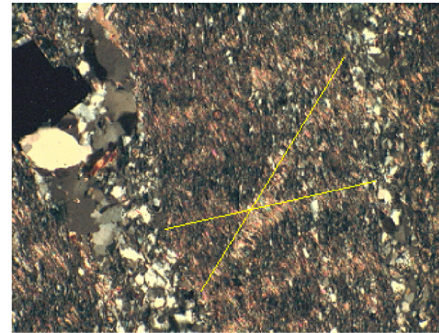
Figure 25. Ségrégation minéralogique au sein des métaarénites de Guéssigié (lumière polarisée)
