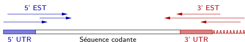
FIG. 2.2 – Les EST sont issus du séquençage partiel des extrémités d'un ARN mature, ici un ARN messager.
