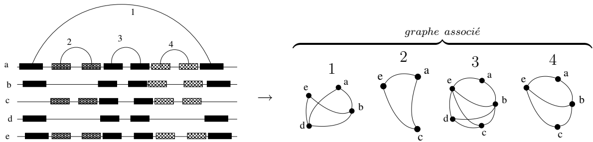
FIG. 3.13 – Graphe des tiges construit après les coreliements de cinq ARN de transfert.
