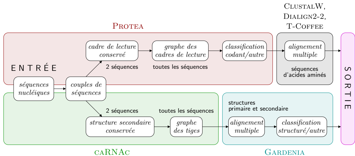
FIG. 4.1 – L'enchaînement des modules qui composent MAGNOLIA.
