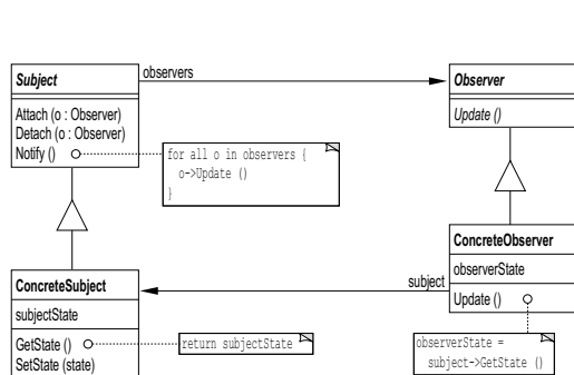
10.5a – Schéma de conception Observateur
