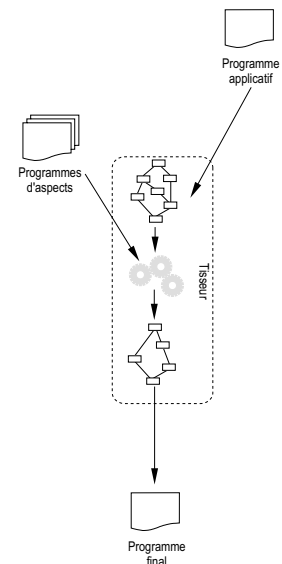
FIG. 7.8 – Principe du « tissage » des aspects
