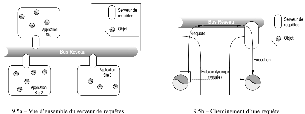
9.5a – Vue d'ensemble du serveur de requêtes
