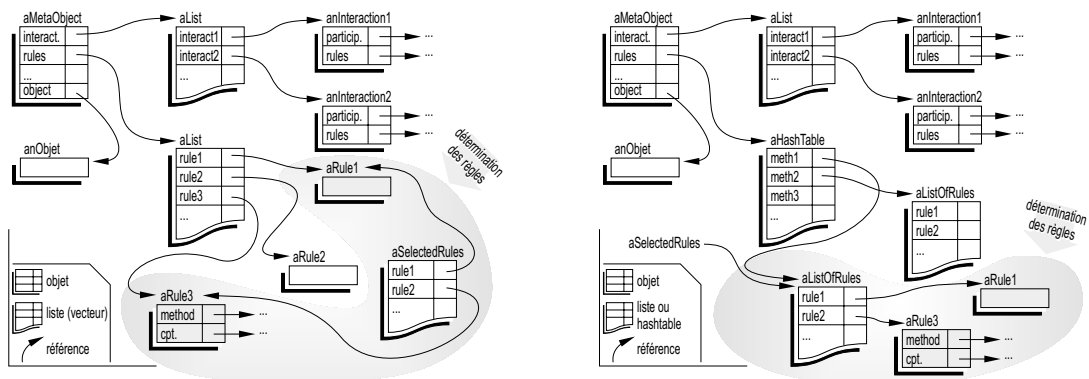
8.9a – Détermination des règles d'interaction à l'aide d'une liste
