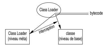
FIG. 7.7 – Principe de la liaison réflexive au chargement de classes
