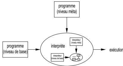
FIG. 7.5 – Principe de la liaison réflexive à l'exécution (tour réflexive)
