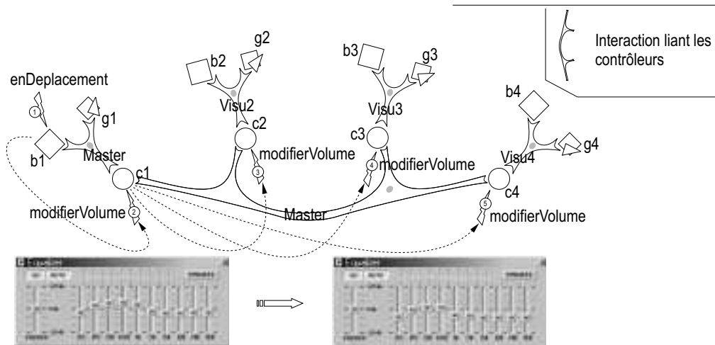
FIG. 4.2 – Envoi d'un message déclenchant l'exécution de plusieurs interactions en cascade
