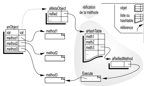
FIG. 9.4 – Enregistrement des instances des méthodes réifiées
