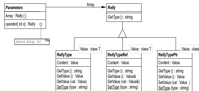
FIG. 9.3 – Schéma UML des classes réifiant les paramètres
