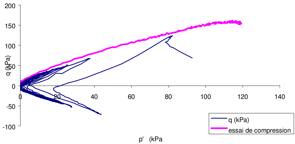
Chemin de contraintes limon ' A' 6v2 - w_c = 17,5\% , s'_{vo} = 100 kPa
