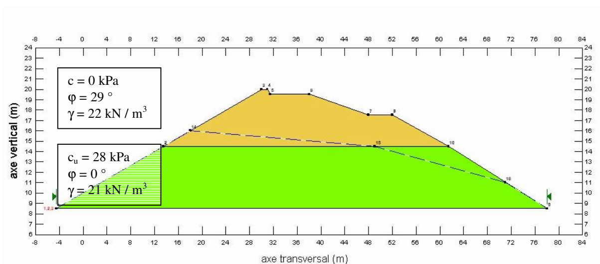
figure 2-28, modèle de section établi à partir du pénétrogramme 20
