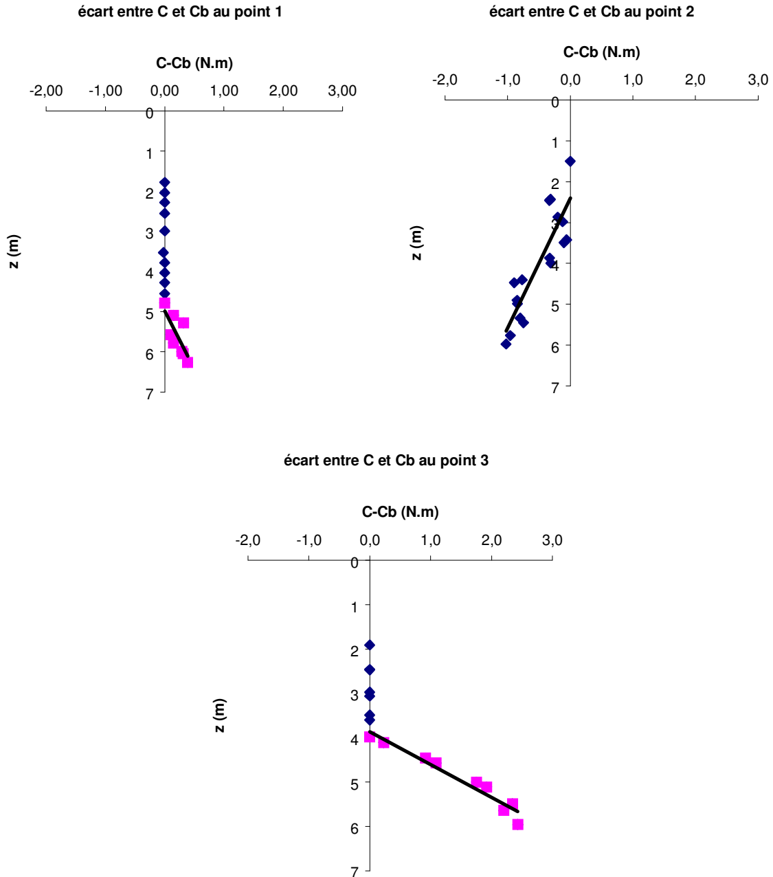
figure 2-4, écarts entre couples mesurés sur les Panda avec et sans bentonite aux trois points inspectés
