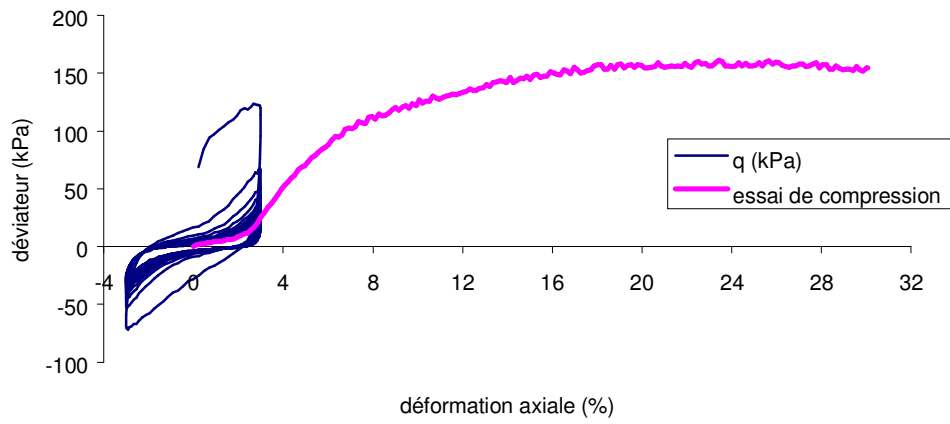
Evolution de la pression intersticielle limon CNR 6v2 - w_c = 19,7\% , s'_{vo} = 100 kPa
