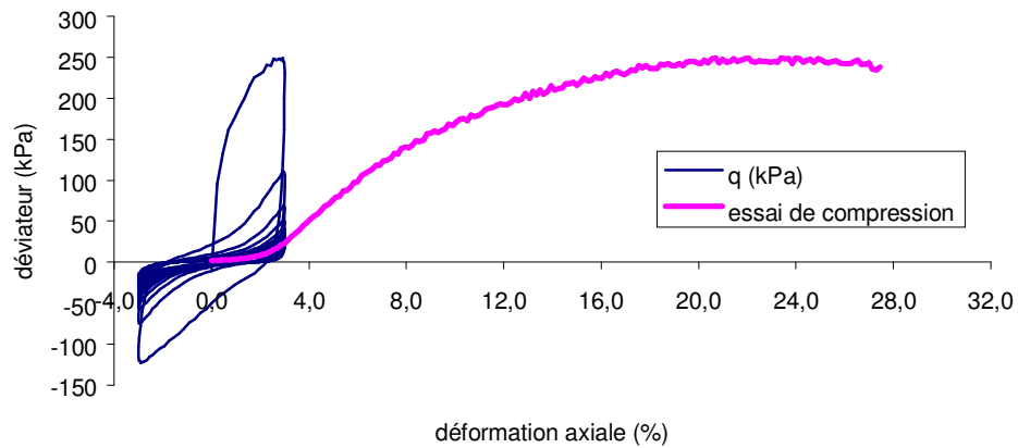
Evolution de la pression intersticielle limon ' A' 3v2 - wc = 21,5%, s' vo = 200 kl
