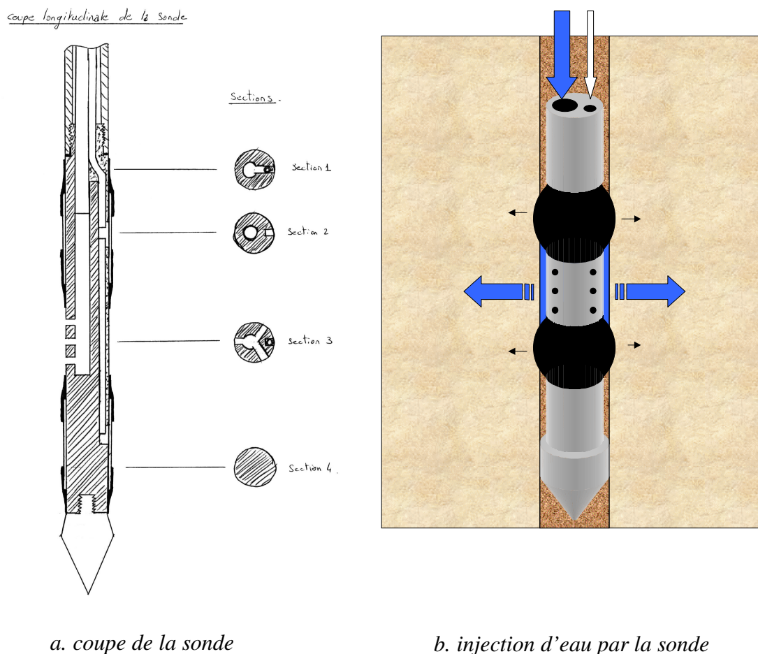
figure 2-5, Schéma de principe de la sonde de perméabilité
