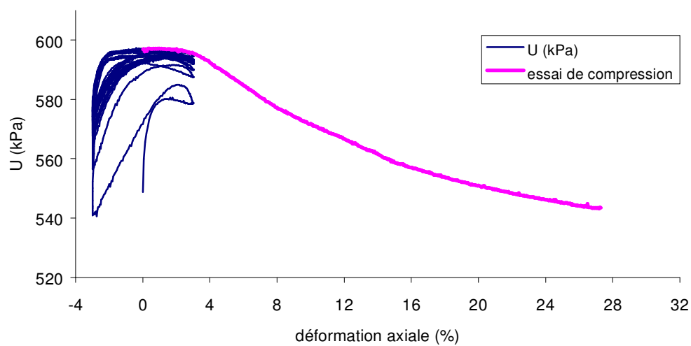
Chemin de contraintes limon ' A' Ila2 - wc = 19,0%, s' vo = 50 kl
