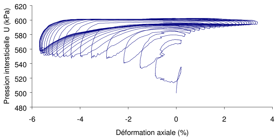
Evolution de la pression interstitielle - Limon ' A' Li CSF wc = 17,8 %, s' vo = 100 kPa - Cycles à CSR = 0,25
