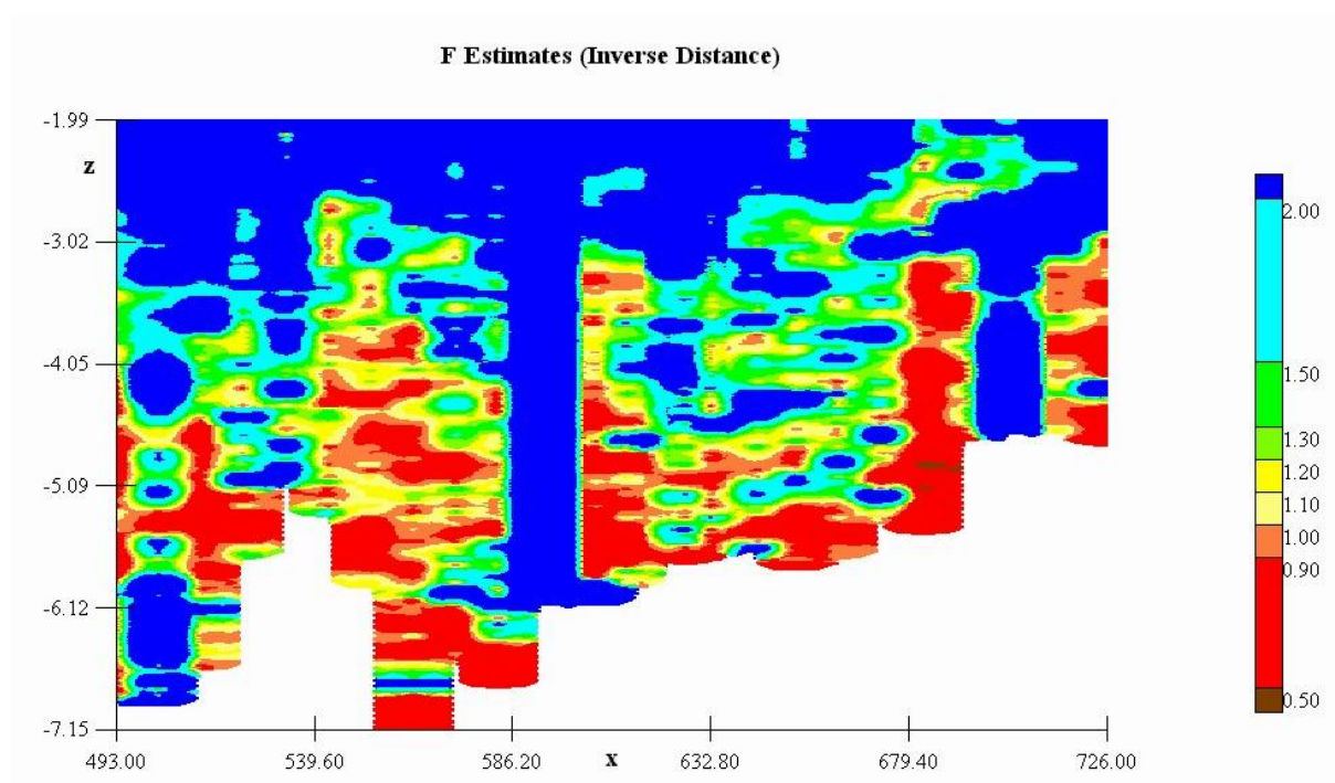
figure 3-26, carte des coefficients de sécurité
