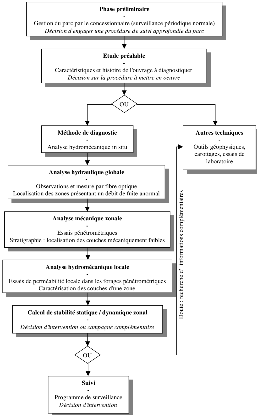
figure 1-24, méthodologie
