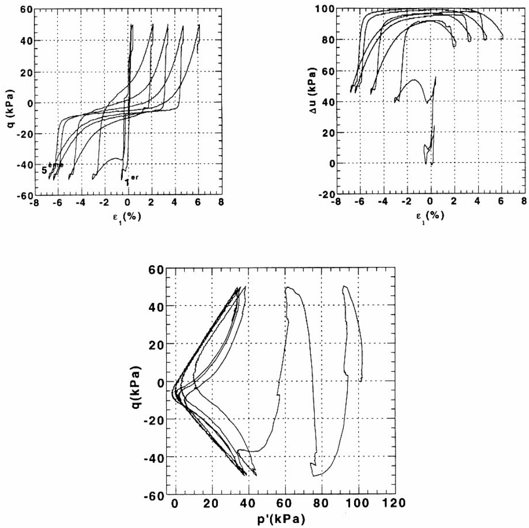
Essai cyclique non drainé sur le sable de Fontainebleau ( I_D = 0,53 , p'_c = 100 kPa, q_{am} = 50 kPa)
