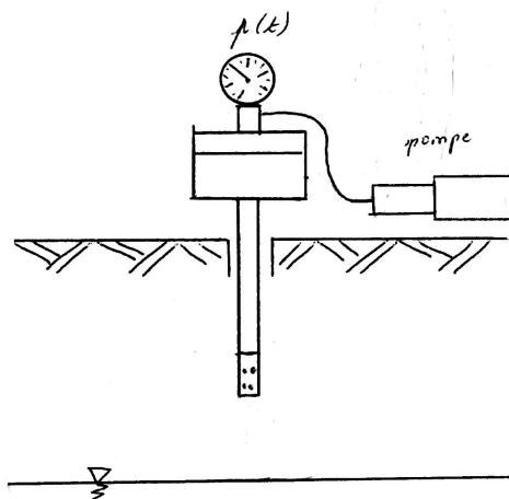
d. injection d'air à charge variable
