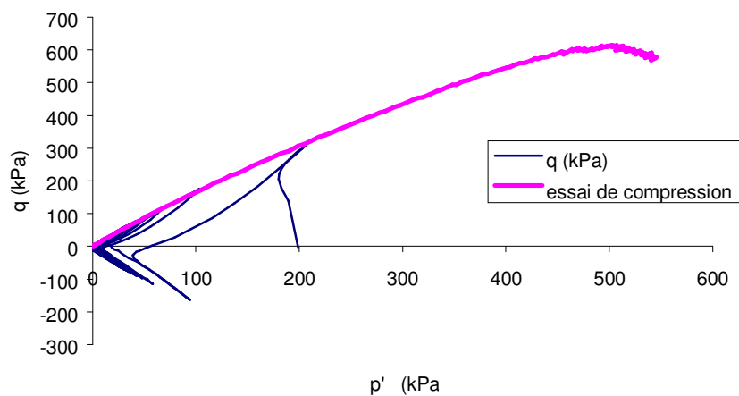
Chemin de contraintes limon ' A' - wc = 17,3% - s' vo = 200 k
