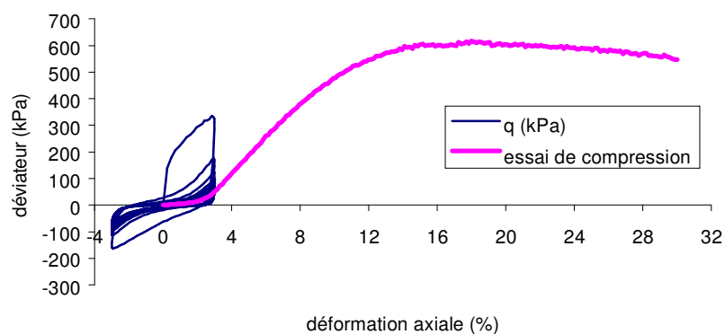
Evolution de la pression interstitielle limon ' A' 1v3 - wc = 17,3%, s' vo = 200kl
