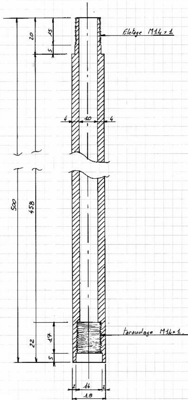
figure D-6, plan d'un tige
