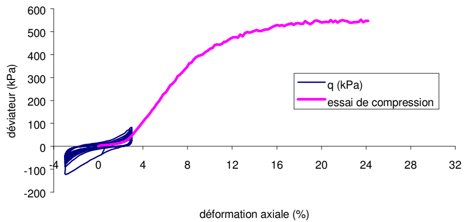
Evolution de la pression interstitielle limon ' A' 5v2 - wc = 17,5%, s' vo = 100 kl
