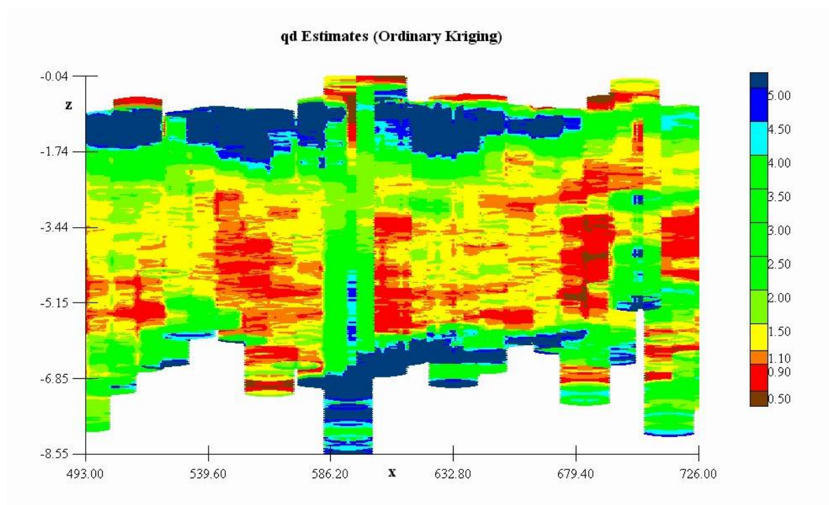
figure 2-31, carte krigée des résistances de pointe
