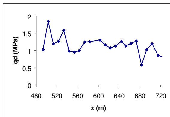
b. limon de fondation
