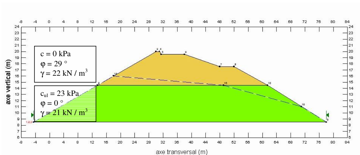
figure 3-37, modèle de section caractéristique post-sismique (critère C_2 )
