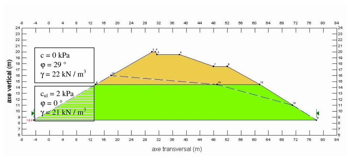
figure 3-36, modèle de section caractéristique post-sismique (critère C_1 )
