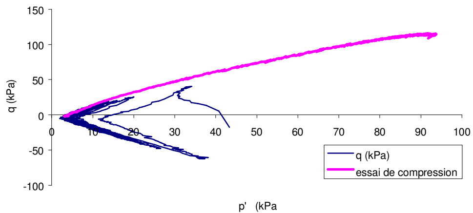
Chemin de contraintes limon ' A' Ila2 - wc = 19,0%, s' vo = 50 kl
