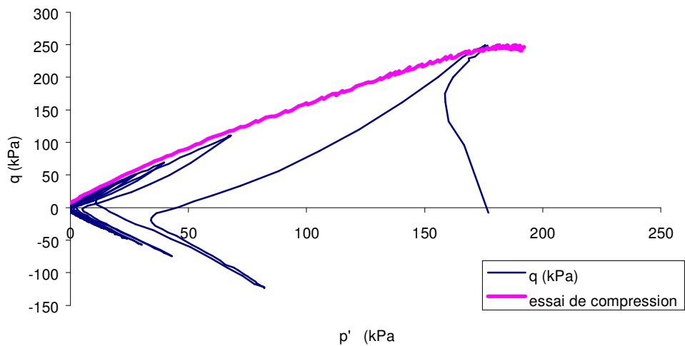
Chemin de contraintes limon ' A' 3v2 - wc = 21,5%, s' vo = 200 kl
