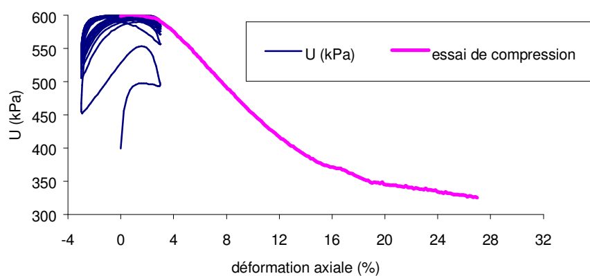
Chemin de contraintes limon ' A' - wc = 17,3% - s' vo = 200 k
