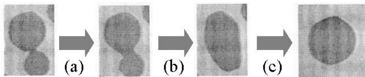
Figure IV-9 : Etapes de la coalescence de deux agrégats (vues planes) [ Rosenfeld1999 ], (a) les deux agrégats (sous leur forme d'équilibre) se rencontrent et une zone de contact se forme entre eux, (b) l'agrégat formé se relaxe pour évoluer vers une forme ellipsoïdale tronquée, (c) puis sphérique tronquée (forme d'équilibre).
