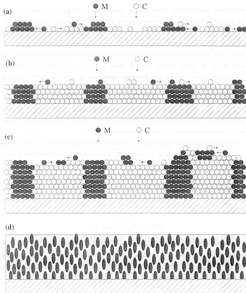
Figure III-3 : (a), (b), (c) Etapes du mécanisme de croissance probable pour la croissance d'un film nanocomposite métal-isolant par codépôt de l'espèce métallique (M) et diélectrique (sur ce schéma, le carbone, C), et (d) structure finale d'un tel matériau [Babonneau].
