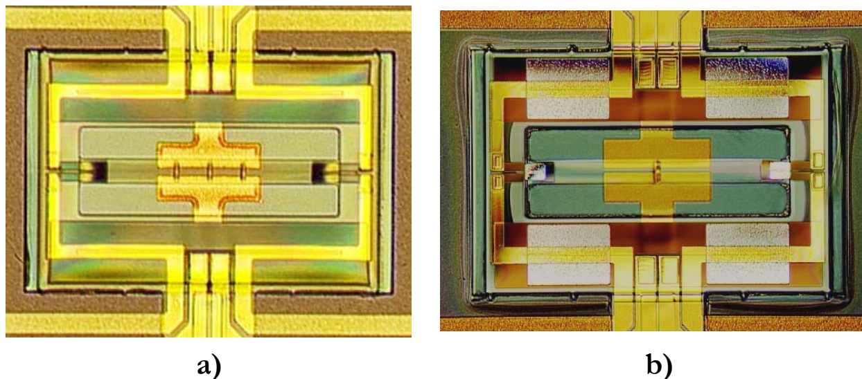
Figure 117 : prototypes fabriqués avec des actionneurs en a) inconel et b) aluminium
