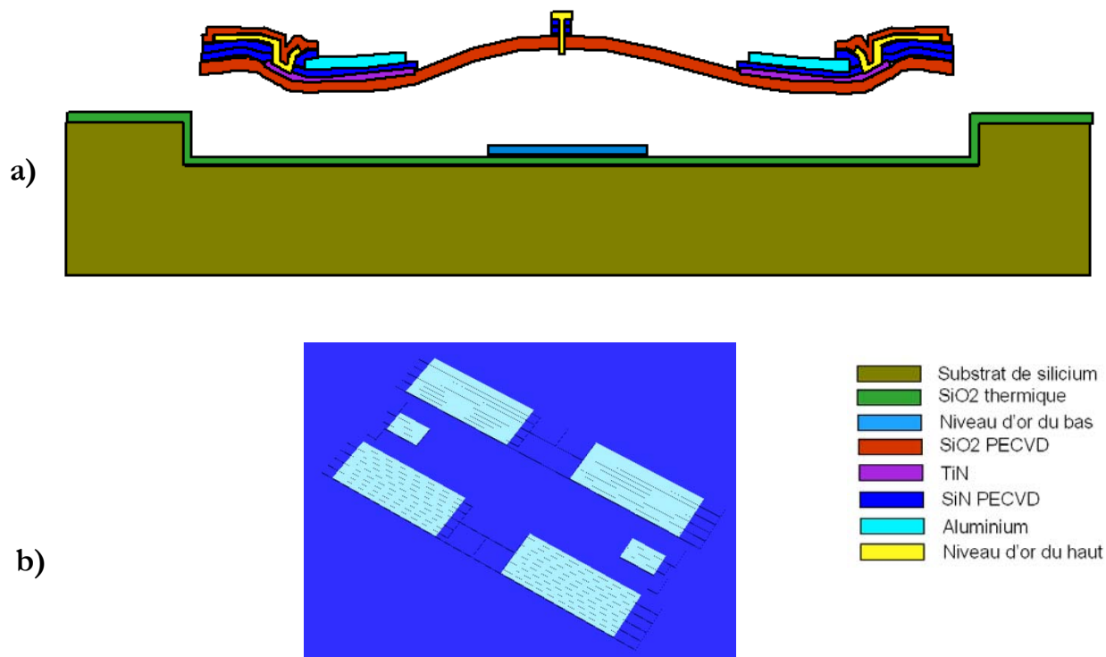
Figure 116 : a) prototypes avec actionneurs en aluminium en coupe le long de la poutre, et b) masque supplémentaire nécessaire pour la gravure de l'aluminium
