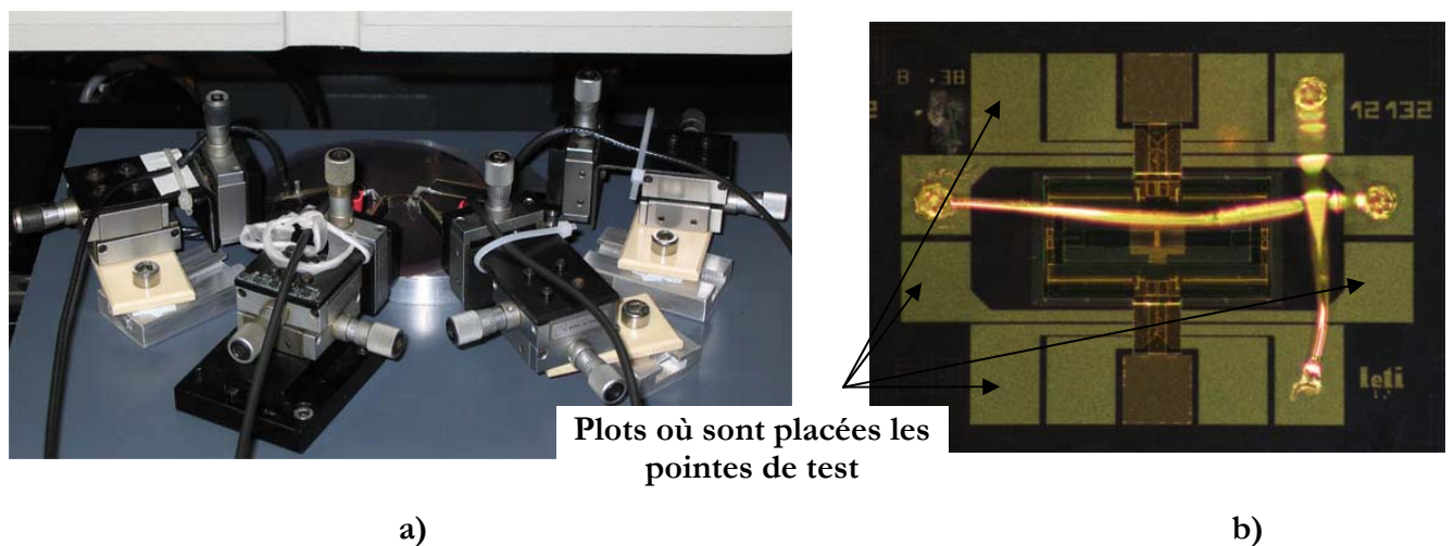
Figure 111 : a) 4 pointes pour test sous WYKO, et b) wire bonding associé à ce test
