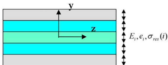
Figure 65 : stratifié miroir
