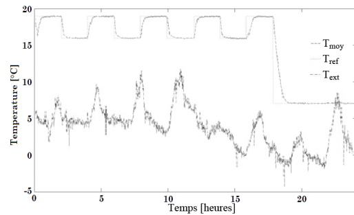
Figure 2.34 – Température régulée par PID-flou (configuration E')
