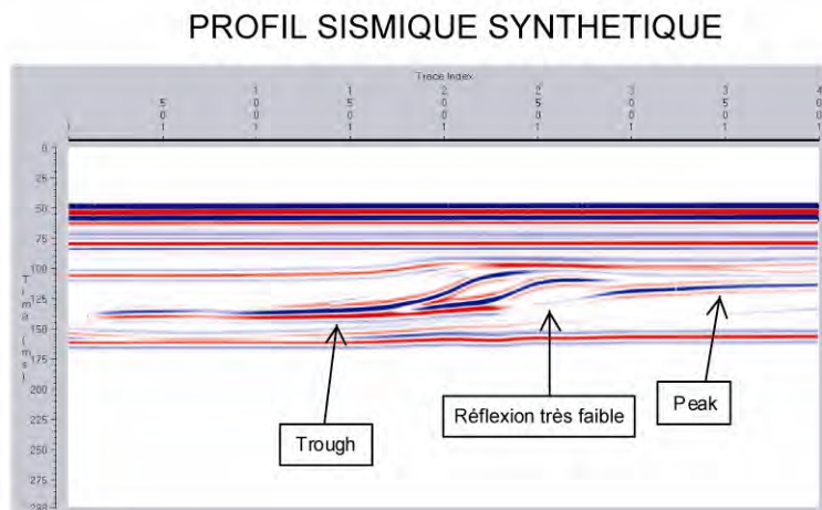
Figure IV-5 : Les réflexions sismiques : indicateurs chronostratigraphiques et lithostratigraphiques. A) Les réflexions sismiques sont générées par les variations de faciès brutales entre les strates (lignes temps). Les variations latérales de faciès au sein des strates ne génèrent pas de réflexion sismique du fait de leur caractère graduel. (D'après Homewood et al. , 2000) B) Modèle sismique d'un système progradant dont chaque corps est caractérisé par des variations latérales progressives de faciès. L'étude des variations d'amplitude et autres attributs le long des réflexions sismiques renseigne sur les variations lithostratigraphiques de part et d'autre des clinoformes.
