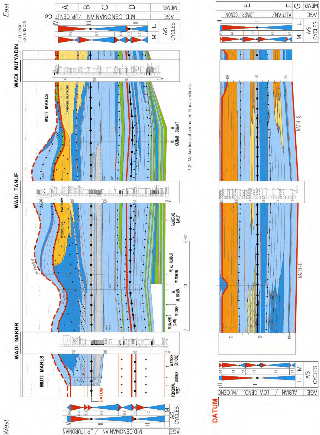
Figure III-16 : Modèle de stratigraphie séquentielle haute-résolution du transect du Jebel Akhdar (van Buchem et al. , 2002).
